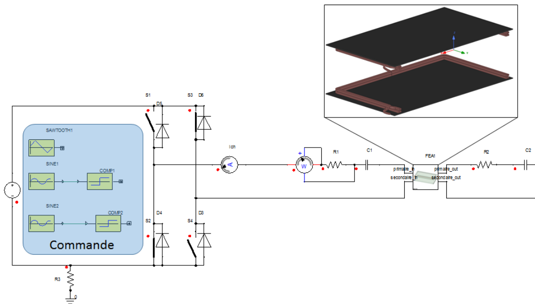
Figure II.46 – Modèle de co-simulation symétrique utilisé.
