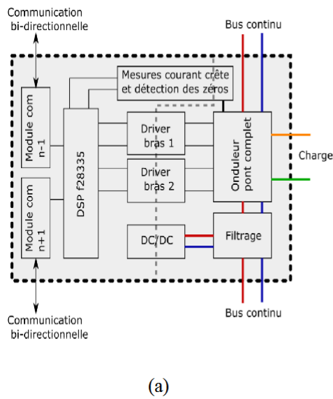
Figure II.22 – L'onduleur utilisé, synoptique de l'onduleur (a), photo de l'onduleur (b).
