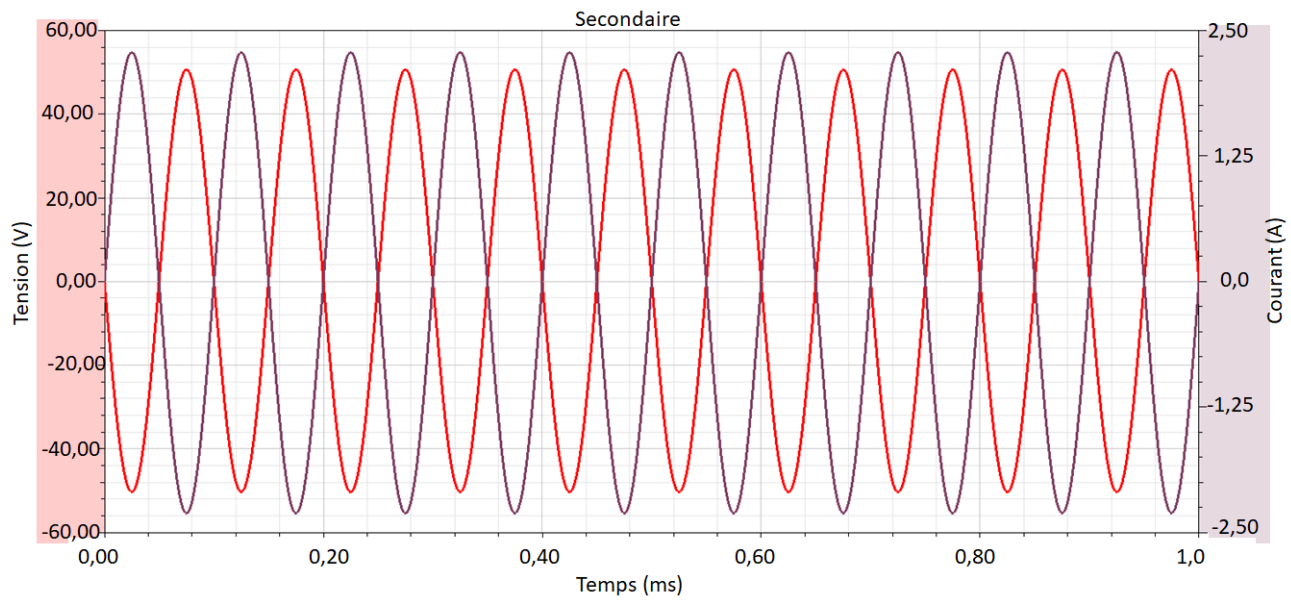
Figure II.20 – Courant et tension du secondaire.
