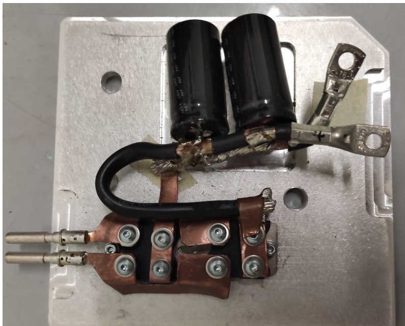
Figure IV.12 – Redresseur utilisé dans le banc d'essai.
