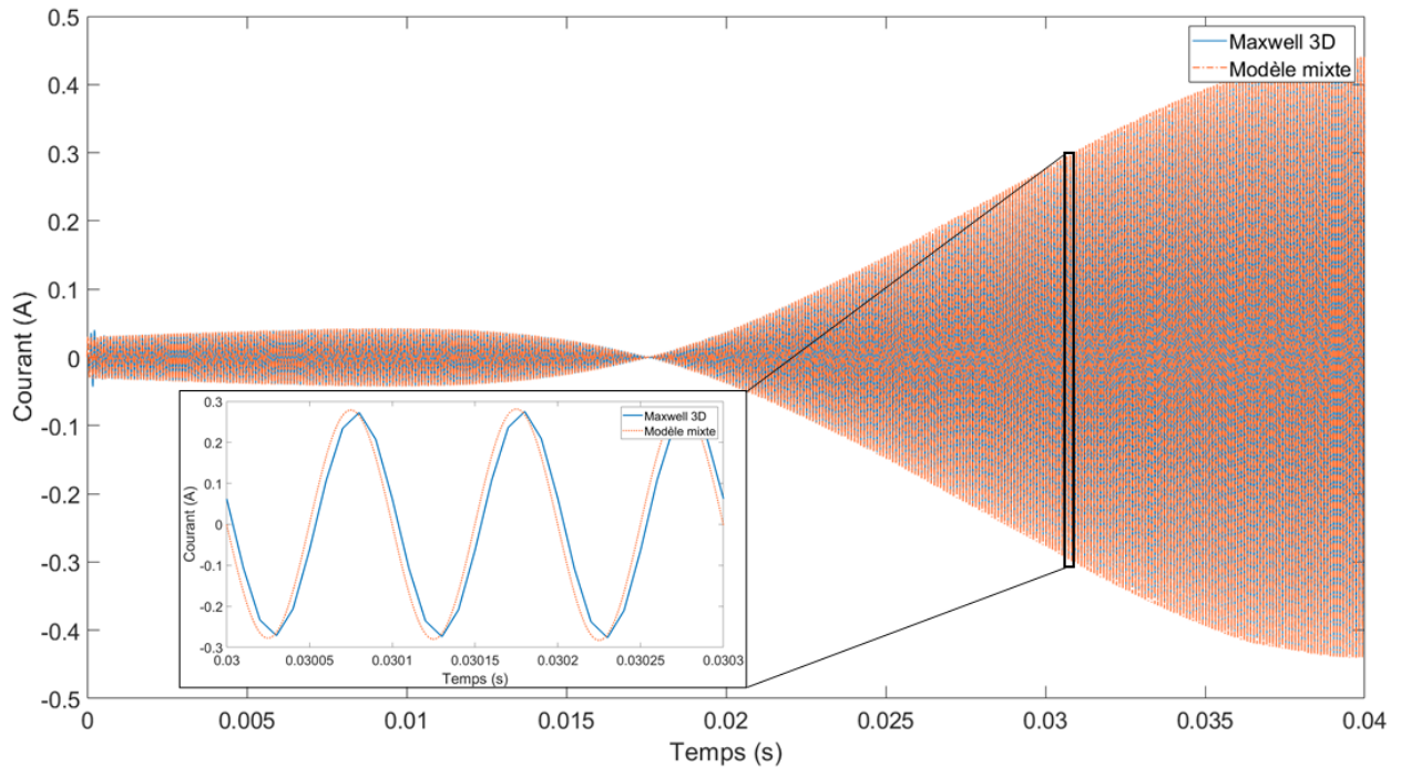
Figure III.8 – Comparaison des courants induits obtenus avec le modèle mixte et le solveur temporel.
