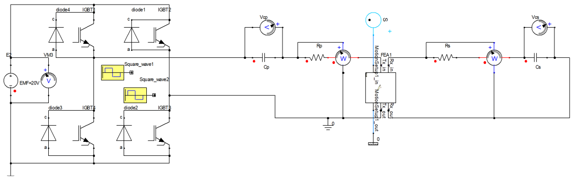
Figure III.16 – Circuit électrique associé.
