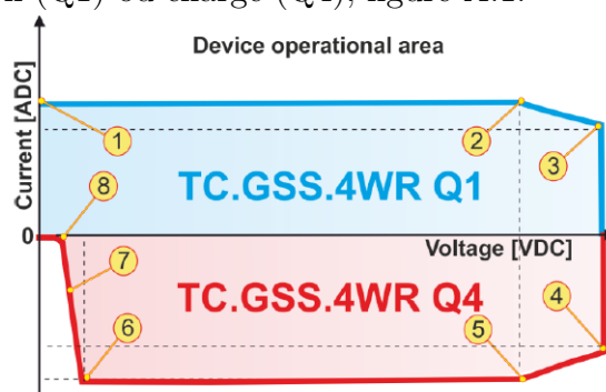
Figure A.1 – Cadrants de fonctionnement du Regatron .
