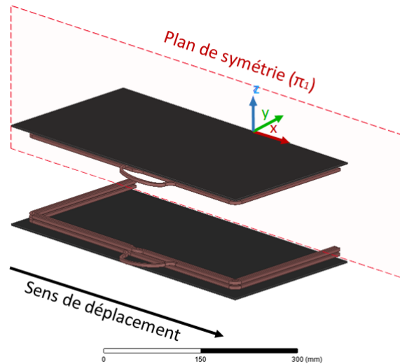
Figure II.45 – Modèle de coupleur avec un seul plan de symétrie considéré.
