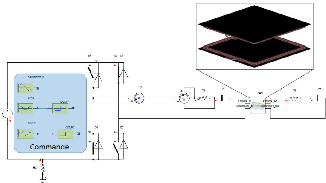
Figure II.23 – Modèle électrique d'onduleur connecté aux bobines en position vis-à-vis.
