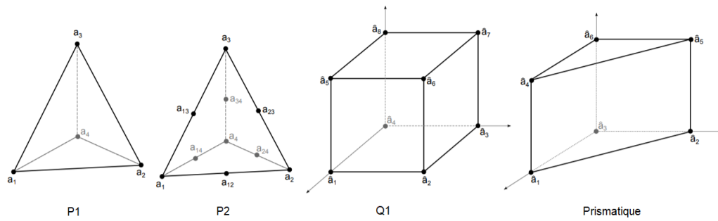
Figure B.2 – Éléments finis tridimensionnels de Lagrange : tétraédriques P1 et P2, parallélépipédique Q1 et prismatique [84].
