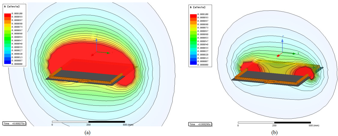
Figure II.17 – Induction magnétique dans le plan ZY à t = \frac{3T}{4} (a) et à t = \frac{19T}{20} (b).
