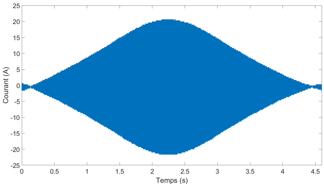
Figure IV.31 – Évolution du courant mesuré dans la bobine secondaire.
