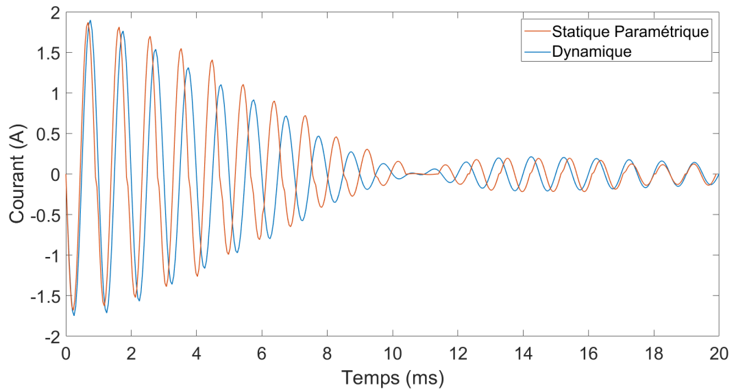
Figure C.2 – Comparaison entre le courant induit obtenus par les deux méthodes.
