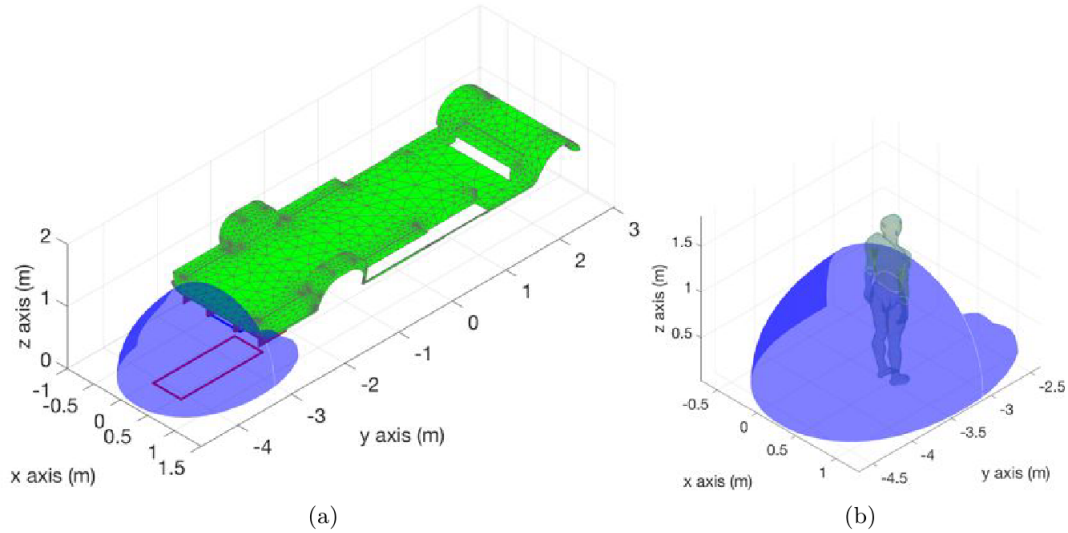
Figure I.27 – Simulation du champ magnétique généré dans une région d'espace au-dessus de la bobine primaire (scénario pire cas), (a) en absence de mannequin, (b) en présence de mannequin [66].
