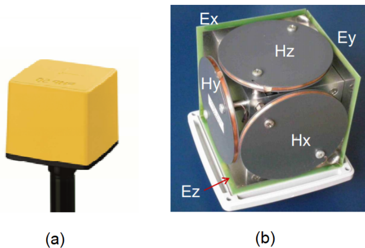
Figure IV.20 – Sonde Narda utilisée.
