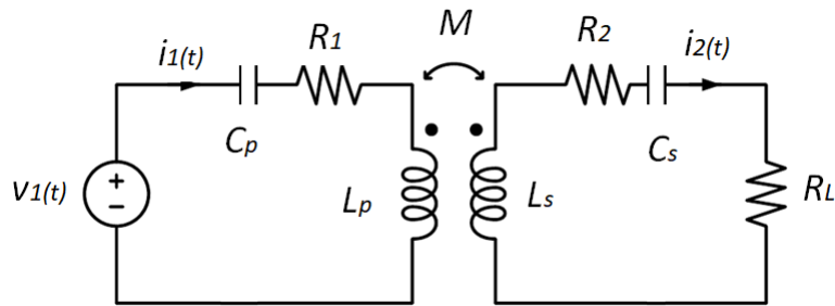
Figure IV.4 – Circuit électrique équivalent du système de charge dynamique sans contact réalisé.
