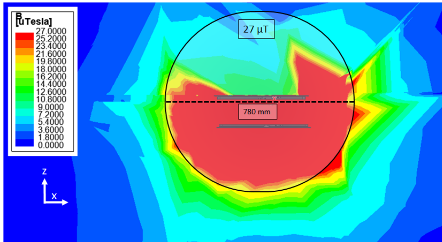
Figure IV.46 – Périmètre de sécurité autour du coupleur en coupe transversale en position vis-à-vis pour un seuil de 27 \mu T .
