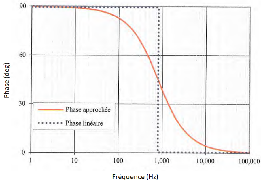
Figure II.59 – Phase de référence des champs en fonction de la fréquence.
