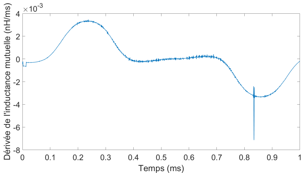
Figure III.13 – Variation de la dérivée de l'inductance mutuelle.
