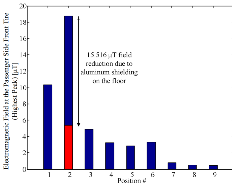
Figure I.25 – Impact de la plaque d'aluminium sur le champ magnétique généré par les deux bobines [56].
