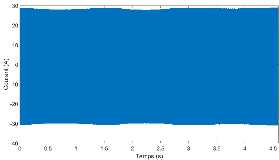
Figure IV.34 – Évolution du courant mesuré dans la bobine primaire.
