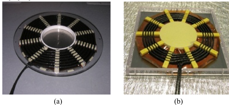
Figure I.19 – Système "ORNL" de recharge sans contact, bobine du primaire (a) et bobine du secondaire (b) [56].
