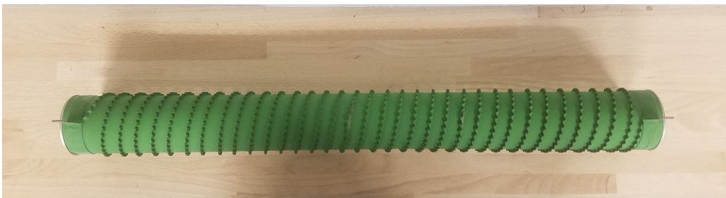
Figure IV.9 – Résistance de 1 \Omega à connecter au primaire et au secondaire.
