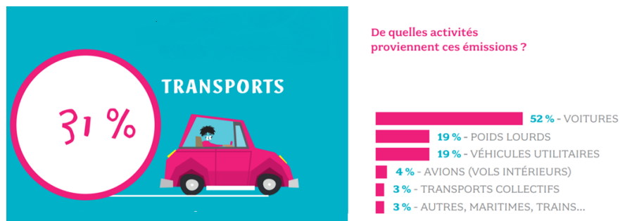
Figure 2 – Participation du domaine de transport dans les émissions de gaz à effet de serre en France en 2019. Source : Haut conseil pour le climat.
