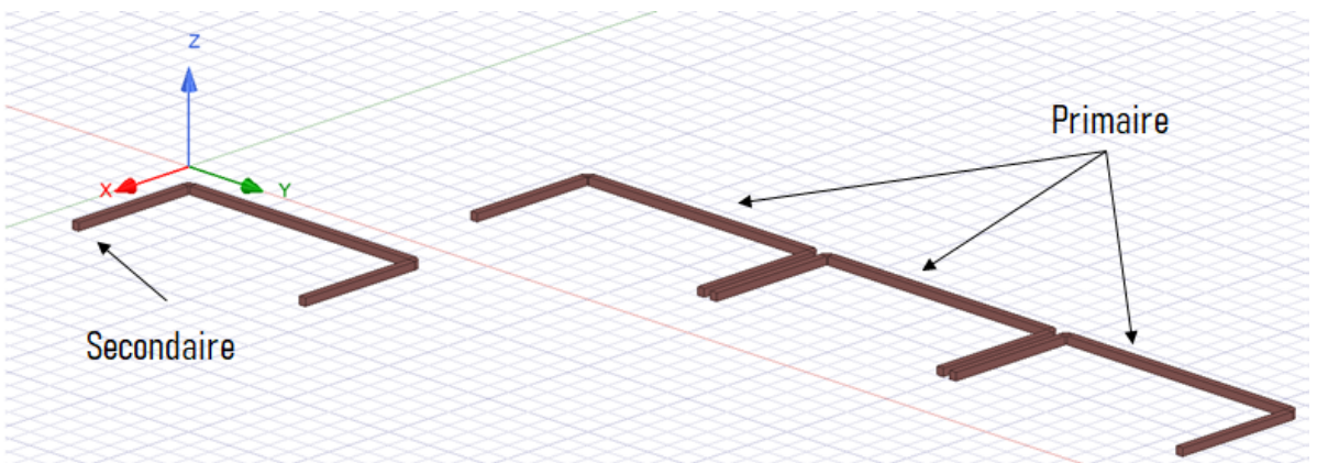
Figure III.10 – Disposition des bobines dans le modèle trois bobines au primaire.
