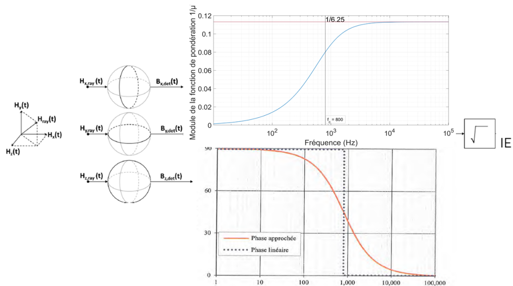
Figure II.60 – Synoptique d'une sonde de mesure pondérée.
