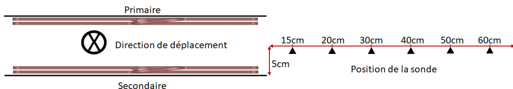
Figure IV.36 – Positions de la sonde pour mesurer l'induction magnétique.
