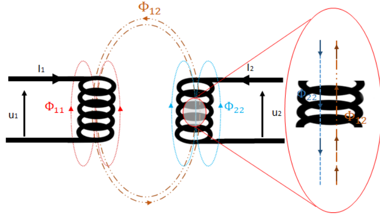
Figure III.2 – Répartition des flux magnétiques autour des bobinages primaire et secondaire.
