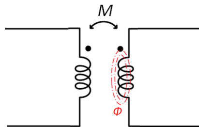
Figure I.8 – Schéma du couplage magnétique.
