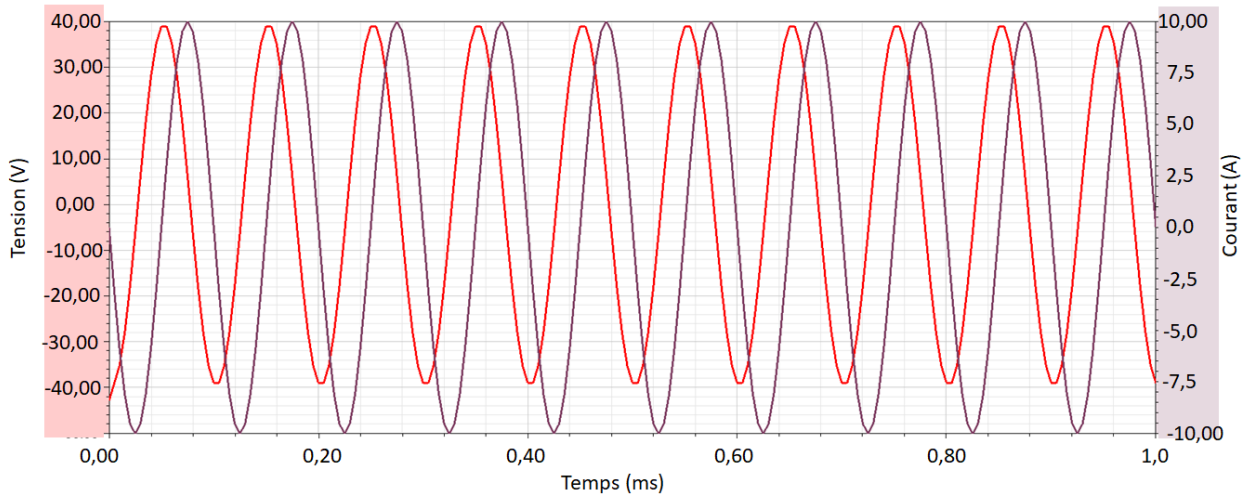
Figure II.16 – Courant et tension de la bobine excitée par un courant sinusoïdal d'amplitude 10 A et de fréquence 10 kHz.
