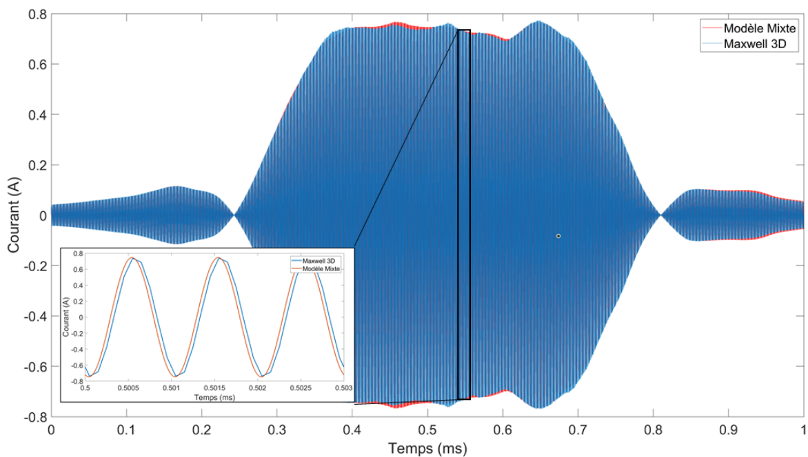
Figure III.15 – Comparaison du courant induit obtenu avec le modèle Maxwell 3D amélioré et le modèle mixte.
