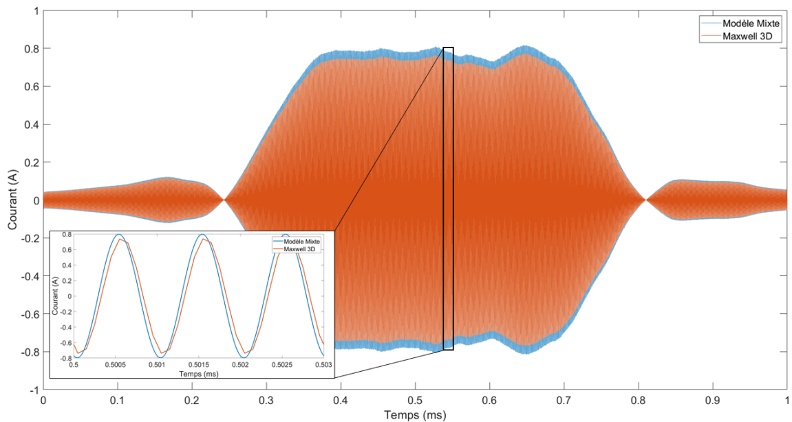
Figure III.14 – Comparaison du courant induit obtenu avec le modèle Maxwell 3D et le modèle mixte.
