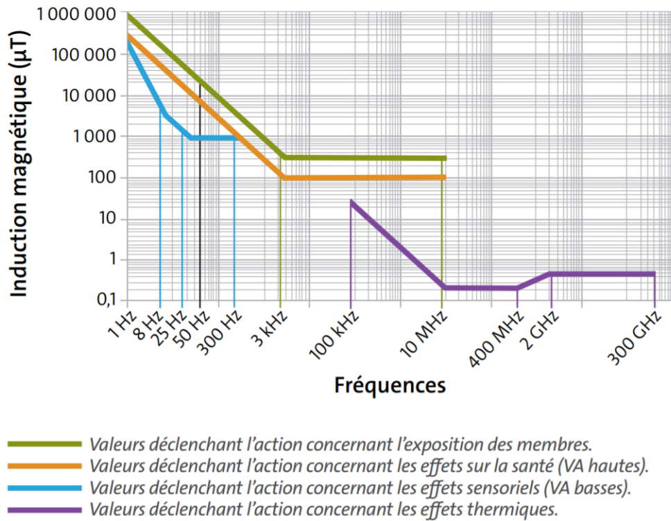
Figure D.5 – Valeurs d’action pour les champs magnétiques, [89], selon la directive 2013/35/UE.
