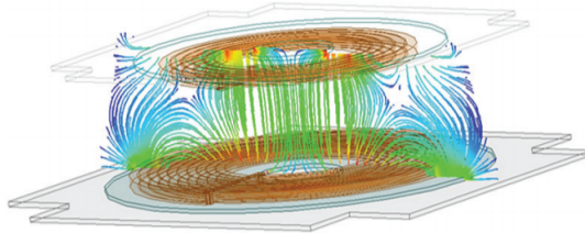
Figure B.3 – Exemple de coupleur simulé sous Maxwell 3D.
