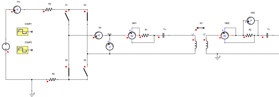
Figure IV.5 – Circuit électrique du système de charge sans contact.
