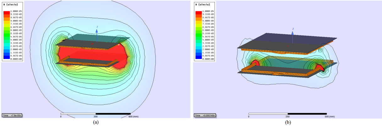
Figure II.21 – Champ magnétique dans le plan ZY à t = \frac{3T}{4} (a) et à t = \frac{T}{2} (b).
