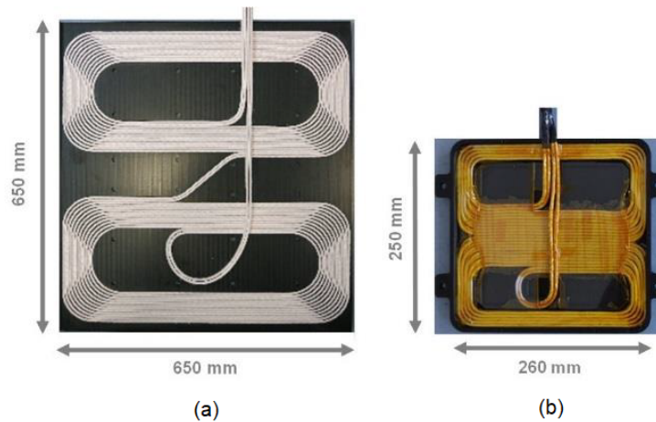
Figure II.2 – Exemple de modèles de bobines utilisées dans un système de recharge sans contact, (a) émettrice (primaire), (b) réceptrice (secondaire) [76].
