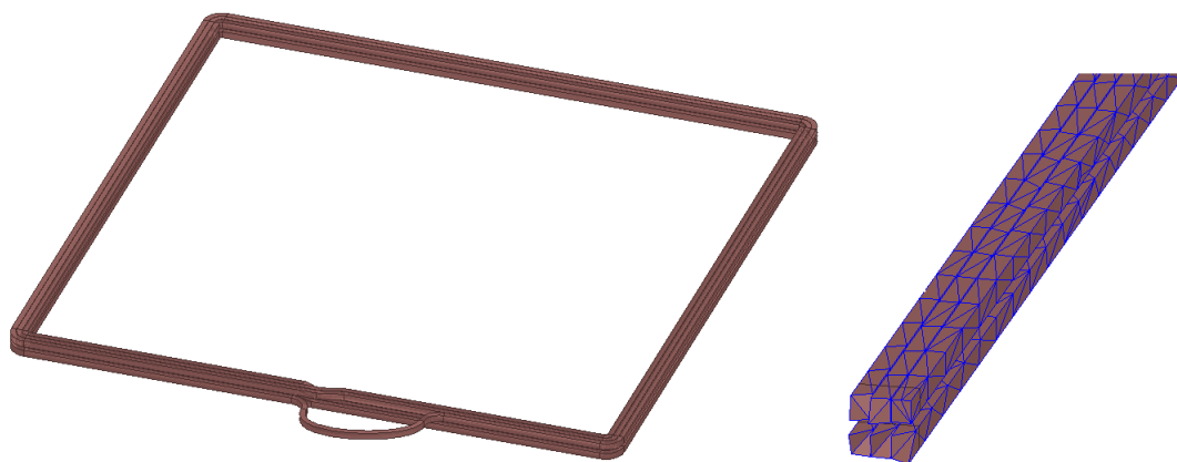
Figure B.1 – Exemple d'une bobine et d'une partie de son maillage.
