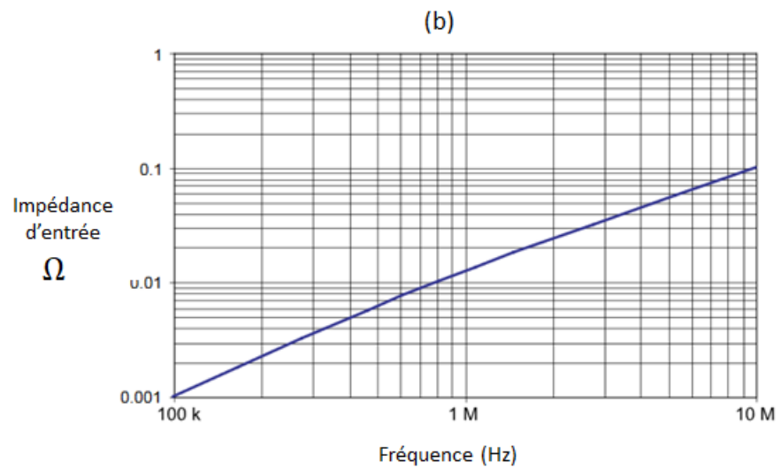
Figure A.3 – Caractéristique de courant (a) et d'impédance d'entrée (b) en fonction de la fréquence.
