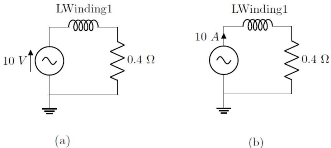
Figure II.15 – Modèle d'alimentation réalisé sous "MaxwellCircuit" connecté à la bobine, source de tension (a), source de courant (b).
