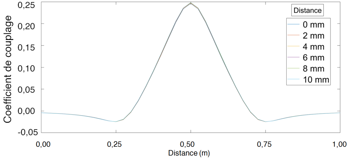
Figure II.9 – Impact de la distance bobine-ferrite sur le coefficient de couplage.
