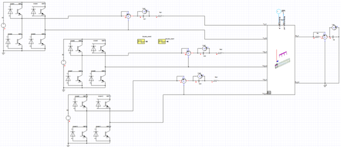
Figure III.9 – Circuit associé au modèle trois bobines au primaire.
