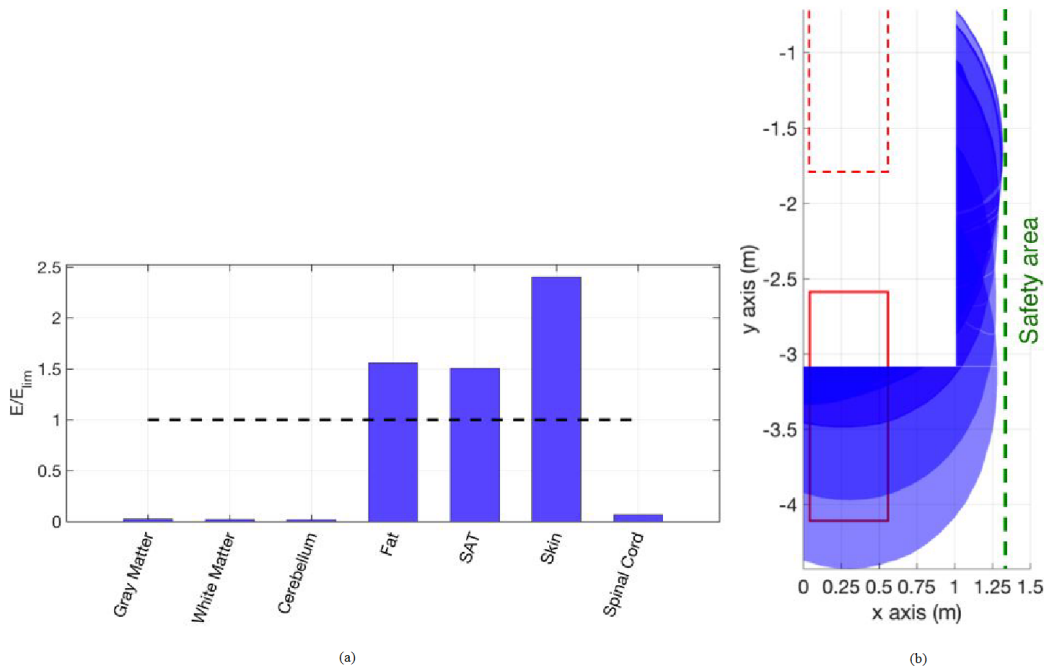
Figure I.28 – (a) indice d'exposition de différentes parties du corps, (b) périmètre de sécurité autour du véhicule selon les recommandations de l'ICNIRP 1998 [66].
