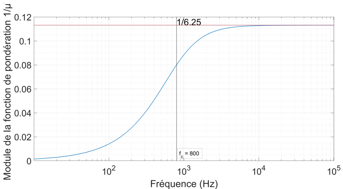
Figure II.58 – Filtre de pondération de la MCP.
