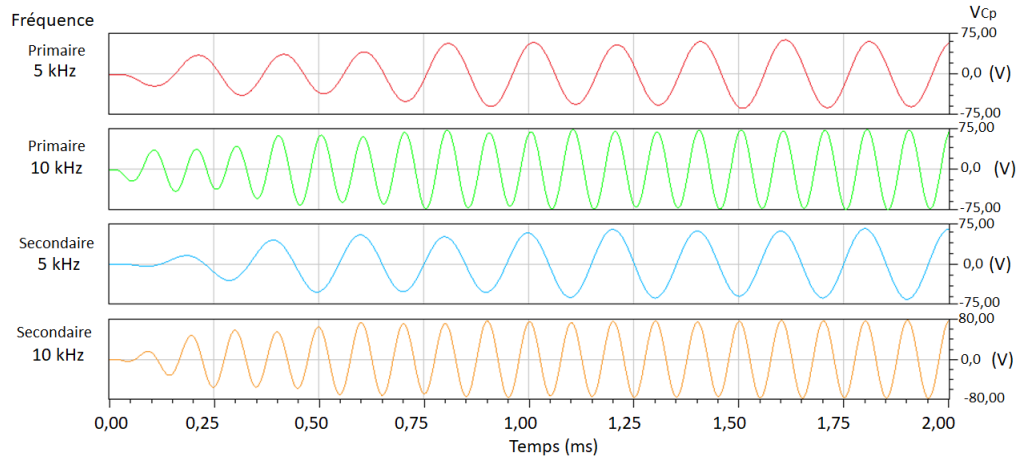
Figure II.26 – Tensions aux bornes des condensateurs primaire et secondaire aux fréquences 5\text{ kHz} et 10\text{ kHz} .
