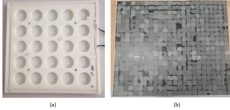
Figure IV.3 – La bobine (a) et la plaque de ferrite (b) utilisées.
