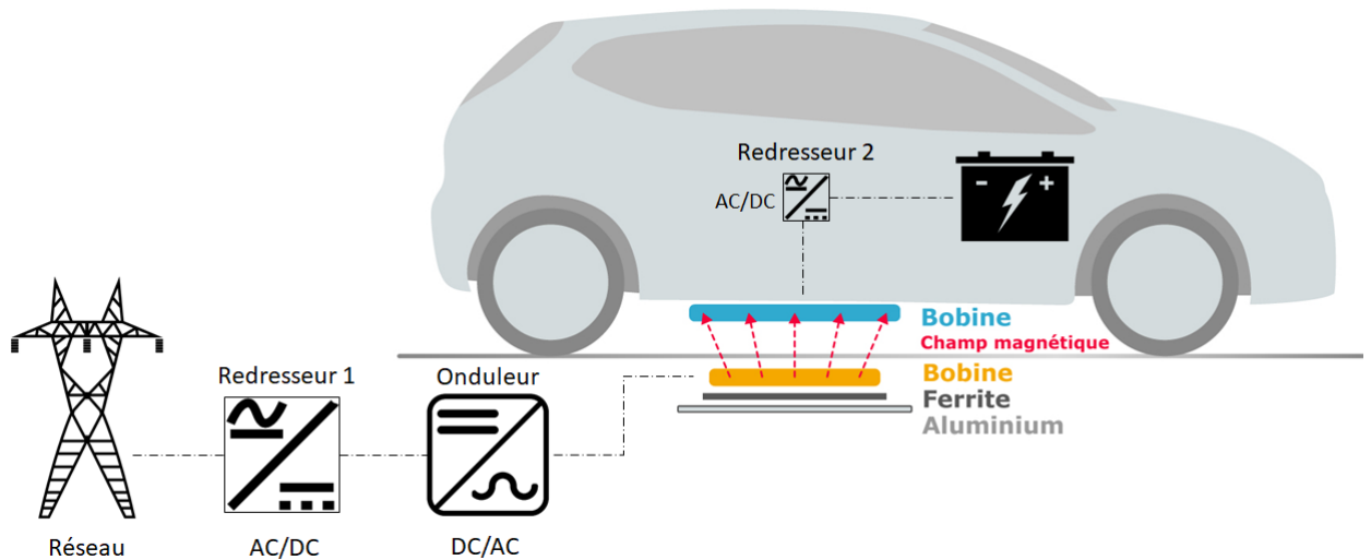
Figure I.7 – Schéma global d'un système de recharge sans contact.
