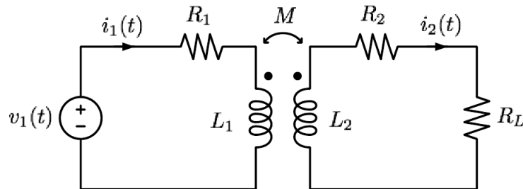
Figure I.15 – Modèle électrique équivalent au système de charge sans contact.
