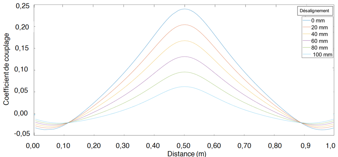
Figure II.10 – Impact du désalignement sur le coefficient de couplage.
