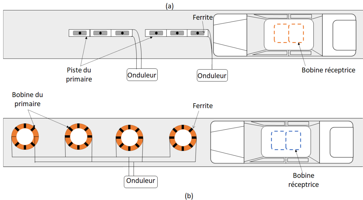
Figure I.9 – Illustration des deux types de pistes de recharge, (a) piste à émetteur unique (b) piste à émetteurs segmentés.
