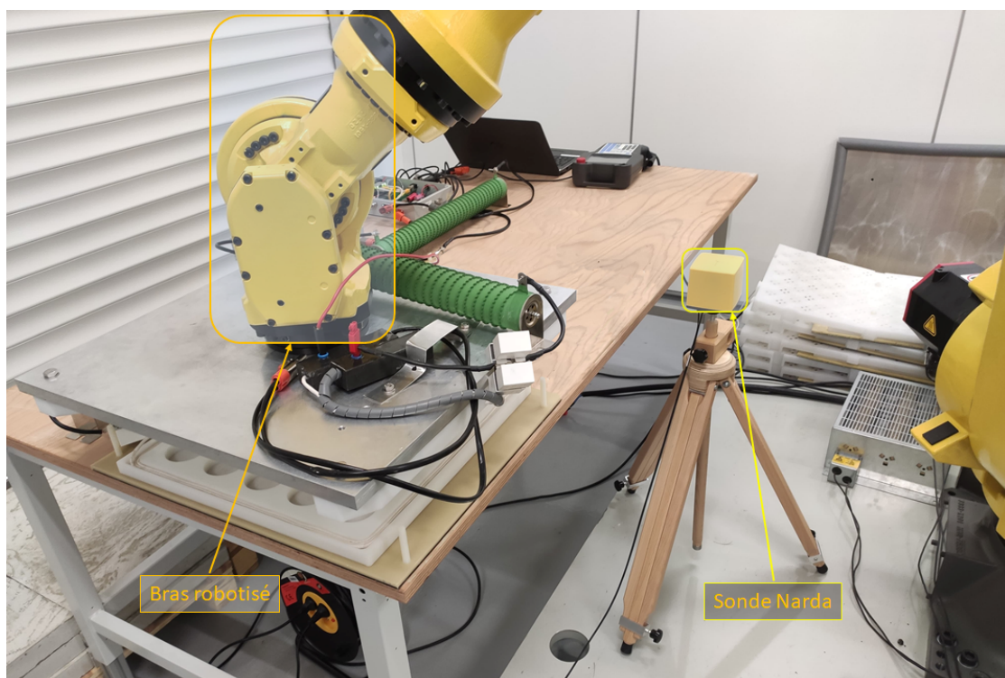
Figure IV.43 – Environnement de mesure de l'induction magnétique.
