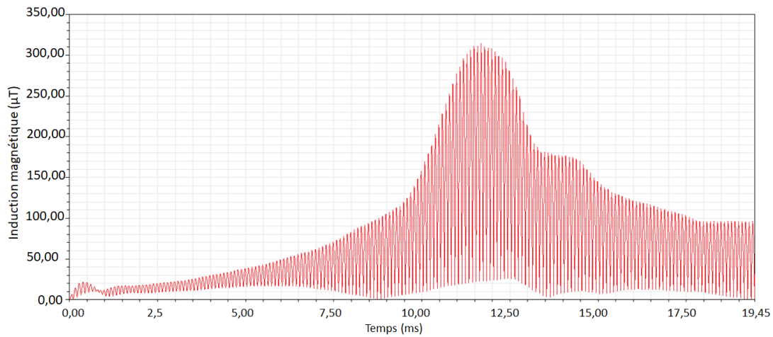
Figure II.38 – Induction magnétique évaluée à 230 mm au-dessus du primaire.
