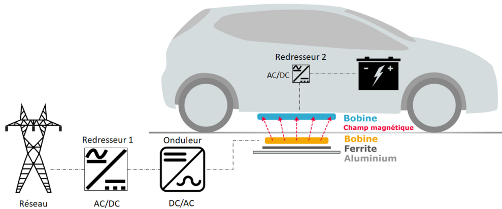
Figure 3 – Système de transfert d'énergie sans contact.
