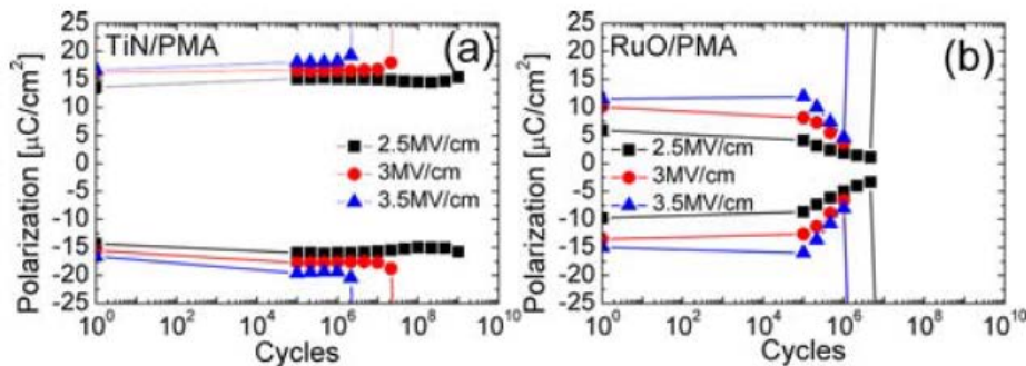
FIGURE IV.32 – (a) Tests d'endurance d'un échantillon TiN/HZO/TiN pour différentes tensions (b) (a) Tests d'endurance d'un échantillon TiN/HZO/RuO(TE) pour différentes tensions. [250]
