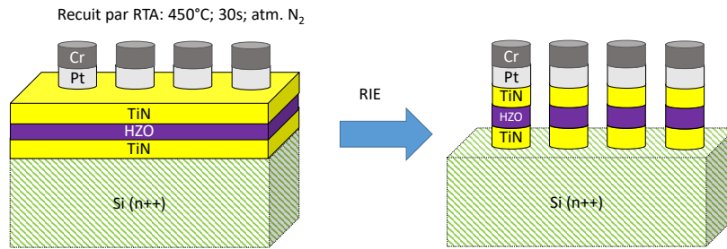
FIGURE VI.18 – Architecture de l'échantillon réalisé par gravure RIE.
