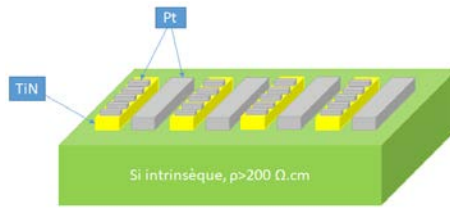
FIGURE III.41 – Schéma de la structure pour l'échantillon de Si/TiN/Pt avec des TLM de Pt dédiés aux mesures de résistivité par la méthode 4 points en configuration Van der Pauw
