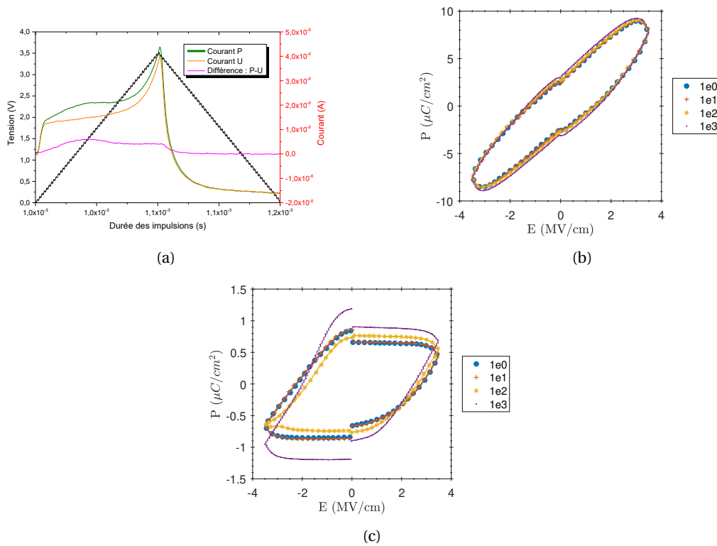
FIGURE V.25 – (a) Réponse des courants P (vert), U (orange) et P-U (magenta) au signal de tension positif en noir après 10^3 cycles. (b) Courbes d’hystérésis P(E) obtenues à partir des signaux P et N pour l’échantillon Pt(évap). (c) Courbes d’hystérésis P(E) obtenues à partir des signaux P-U et N-D pour l’échantillon Pt(évap).
