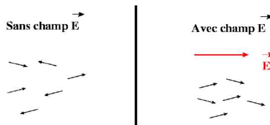
FIGURE I.4 – Répartition des moments dipolaires dans un ensemble de molécules polaires à gauche en l'absence de champ et à droite avec un champ extérieur appliqué.
