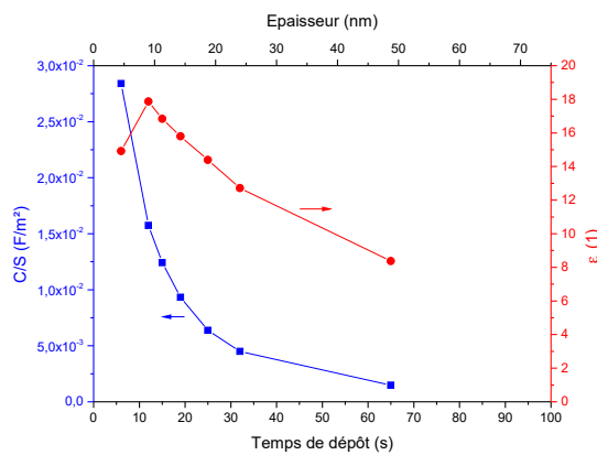
FIGURE V.38 – En bleu : capacité divisée par la surface du pad en fonction du temps de dépôt. En rouge : permittivité diélectrique du matériau en fonction de l'épaisseur. L'épaisseur indiquée sur le graphique est l'épaisseur moyenne estimée depuis la moyenne des vitesses de dépôts ( \frac{0,67+0,83}{2} = 0,75 nm/min).
