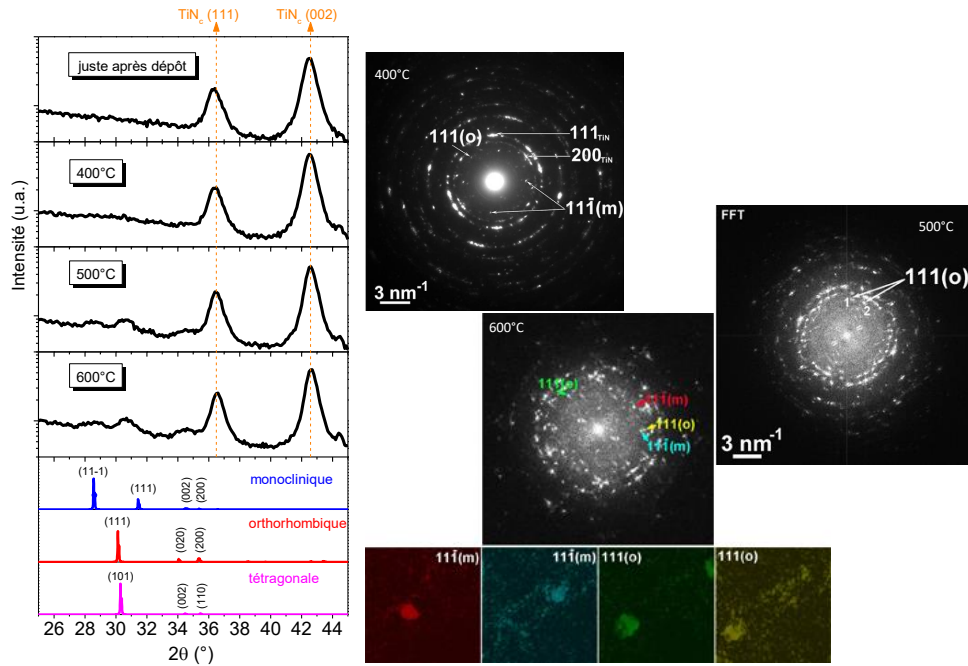
FIGURE V.9 – Identification des phases des échantillons Si/TiN/HZO/TiN déposé à 5 \times 10^{-2} mbar, non-recuit et recuits post-dépôt entre 400 °C et 600 °C. A gauche : diffractogrammes obtenus par GIXRD. A droite : motifs de diffraction issus des images HRTEM et SAED.
