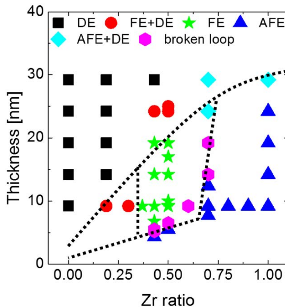
FIGURE IV.21 – Comportement de films de \text{Hf}_{1-x}\text{Zr}_x\text{O}_2 réalisés par ALD et déposés et recuits entre deux électrodes de TiN en fonction de l'épaisseur et de x . [161]
