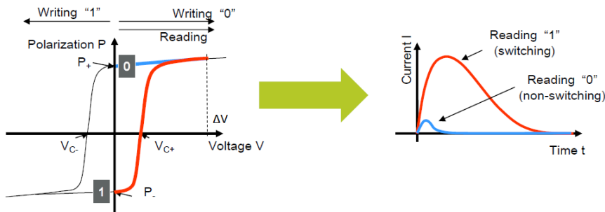
FIGURE I.29 – Description du fonctionnement d'une FRAM. [18]
