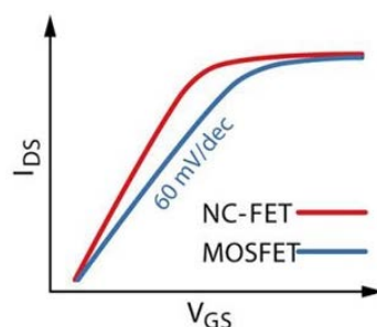
FIGURE I.36 – Caractéristiques I_{DS}(V_G) d'un transistor NC-FET. [27]
