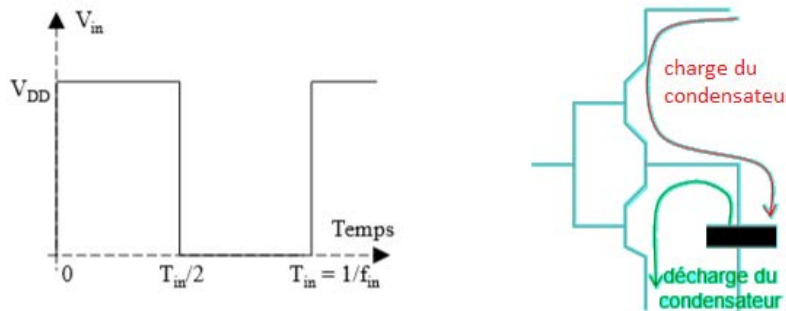
FIGURE I.16 – Paramètres permettant de calculer la puissance dissipée en dynamique. [4]
