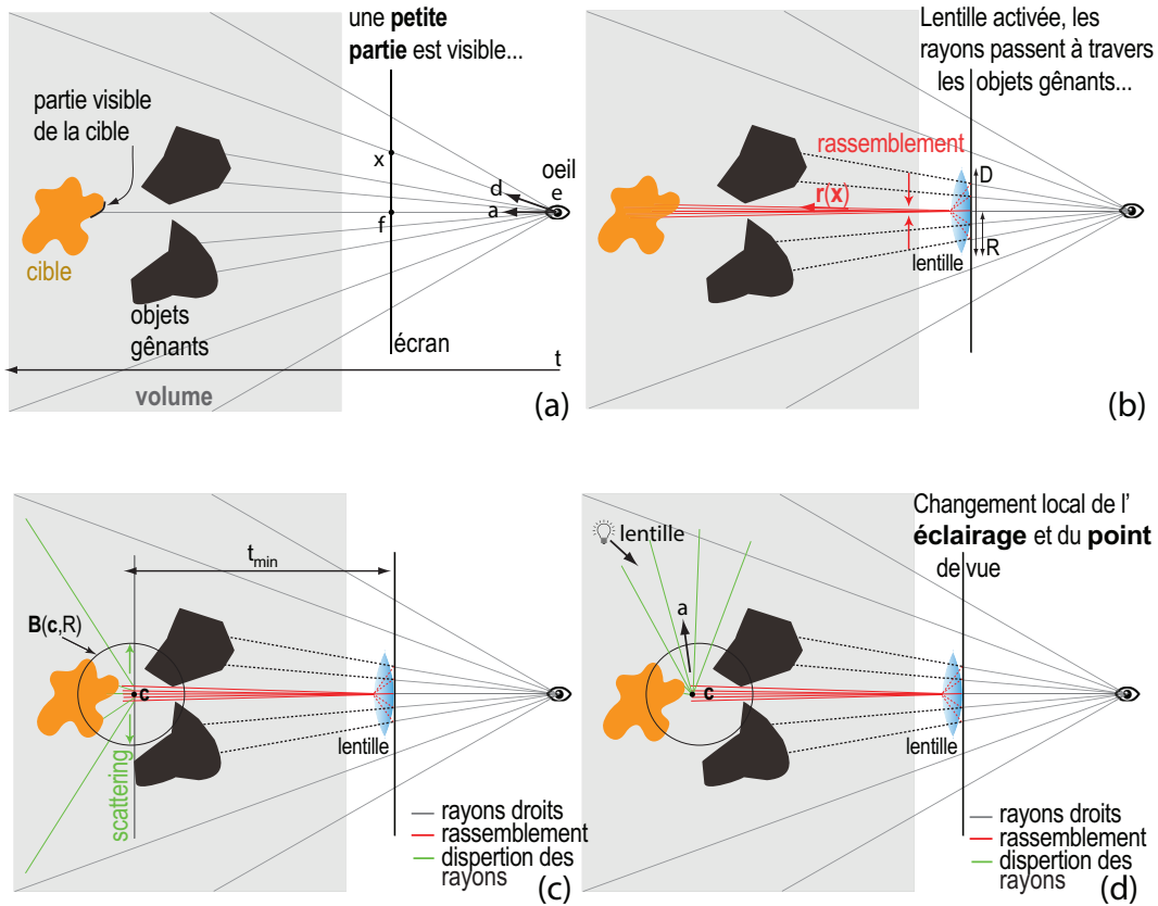
FIGURE 4.1: Fonctionnement de la lentille sans occlusion. Une cible est (principalement) cachée par des objets gênants devant elle. (a) Le DVR classique affiche une petite partie de la cible. (b) Notre lentille recueille des rayons pour éviter les objets gênants. Une fois près de la cible, les rayons suivent à nouveau leurs trajectoires initiales. Cependant, seule une petite partie de la cible est visible. (c) Les rayons se dispersent et rendent toute la cible visible. Enfin, nous ajustons les directions de visualisation et d'éclairage locales a, l^{lens} .
