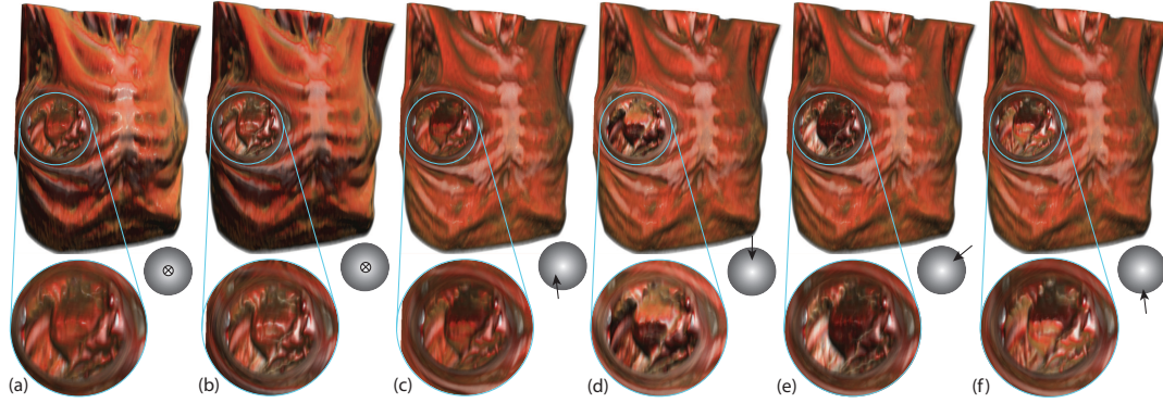
FIGURE 4.2: Modification des paramètres d'éclairage dans la lentille. (a) Coefficient spéculaire global constant. (b) Coefficient spéculaire élevé dans la lentille et faible en dehors. (c-f) La modification du vecteur lumière à l'intérieur de la lentille produit l'effet d'une lampe de poche tournant autour de la cible. Les icônes de la balle illustrent la direction du vecteur de lumière locale.
