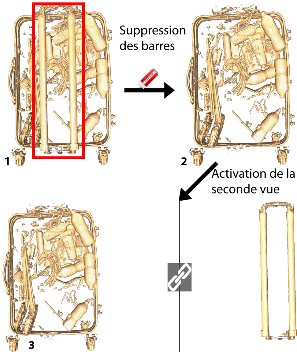
FIGURE 3.3: Résolution du problème d'occlusion en supprimant des objets d'une vue à une autre. 1- L'utilisateur veut retirer les barres du bagage. 2- Après un double clic avec l'outil de suppression, l'objet est supprimé de la vue principale. 3- Après l'activation de la 2ème vue, les objets retirés sont visibles à l'extérieur des bagages.
