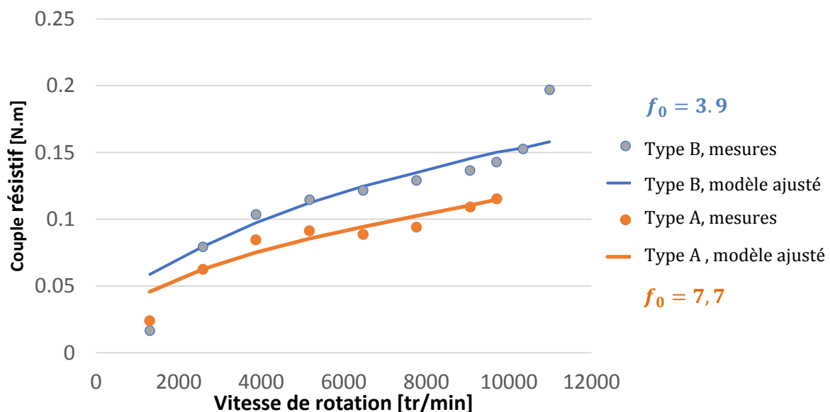
Figure 0.3 : Comparaison des modèles ajustés et des mesures de couple résistif pour les deux roulements testés.
