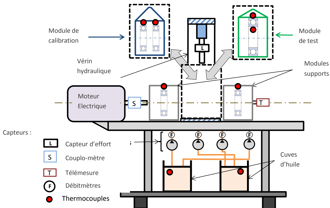
Figure 0.1 : Schéma du banc d'essai
