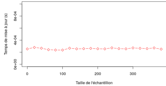
(b) Estimateur récursif f_n^{WW}
