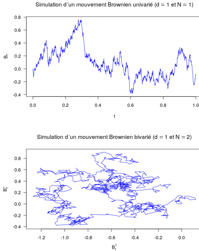
FIGURE 1.1. – Simulation d'un mouvement brownien univarié et bivarié
