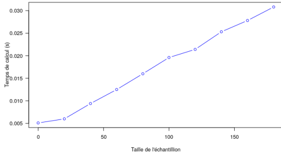
(a) Estimateur non-récursif f_n^{PR}
