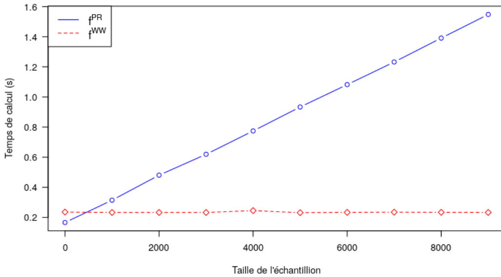
FIGURE 2.1. – Comparaison du temps de calcul pour des mises à jour par paquet de 1000 observations de l'estimateur non-récursif f_n^{PR} et l'estimateur récursif f_n^{WW}
