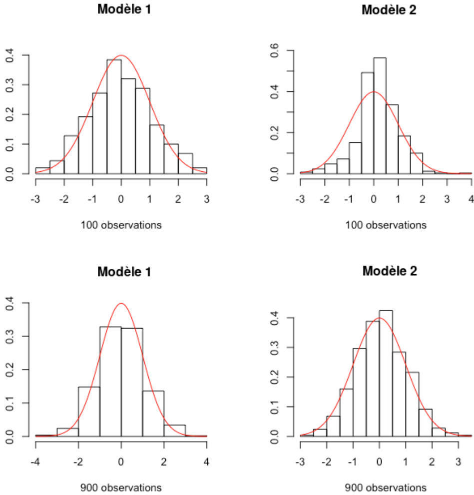
FIGURE 5.1. – Histogramme de \sqrt{2\sqrt{\pi}\hat{f}_{n_1}^{(\text{AR})}(0)n_1^2b_{n_1}r_{n_1}^{(\text{AR})}(0)} (Modèle 1) et \sqrt{2\sqrt{\pi}\hat{f}_{n_2}^{(\text{Vol})}(0)n_2^2b_{n_2}r_{n_2}^{(\text{Vol})}(0)} (Modèle 2) ainsi qu'une densité de la loi normale centrée réduite.
