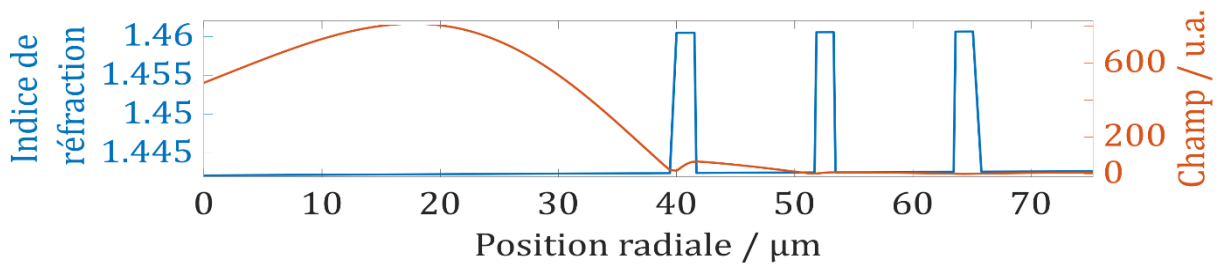
Figure 19 : Répartition transverse du champ électrique dans une fibre de Bragg courbée sur un rayon de 20 cm dont les motifs de la gaine ont été modifiés pour permettre des conditions d'antirésonance lors qu'une courbure est appliquée sur la fibre.
