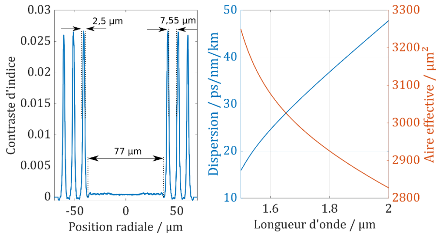
Figure 21 : Profil d'indice de réfraction, dispersion (courbe bleue) et aire effective du mode fondamental (courbe orange) de la fibre de Bragg de diamètre de cœur 77 \mu\text{m} optimisée pour des travaux à 1,7 \mu\text{m} , fabriquée au Fiber Optics Research Center.
