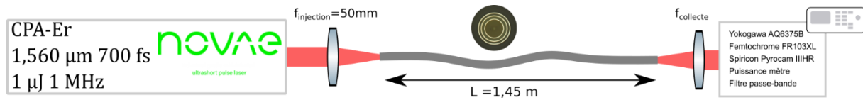
Figure 24 : Montage expérimental pour la génération d'impulsion solitonique dans la gamme 1,6 – 1,8 \mu\text{m} par effet solitonique dans 1,45 m de fibre Bragg de 77 \mu\text{m} de cœur pompé par une source de pompe CPA-Er de l'entreprise Novae.
