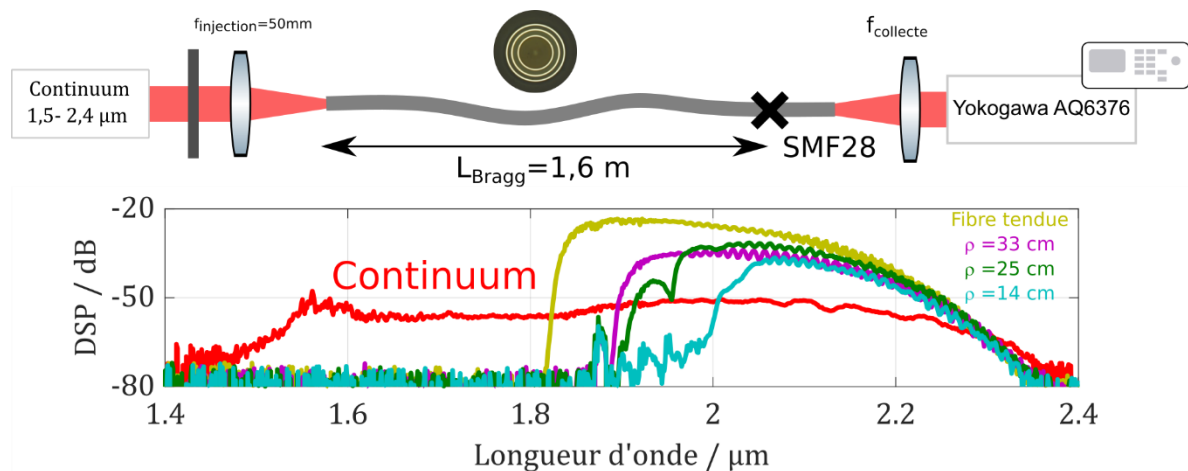
Figure 36 : Haut : montage expérimental pour la mesure de l'impact de la courbure sur la bande de transmission de la fibre de Bragg de 77 μm diamètre de cœur conçue pour des applications autour de 2 μm. Bas : spectres mesurés pour différentes courbures.
