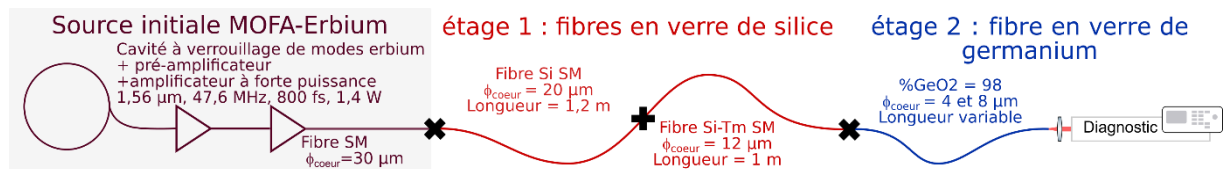
Figure 48 : Schéma du montage expérimental pour le décalage d'un soliton à \lambda > 2,4 \mu\text{m} dans une cascade de fibres à base de silice et de fibres de silice dopée germanium 98%.
