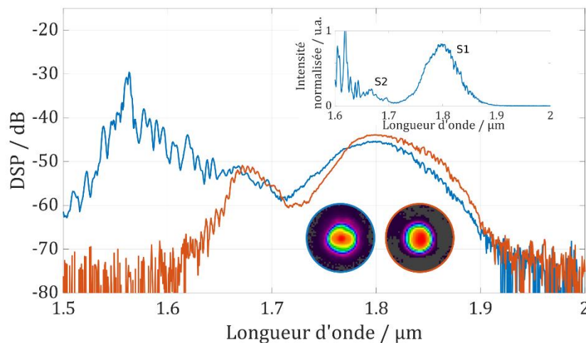
Figure 25 : Profil spectral, en dB et en linéaire, mesuré sans filtre (courbe bleue) et avec filtre passe-bande (courbe orange) à la sortie de 1,45 m de fibre de Bragg de 77 \mu\text{m} de diamètre de cœur pompée à 1,56 \mu\text{m} , 700 fs, 1 \mu\text{J} , 1 MHz. Insert : répartitions spatiales d'intensité mesurées sans filtre (cercle bleu) et avec filtre passe-bande (cercle orange). Paramètres des filtres : passe-bande 1,65 - 1,85 \mu\text{m} et passe-haut 1,56 \mu\text{m} .
