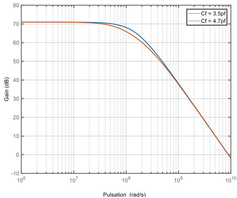
Figure V-7 : Fonction de transfert de l'amplificateur de transimpédance
