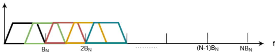
Figure II-10: Illustration de l'occupation de la bande passante par une modulation multi-porteuses avec recouvrement
