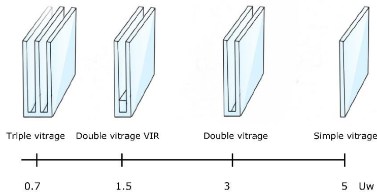
Figure 1-3 : Différents type d'assemblage de couches de verre en fonction du coefficient de transmission thermique, U_w , (en W \cdot K^{-1} \cdot m^{-2} )
