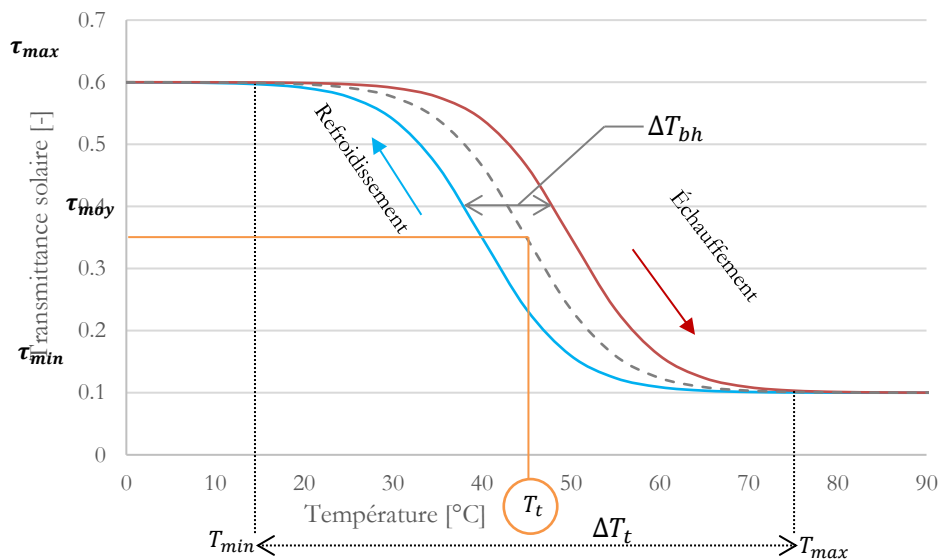
Figure 1-12 : Exemple de la transmittance solaire d'un vitrage thermochrome en fonction de sa température et cycle d'hystérésis
