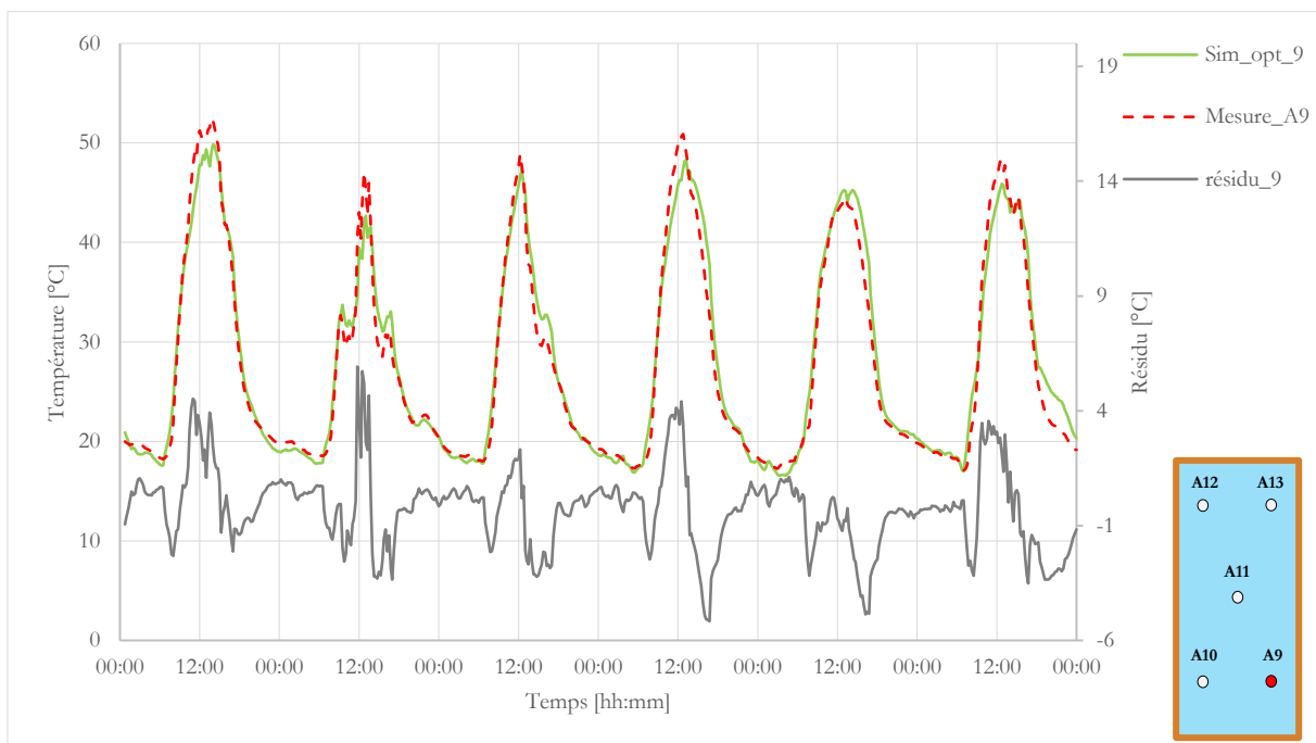
Figure 4-19 : Comparaison des profils de température entre la simulation pour le modèle convectif intérieur optimisé et la mesure pour la position A9
