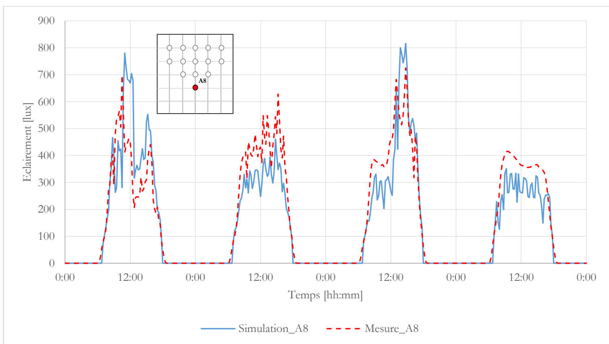
Figure 4-31 : Comparaison des profils d'éclaircement simulé et mesuré pour la position A8
