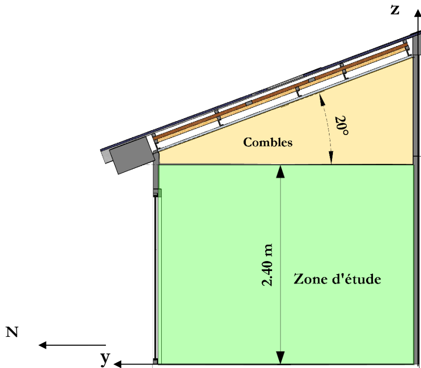
Figure 2-3 : Coupe transversale de la LGI
