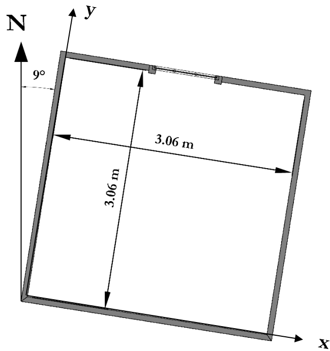
Figure 2-2 : Vue en plan de la LGI
