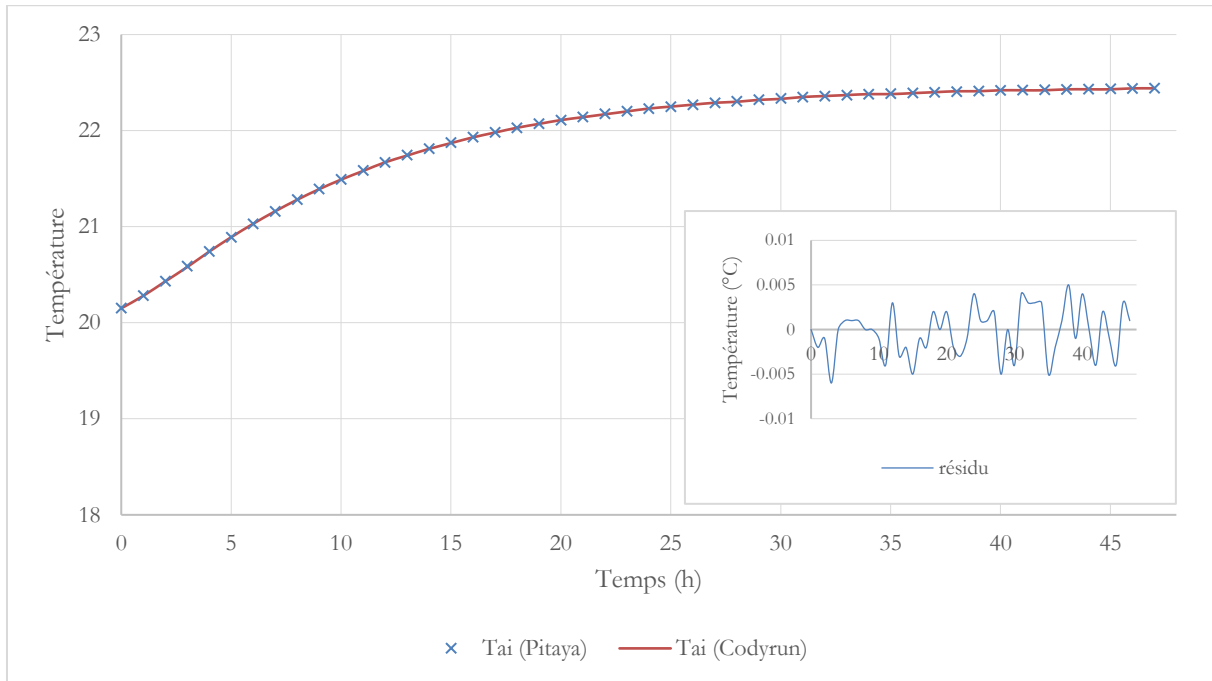
Figure 3-6 : Evolution de la température d'air et du résidu pour le scénario 1 entre PITAYA et CODYRUN
