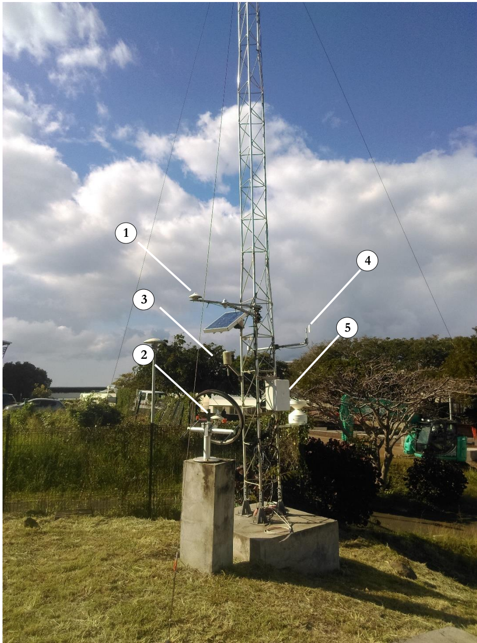
Figure 2-8 : Station météo n°1
