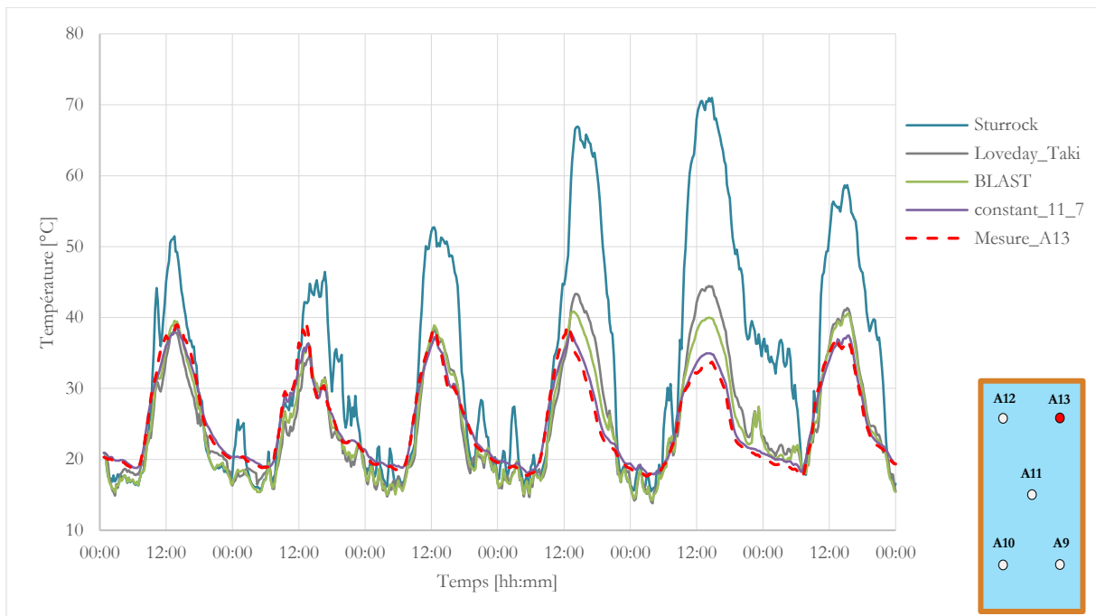
Figure 4-10 : Comparaison des profils de température entre les simulations pour différents modèles convectifs extérieurs et la mesure pour la position A13
