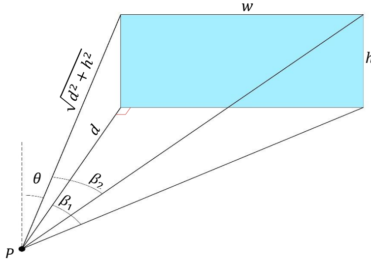
Figure 3-11 : Composante directe provenant d'une ouverture rectangulaire verticale (en bleue) pour un point P dans la pièce
