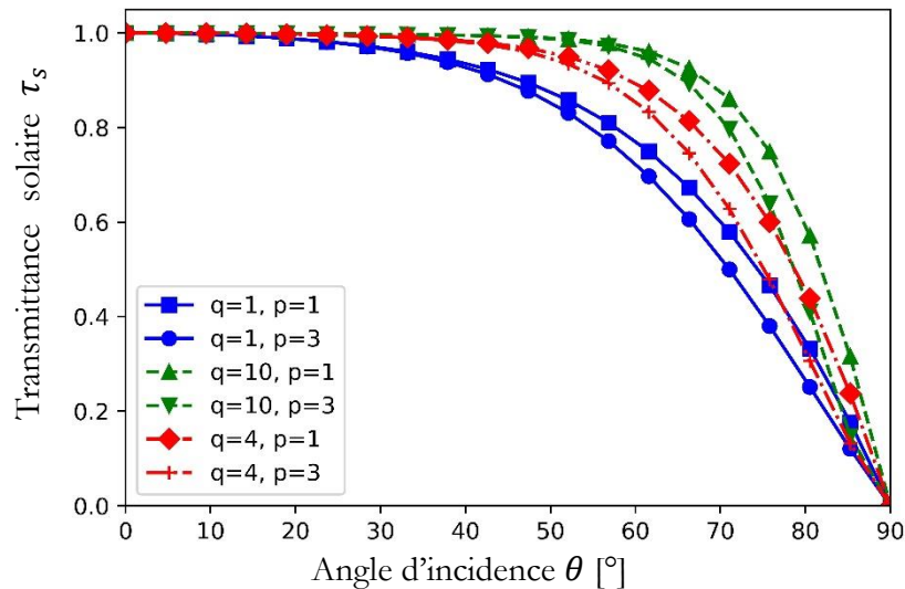
Figure 3-3 : Modèle polynomial de \tau_s , pour différents paramètres q , et nombres de couches de verre p (reproduit de J. Karlsson et al., 2001; Karlsson et Roos, 2000)
