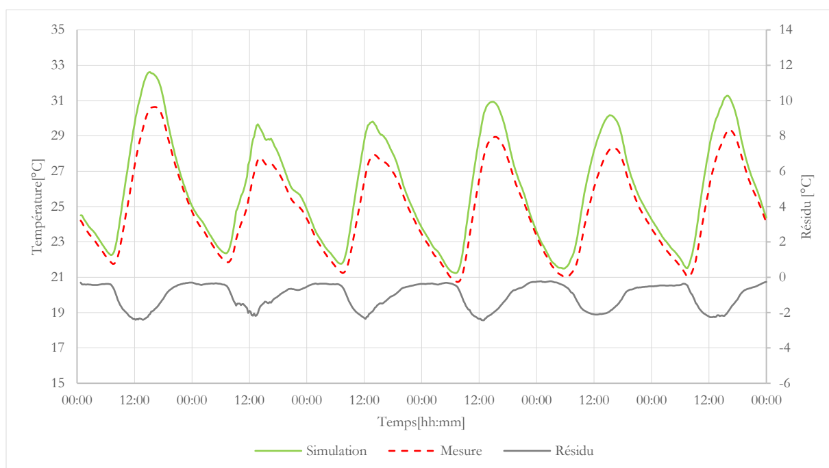
Figure 4-22 : Comparaison des profils de température d'air intérieur entre la simulation et la mesure avant optimisation
