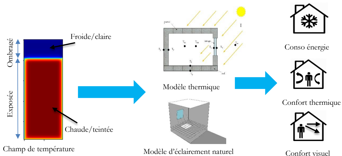
Figure 3-22 : Représentation schématique du couplage du modèle 2D vers le modèle de bâtiment 1D
