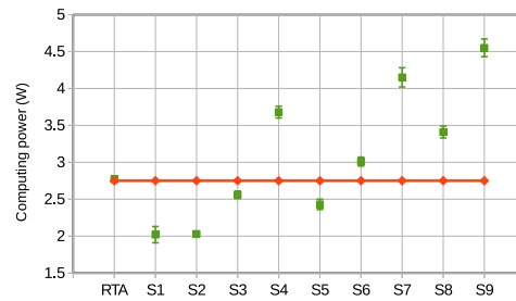
(D) Mean computing power consumption.
