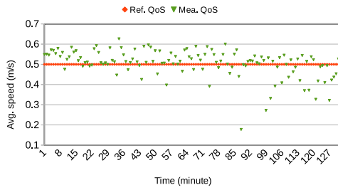
(D) Quality of service of Navigation Mission.
