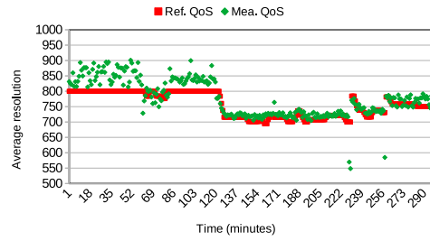
(D) Quality of service of Server Mission.
