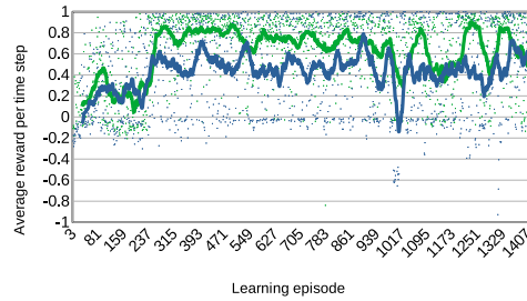
(D) Average reward per time step of Server Mission.
