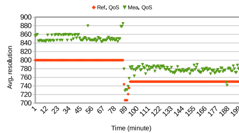
(D) Quality of service (RTA).
