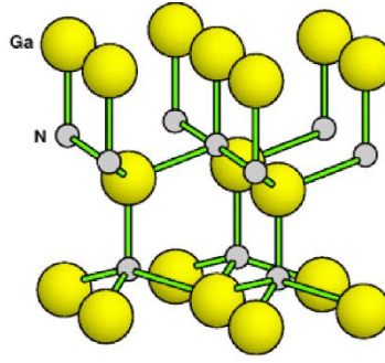
Fig. 2.21: Schematic of the wurzite GaN [32].
