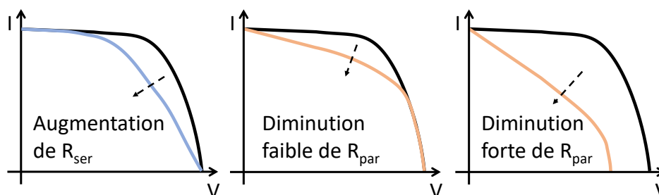
Figure 107. Incidence de l'augmentation de R_{ser} , et de la diminution de R_{par} sur une courbe I(V) d'une cellule solaire. Ces résistances n'impactent pas le J_{SC} ou le V_{OC} , excepté pour des faibles valeurs de résistance parallèle ( < 100 \Omega.cm^2 )
