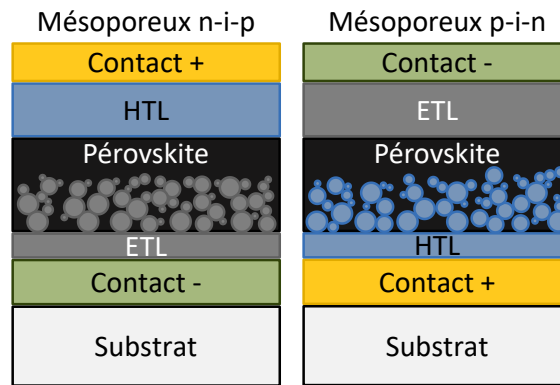
Figure 14. Structure de type mésoporeuse pour les cellules pérovskite n-i-p et p-i-n (l'éclairage est ici en face arrière)
