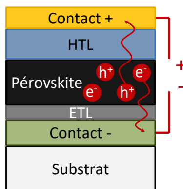
Figure 11. Structure générale d'une cellule solaire pérovskite. Le substrat est ici transparent, et l'éclairage provient de la face arrière
