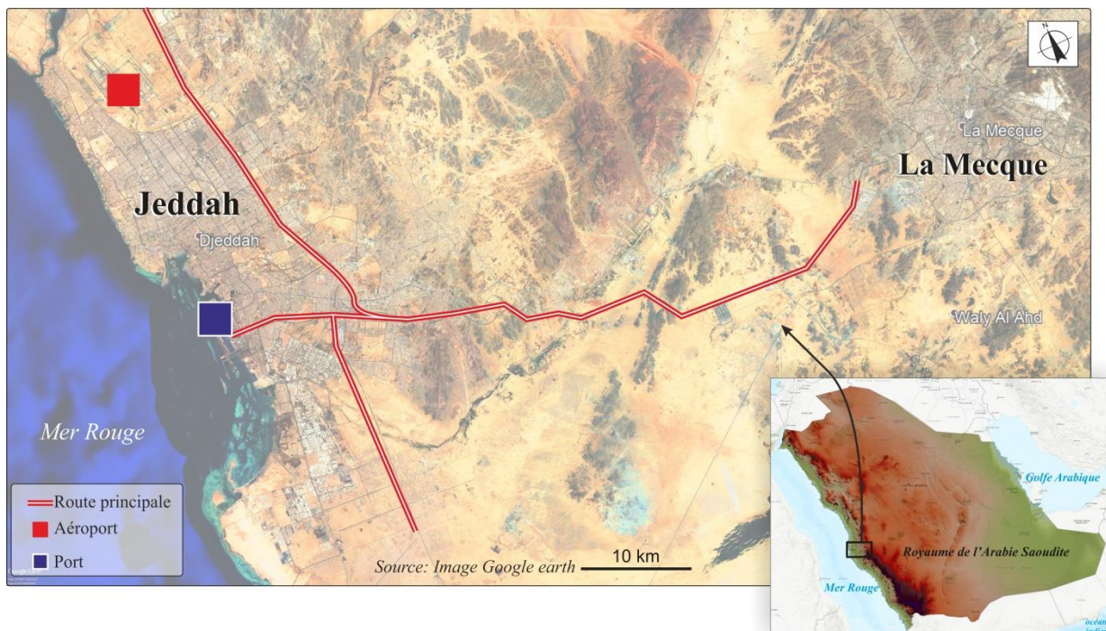
Figure 20: Vue aérienne des agglomérations de Jeddah et de La Mecque
