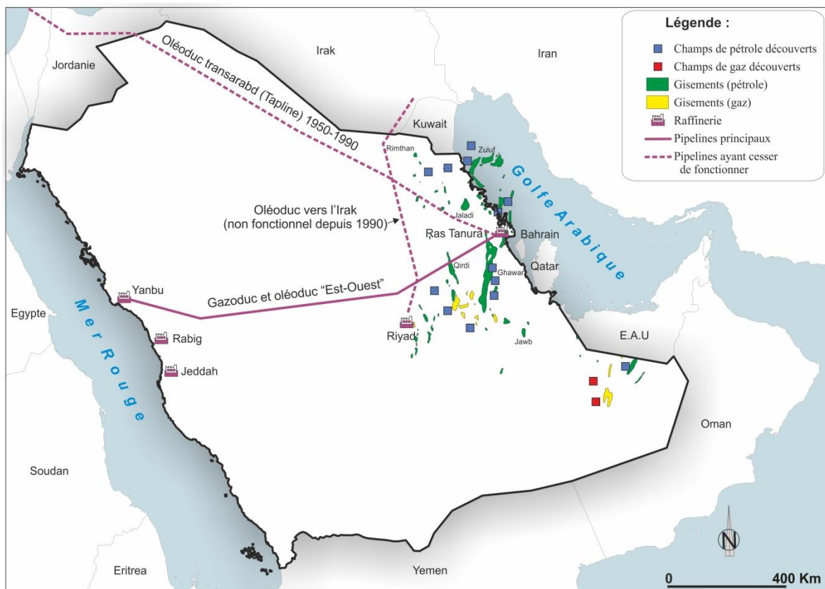
Figure 9: Localisation des champs pétroliers et gazeux et transfert des hydrocarbures
