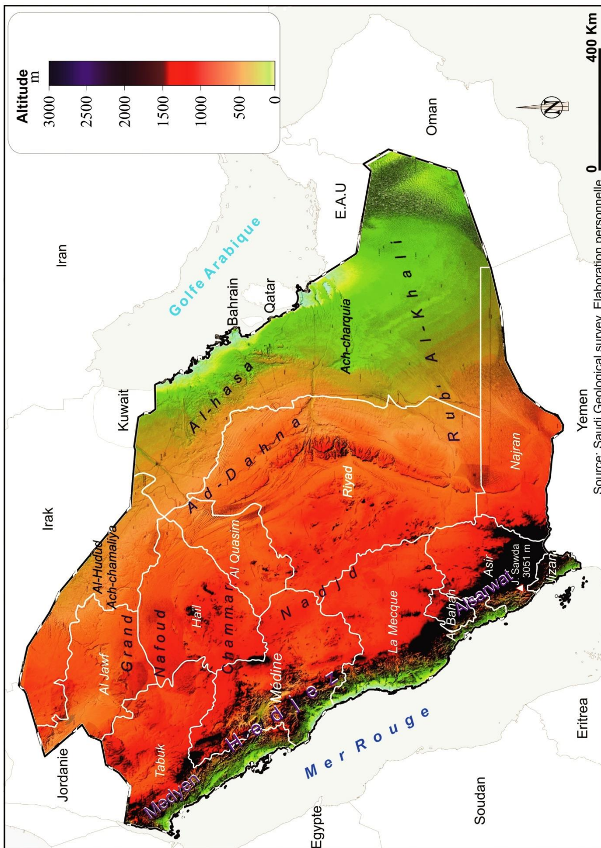
Figure 1: Les altitudes des unités topographiques de l'Arabie Saoudite
