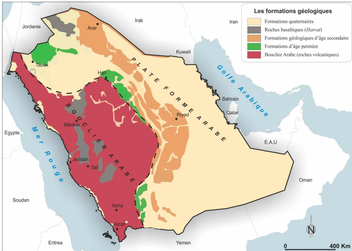
Figure 7: les principales formations géologiques en Arabie Saoudite
