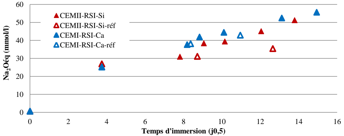
Evolution de la teneur en alcalins équivalent dans la solution de conservation des bétons CEMII-RSI-Si , CEMI-RSI-Ca , CEMII-RSI-Si-réf et CEMI-RSI-Ca-réf
