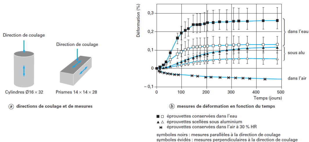
Figure I-33: Éprouvettes cylindrique et prismatique (a) et mesures de déformations (b)
