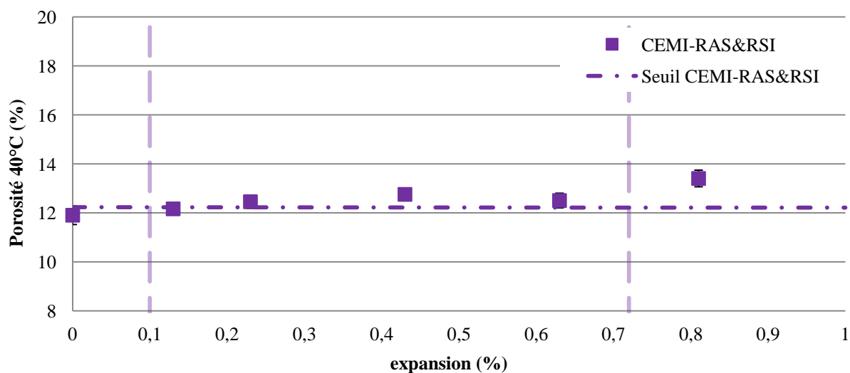
Figure III-41: Evolution de la porosité accessible à l'eau (séchage à 40°C) en fonction de l'expansion du béton CEMI-RAS&RSI
