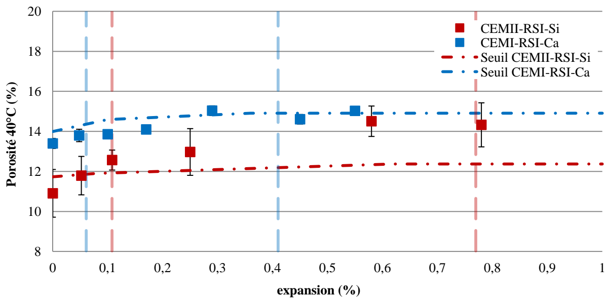
Figure III-37: Evolution de la porosité accessible à l'eau (séchage à 40°C) en fonction de l'expansion des bétons CEMI-RSI-Si et CEMI-RSI-Ca
