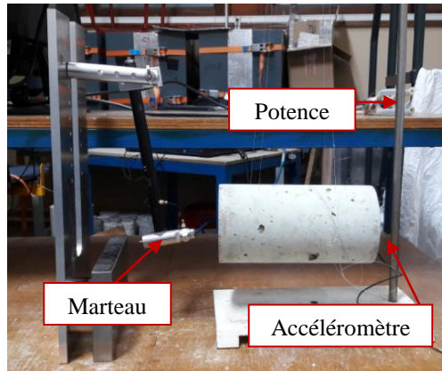
Figure II-14 : Mesure du module dynamique en acoustique non linéaire
