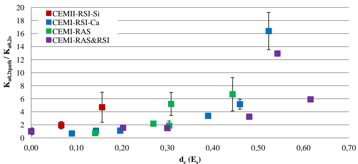
Figure IV-6 : Corrélation entre le rapport de la perméabilité apparente ( K_{a0,2tpath}/K_{a0,20} ) et l'endommagement mesuré par le module statique
