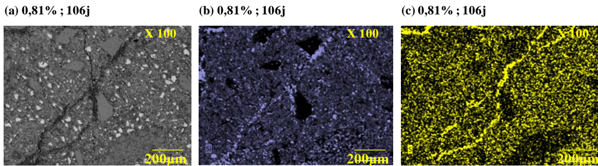
Figure III-21: Analyse MEB du béton CEMI-RAS&RSI (a) image initiale, (b) cartographie de la silice et (c) cartographie du soufre
