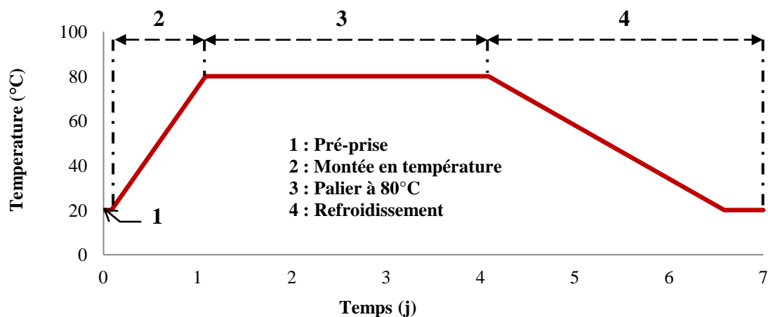
Figure II-3 : Traitement thermique appliqué aux bétons développant la RSI
