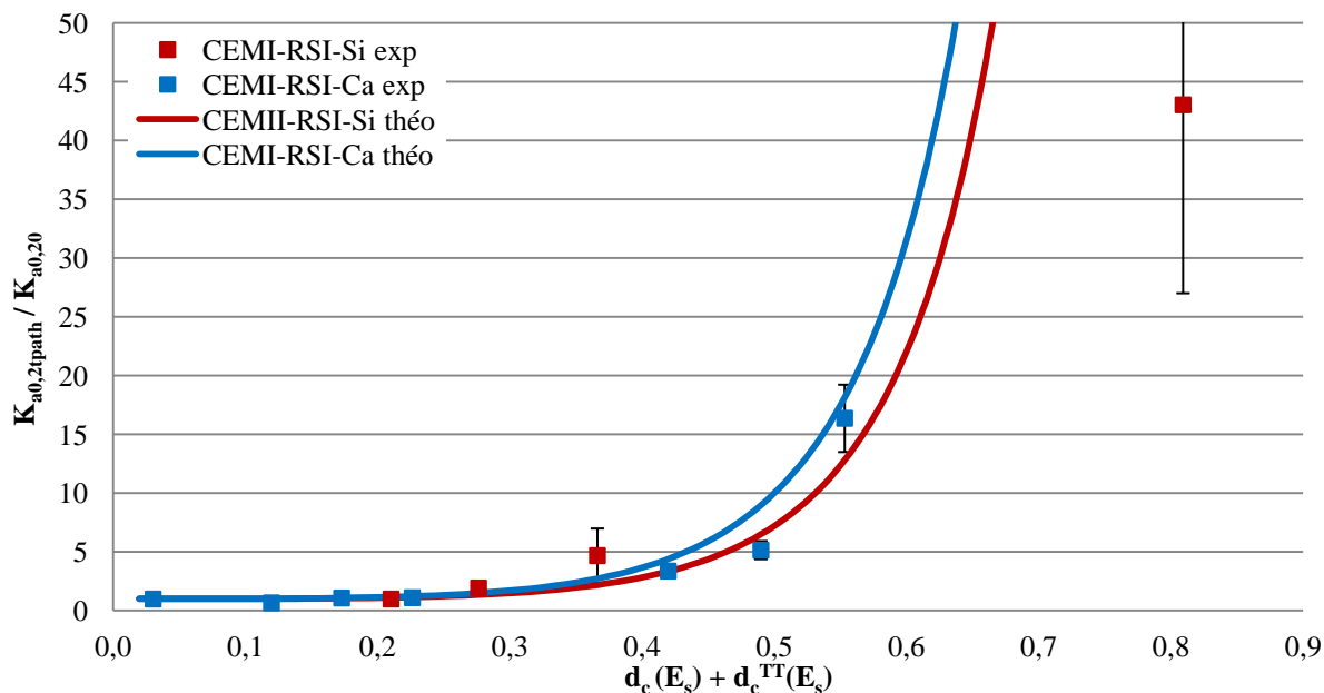
Figure IV-19 : Evolution du rapport de perméabilité K_{a0,2ipath} / K_{a0,2o} en fonction de l'endommagement (CEMI-RSI-Si, CEMI-RSI-Ca)
