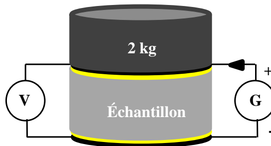
Figure II-17 : Schéma de l'essai de résistivité électrique (PerfDub, 2017 (2))
