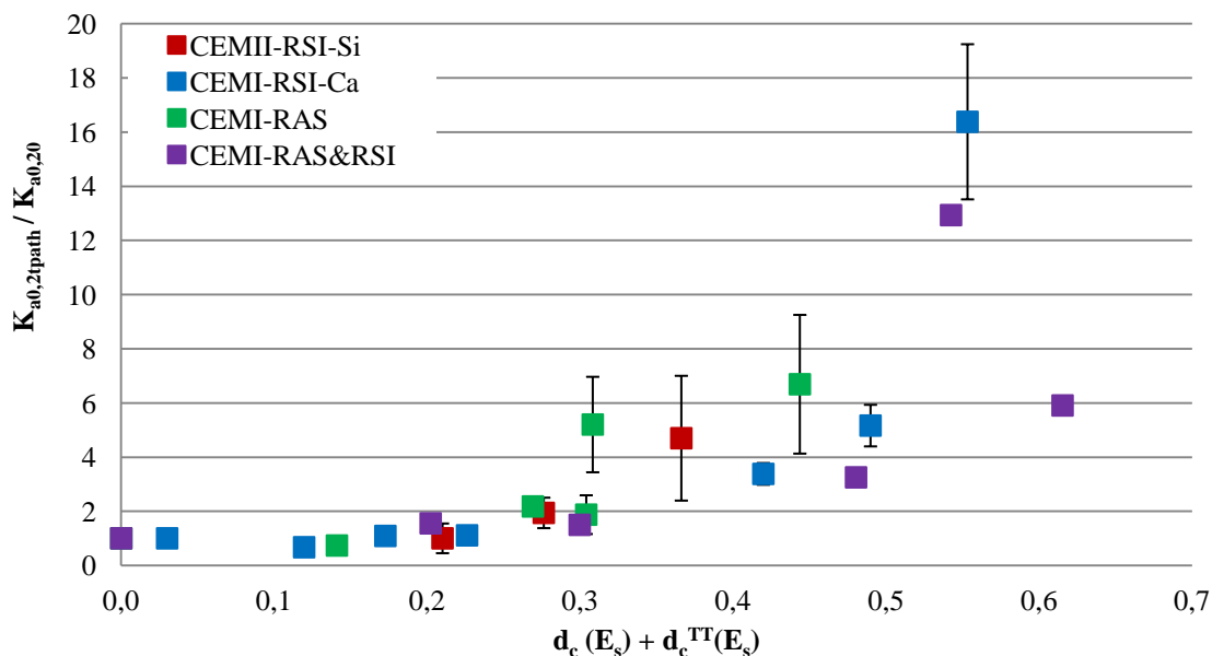
Figure IV-7 : Corrélation entre le rapport de perméabilité apparent ( K_{a0,2path}/K_{a0,20} ) et l'endommagement mesuré par le module statique (prise en compte du traitement thermique)
