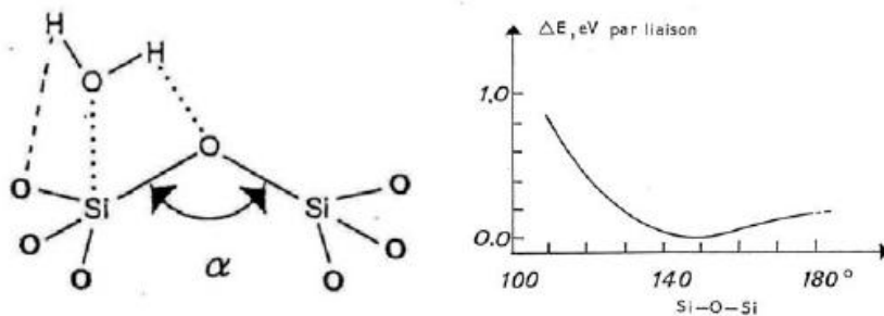
Figure I-35: Energie de la liaison en fonction de l'angle de la liaison siloxane (Couty, 1999)
