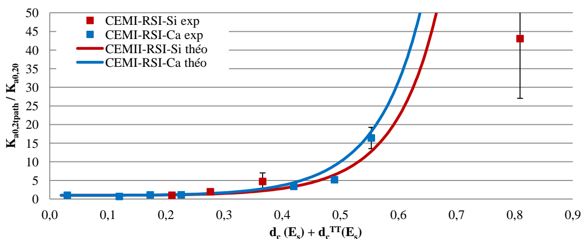
Figure IV-22 : Evolution du rapport de perméabilité K_{a0,2tpath}/K_{a0,2o} en fonction de l'endommagement ( \zeta, \chi ) (CEMII-RSI-Si et CEMI-RSI-Ca)
