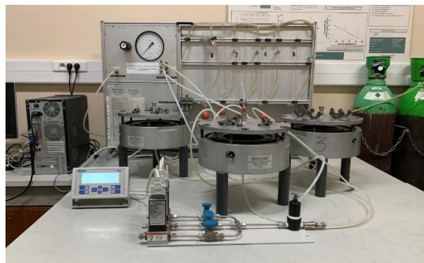
Figure II-15 : Perméamètre Cembureau
