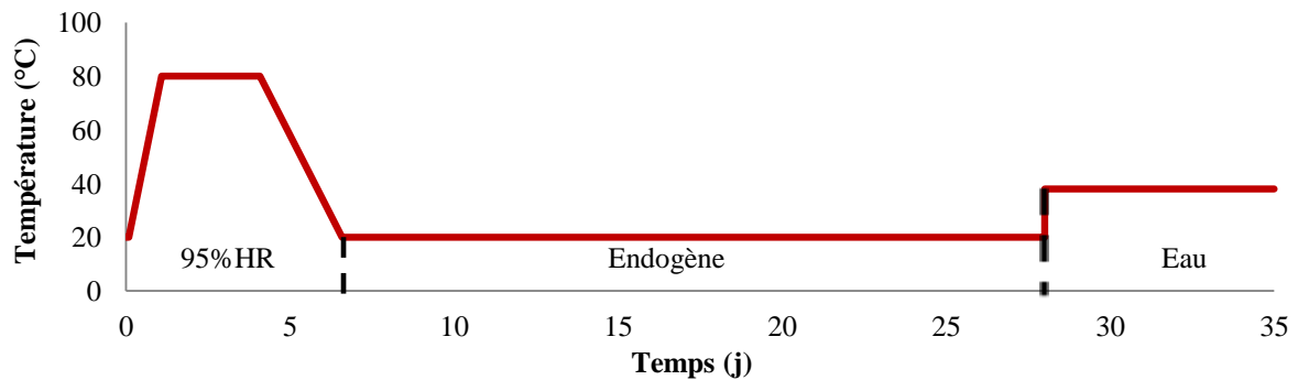
Figure II-9 : Environnement de conservation du béton développant les deux RGI
