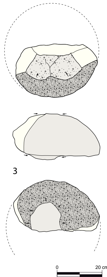
Figure 131 Ébauche de meule rotative gauloise n° 3 en Grès de Macquenoise découverte au fond de la douve du château du « Camp de Macquenoise ». Dessin éch. 1/10.
