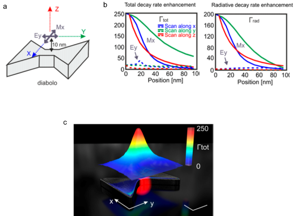
Figure 1.15 - a) Représentation en 3D d'un dipôle magnétique M_x et électrique E_y à proximité de la jonction métallique de la nano-antenne diabol. b) Taux de décroissance total et c) radiatif du dipôle électrique (ligne discontinue) et du dipôle magnétique (ligne continue) en fonction de la position des dipôles par rapport à la structure. c) MLDOS dans un plan transverse à proximité de la nano-antenne diabol. 25
