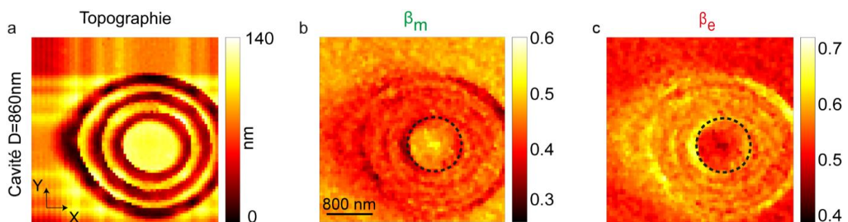
Figure 3.9 – a) Topographie de la surface scannée contenant la cavité plasmonique de diamètre D=860\text{nm} . La taille de l'image est de 3\times 3\ \mu\text{m}^2 . b) Branching ratio magnétique et c) électrique de la partie scannée. Les cercles noirs en pointillé délimitent la cavité. Durée approximative d'obtention de l'image : une heure.
