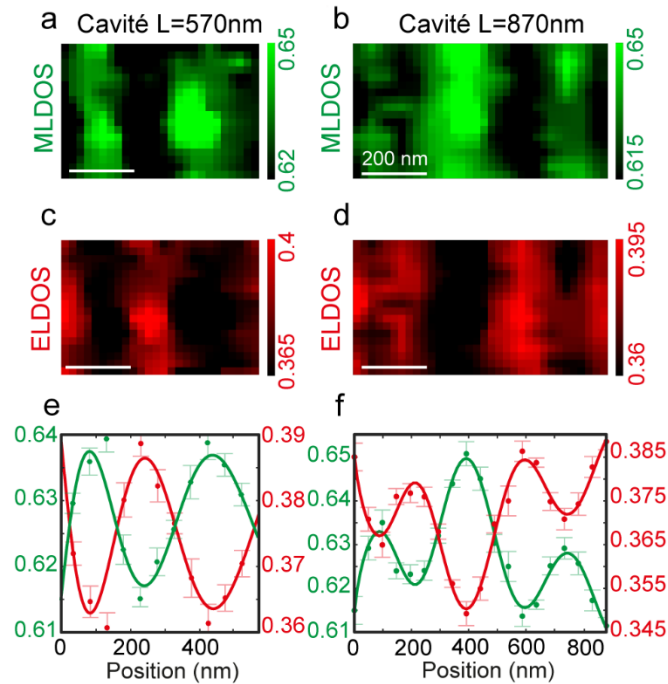
Figure 3.15 – Densité locale des états électroniques. Distributions expérimentales bidimensionnelles des a,b) MLDOS et c,d) ELDOS radiatives dans le plan de chaque cavités. (e, f) LDOS radiatives magnétiques (vert) et électriques (rouge) expérimentales le long des cavités sur une moyenne de 20 balayages. Les points représentent les données expérimentales, les lignes complètes représentent un fit polynomiale et les barres d'erreur représentent l'erreur type de la moyenne.
