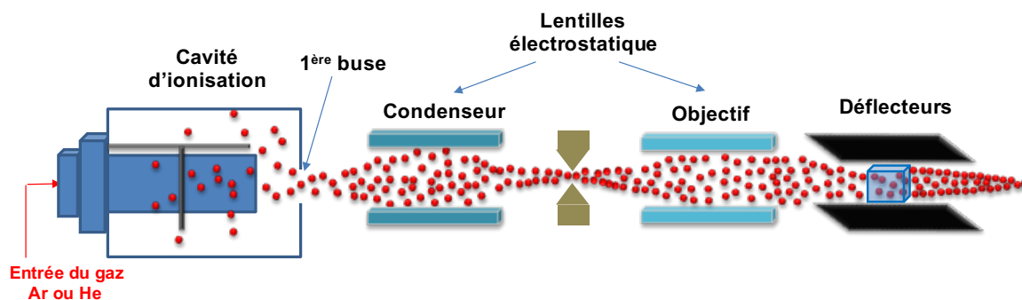
FIGURE 3.6 – Schéma simplifié du canon à ions et du mode de production du faisceau d'ions.
