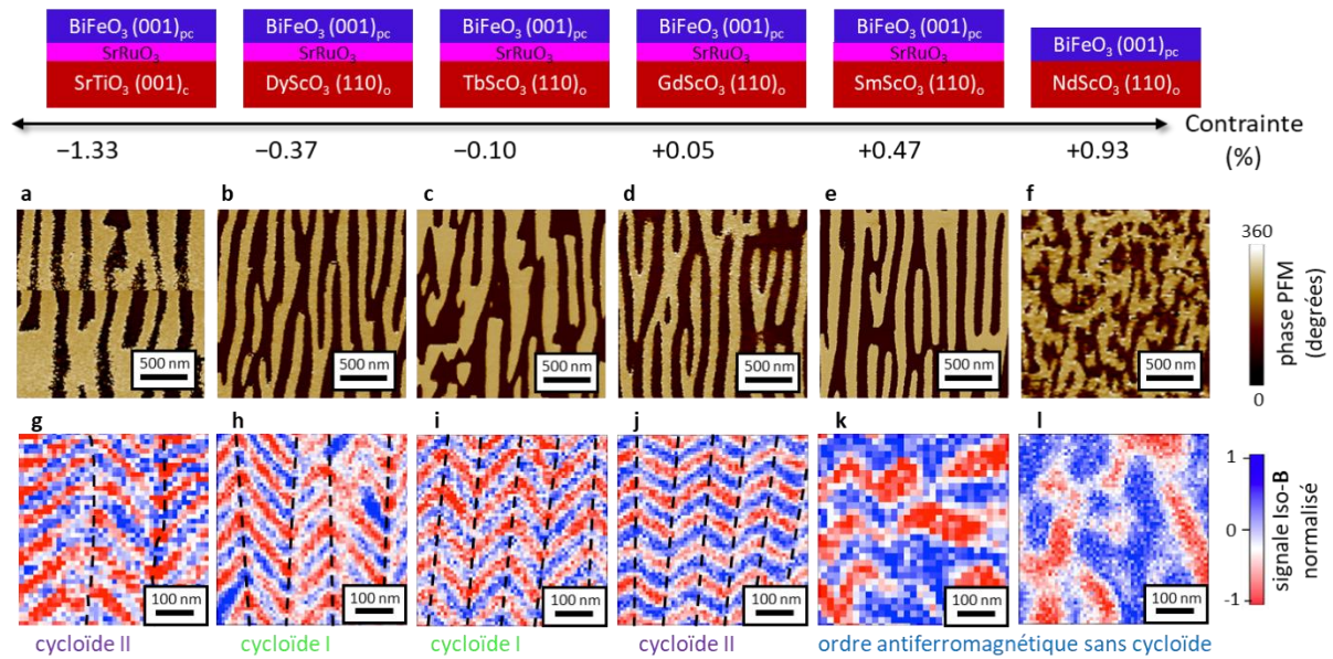
Figure 94 : Corrélation entre les textures électriques et magnétiques dans les films minces de \text{BiFeO}_3 soumis à différentes contraintes épitaxiales. Les différents substrats utilisés sont représentés schématiquement. a-f Images en microscopie à force piézoélectrique de la structure des domaines ferroélectriques (phase dans le plan). Hormis le cas sur \text{NdScO}_3 , les films de \text{BiFeO}_3 présentent une structure sous formes de bandes de deux variantes de polarisation. g-l Textures antiferromagnétiques associées, imagées par la magnétométrie à centre NV. Figure adaptée de la référence [136].
