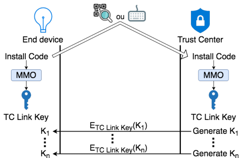
FIGURE A.4 – Procédure d'ajout d'un appareil dans un réseau Zigbee centralisé et renouvellement des clés
