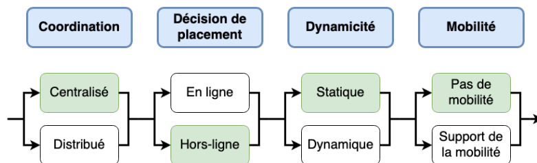
FIGURE 3.3 – Nos conditions de placement selon la taxonomie du placement de Service de Salaht et al. [229])
