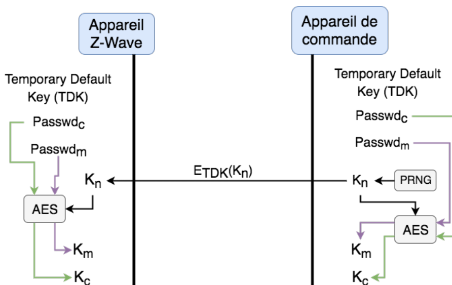
FIGURE A.5 – Échange de clés dans le protocole Z-Wave
