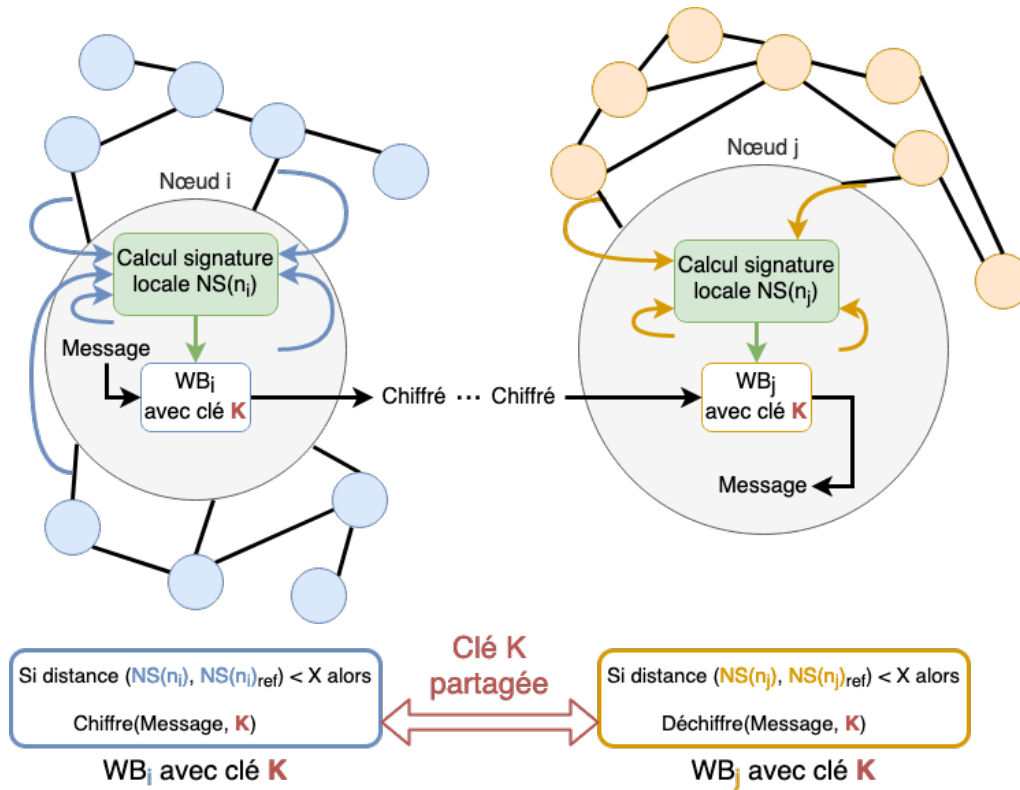
FIGURE 5.9 – Présentation du fonctionnement de l'ancrage d'implémentation white-box avec partage de la même clé de chiffrement.
