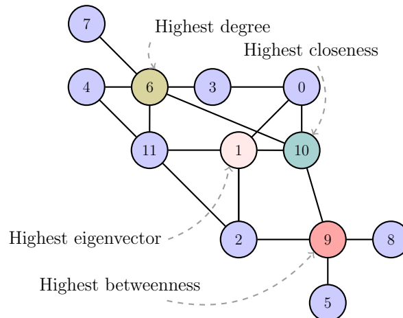
FIGURE 3.7 – Différences entre valeurs de centralité sur un graphe donné.
