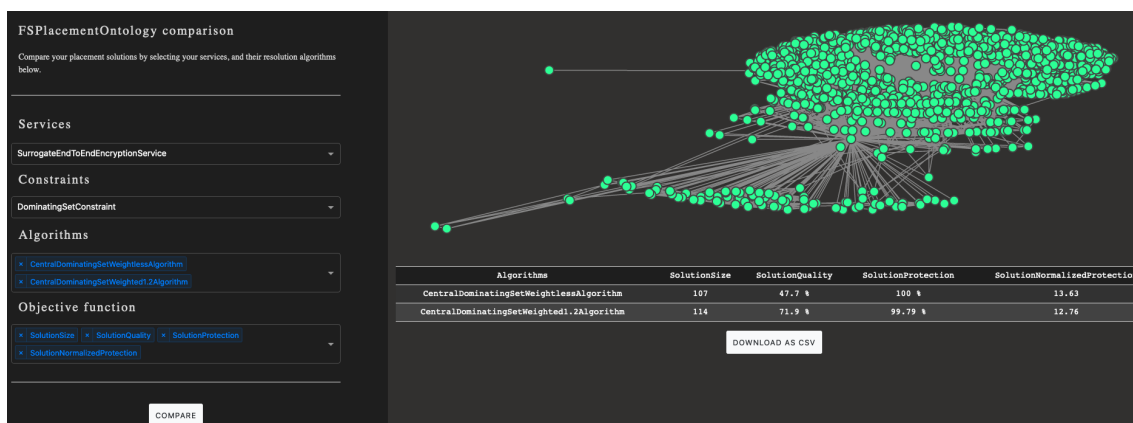
FIGURE 4.8 – Aperçu de l'interface de CSPS.
