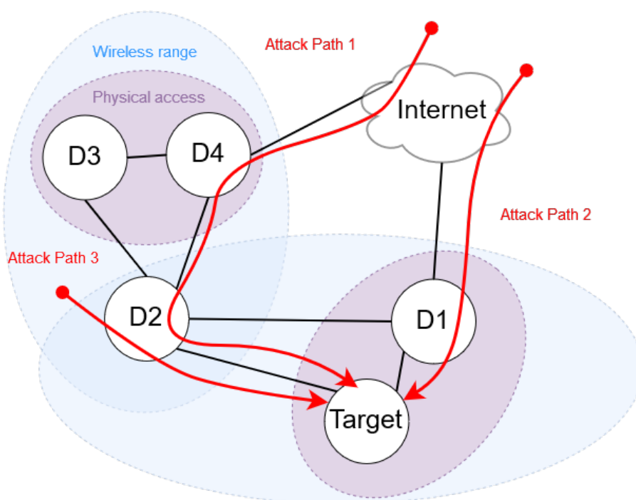
FIGURE 3.4 – Exemples de chemins d'attaque par un attaquant de type outsider .
