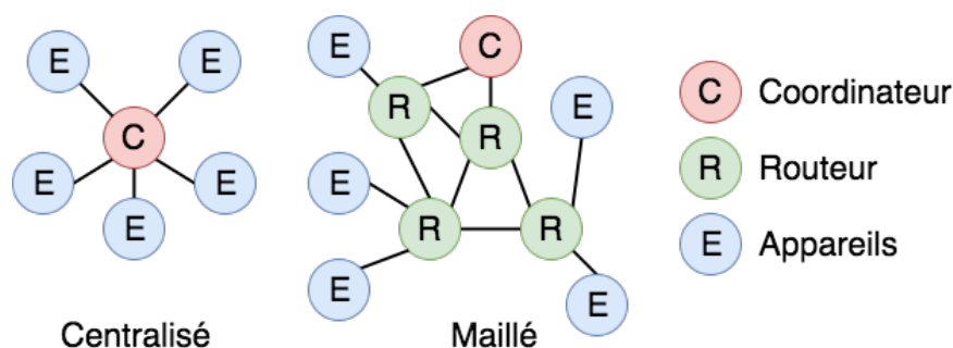
FIGURE A.3 – Les structures de réseau Zigbee
