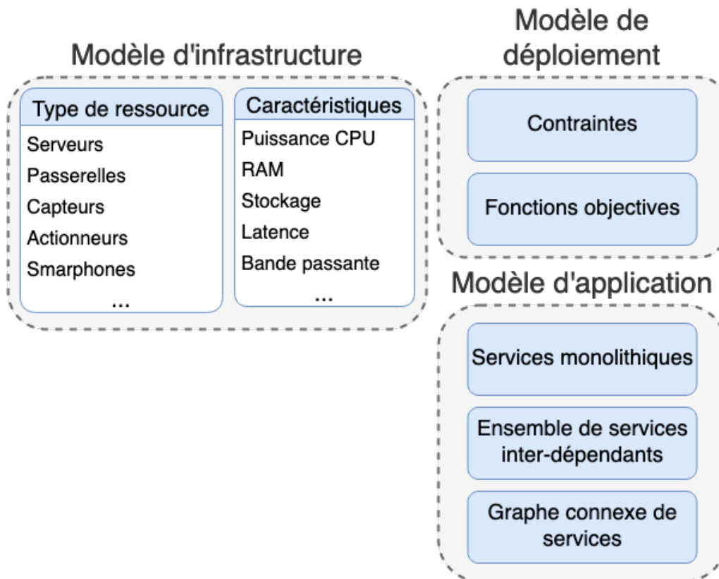
FIGURE 3.1 – Aperçu des modèles pour la description du problème de placement de service (SPP) (inspiré de [229])
