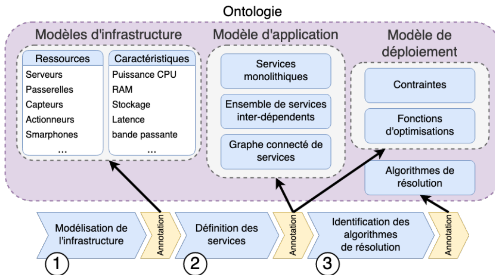
FIGURE 4.3 – Processus de constitution de notre base de connaissance.
