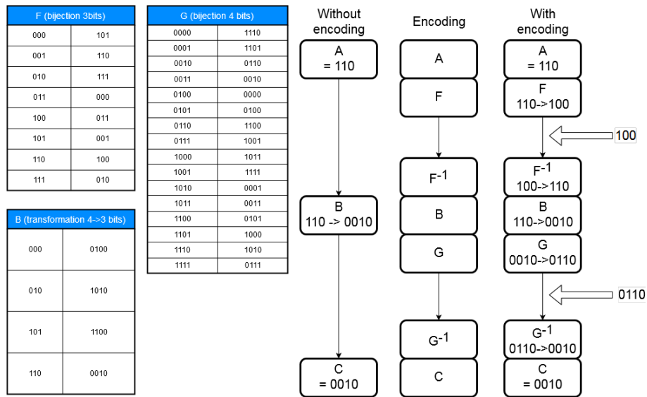
FIGURE 5.1 – Exemple d’encodage via des bijections (F et G) aléatoires.
