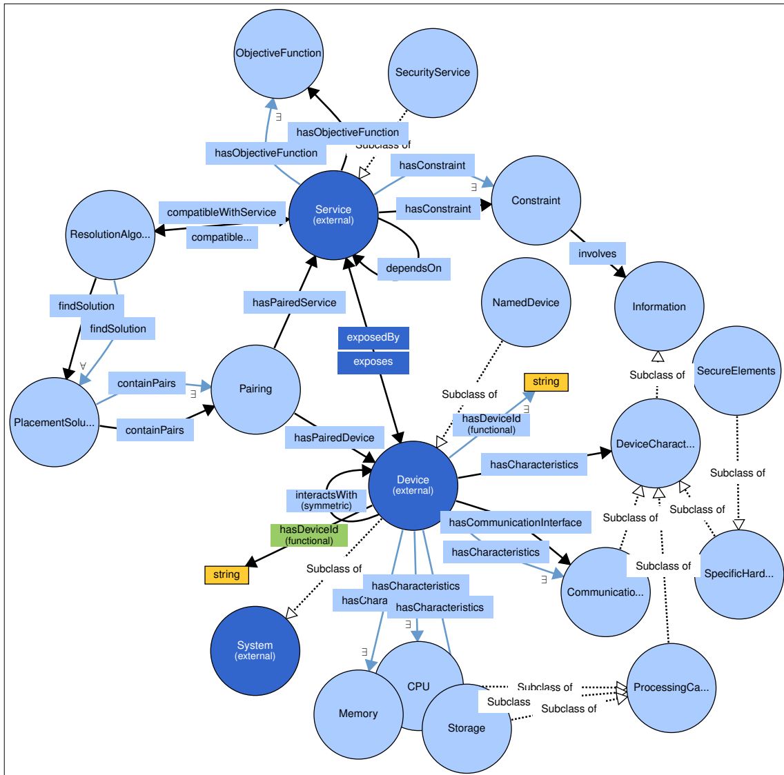
FIGURE 4.6 – Visualisation de FSPlacementOntology d’après l’outil de visualisation WebVOWL 4
