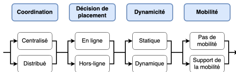
FIGURE 3.2 – Taxonomie du placement de Service (inspiré de [229])
