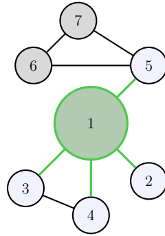
FIGURE 5.11 – Environnement local (vert) du noeud 1.
