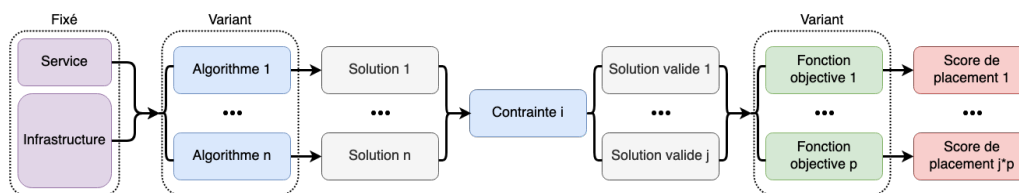
FIGURE 4.2 – Principe et enchaînement des éléments de l'ontologie pour l'identification et la comparaison des solutions de placement de services.
