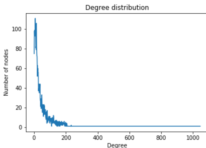
FIGURE 3.14 – Distribution des degrés du graphe Ego-Facebook [182].
