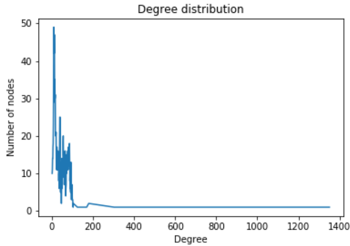
FIGURE 3.13 – Distribution des degrés du graphe IoT
