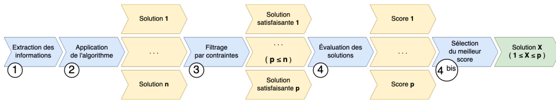
FIGURE 4.4 – Résolution d'un problème de placement utilisant la base de connaissance.
