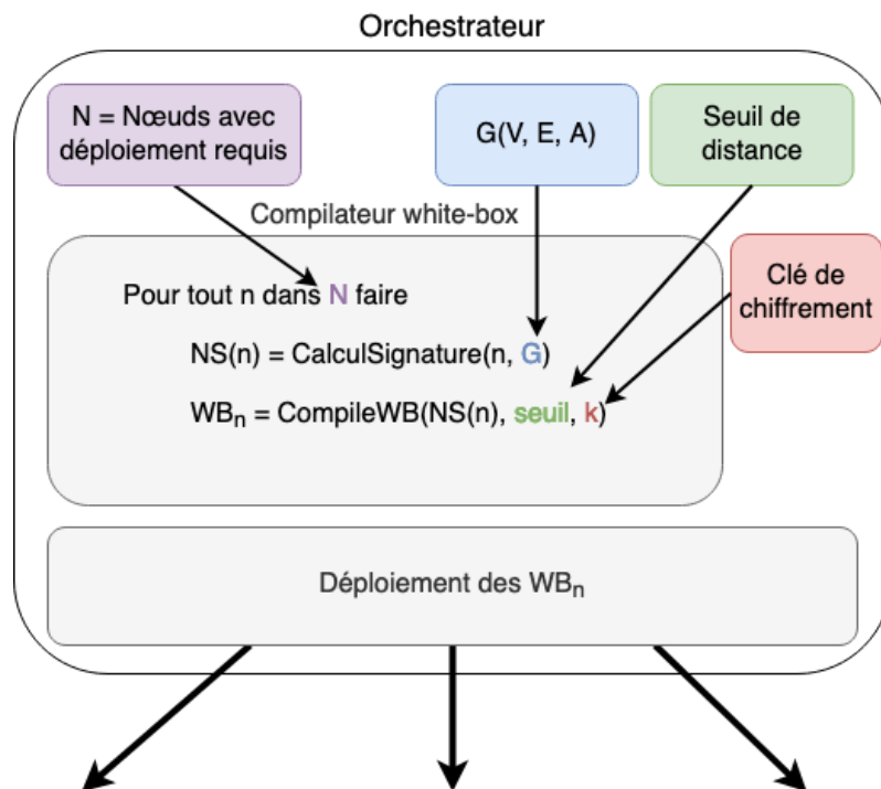
FIGURE 5.7 – Principe de génération d'une implémentation white-box ancrée.
