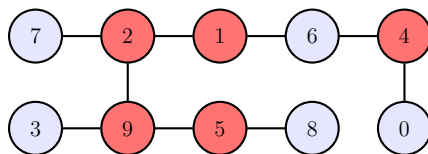
FIGURE 3.10 – Ensemble dominant (rouge) identifié avec notre méthodologie sur le graphe de la Figure 3.6.
