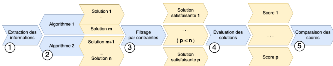
FIGURE 4.5 – Processus de comparaison des solutions de placement.
