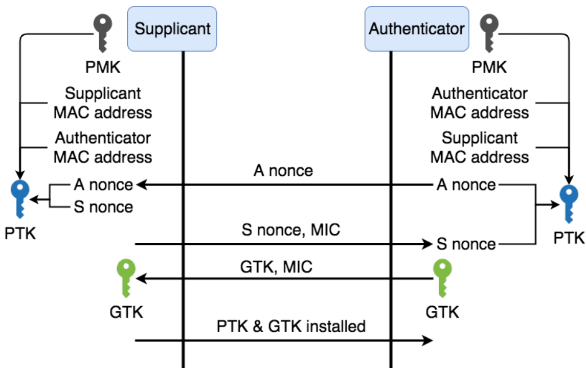
FIGURE A.2 – Représentation du 4 way handshake utilisé dans WPA
