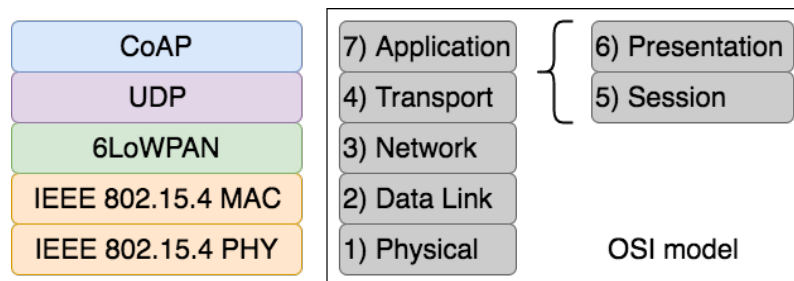
FIGURE A.7 – Position de CoAP par rapport au modèle OSI [161, 57]
