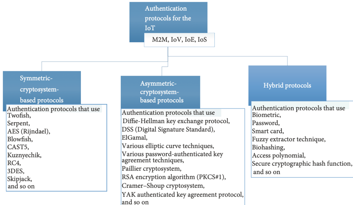
FIGURE 2.4 – Classification des protocoles d'authentification pour l'IoT d'après leurs cryptosystèmes (source : [104])
