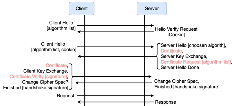
FIGURE A.8 – DTLS handshake avec requête. Les données en rouge ne sont pas transmises dans le mode PreSharedKey (source : [259, 207])
