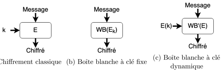
FIGURE 5.2 – Catégories d’implémentations cryptographiques boîte blanche (source : [266])
