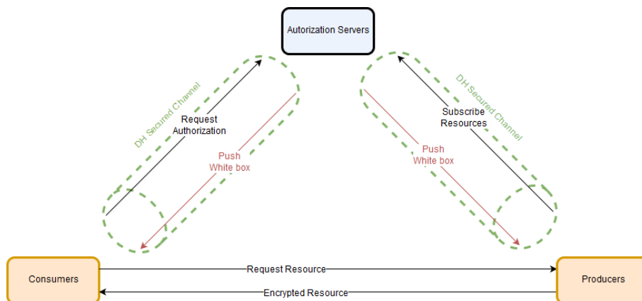
FIGURE 5.3 – Exemple d'utilisation de white box sur l'architecture OSCAR
