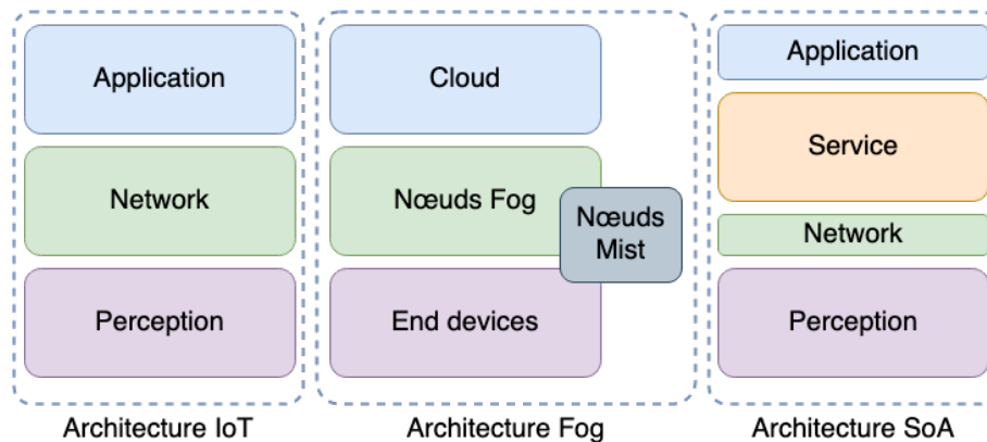
FIGURE 2.1 – Mise en correspondance des architectures IoT, Fog et SoA.
