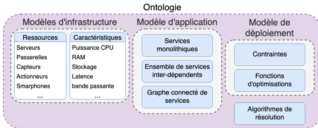
FIGURE 4.1 – Illustration des concepts à définir dans notre ontologie.
