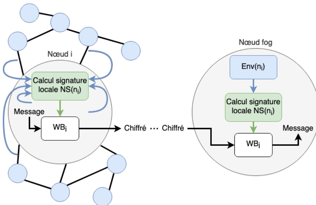
FIGURE 5.8 – Présentation du fonctionnement de l'ancrage d'implémentation white-box avec partage du même programme.
