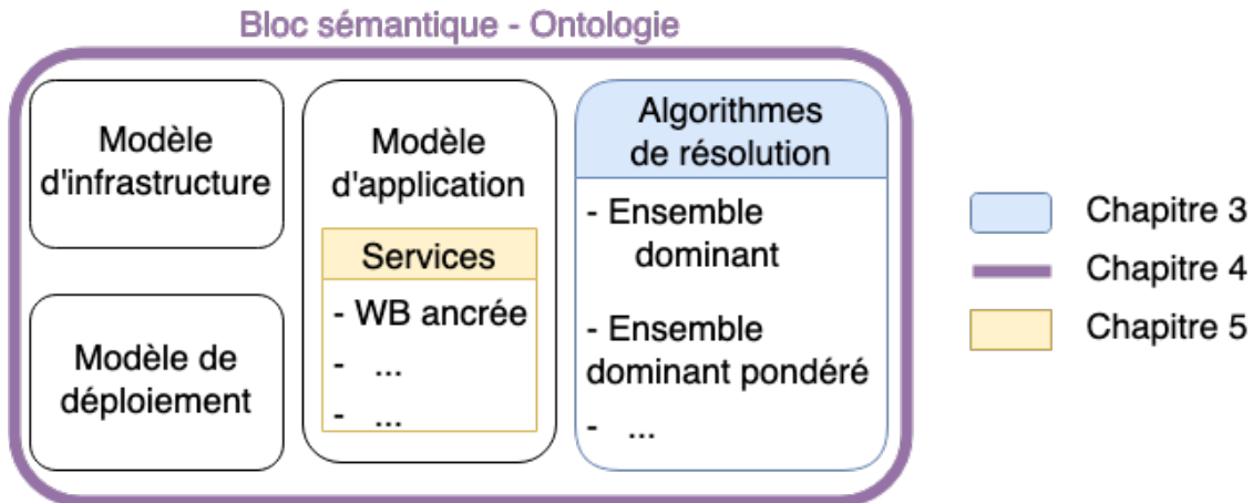
FIGURE 6.3 – Positionnement des contributions sur le bloc sémantique de notre framework de sécurisation adaptatif des objets de l'IoT.
