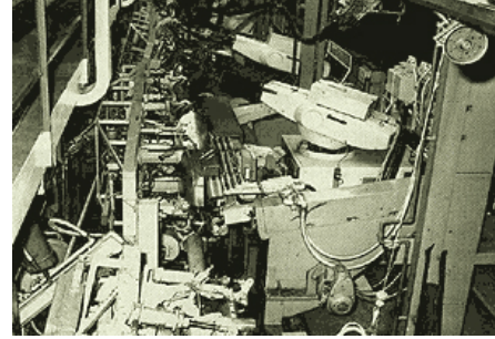
(b) Première ligne de soudage (Crédit IFR)
