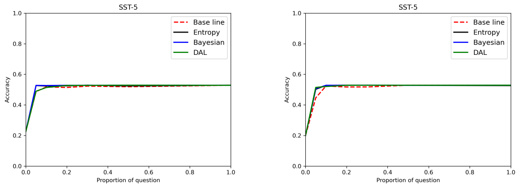
FIGURE IV.7 – L’abscisse représente la proportion des questions posées à l’oracle au regard du nombre de questions possibles et l’ordonnée, l’exactitude du classifieur. Le graphique de la première colonne correspond à l’architecture BERT tandis que la deuxième colonne correspond à l’architecture XLNet (jeu de données SST).
