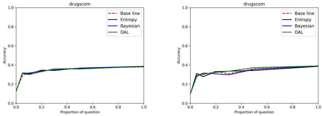
FIGURE IV.6 – L’abscisse représente la proportion des questions posées à l’oracle au regard du nombre de questions possibles et l’ordonnée, l’exactitude du classifieur. Le graphique de la première colonne correspond à l’architecture BERT tandis que la deuxième colonne correspond à l’architecture XLNet (jeu de données Drugs.com).
