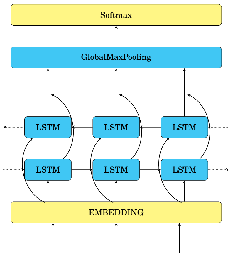
FIGURE III.5 – Réseau LSTM
