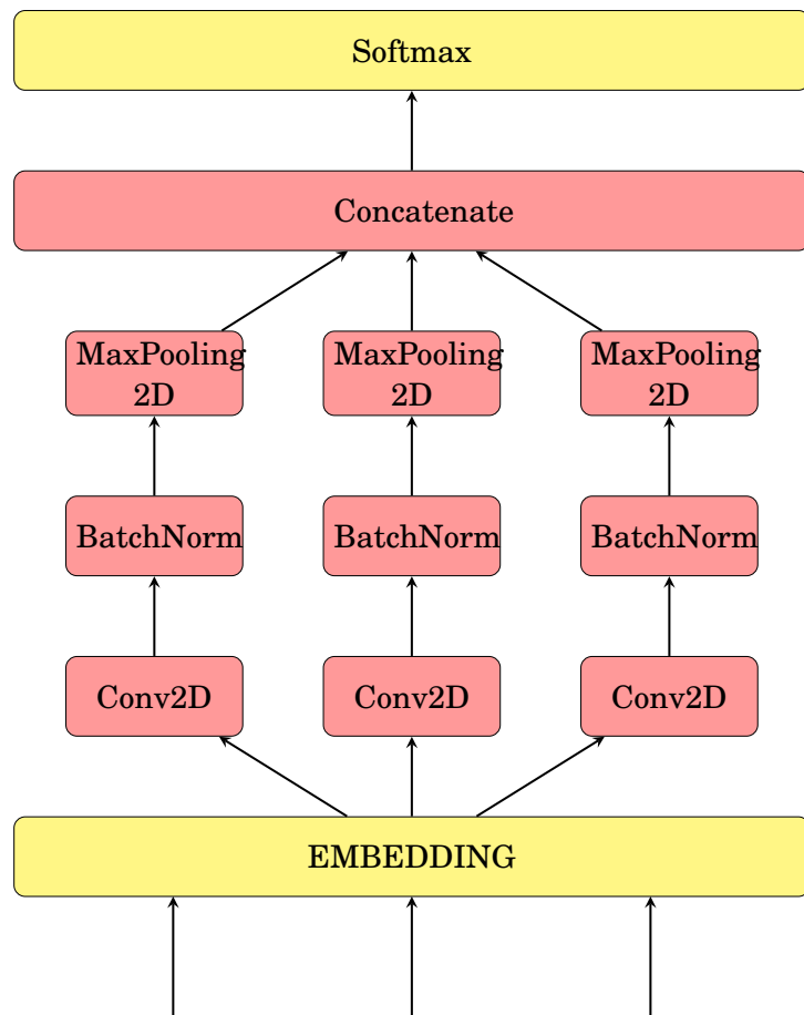
FIGURE III.4 – Réseau CNN
