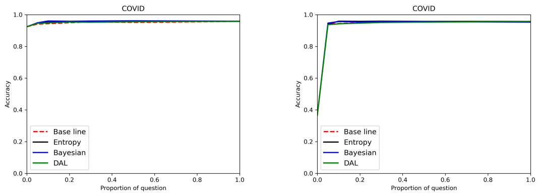
FIGURE IV.3 – L’abscisse représente la proportion des questions posées à l’oracle au regard du nombre de questions possibles et l’ordonnée, l’exactitude du classifieur. Le graphique de la première colonne correspond à l’architecture BERT tandis que la deuxième colonne correspond à l’architecture XLNet (jeu de données COVID 19).
