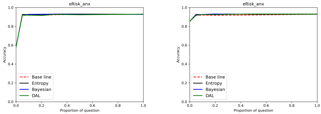
FIGURE IV.5 – L’abscisse représente la proportion des questions posées à l’oracle au regard du nombre de questions possibles et l’ordonnée, l’exactitude du classifieur. Le graphique de la première colonne correspond à l’architecture BERT tandis que la deuxième colonne correspond à l’architecture XLNet (jeu de données eRisk anorexie).
