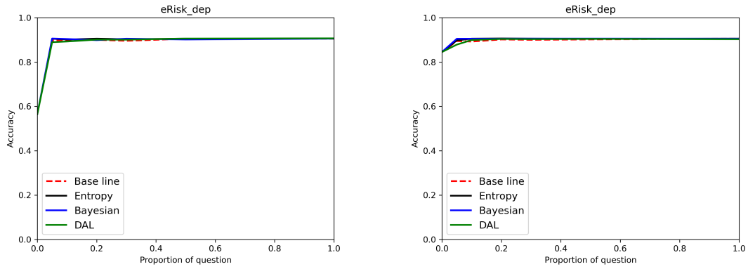
FIGURE IV.4 – L’abscisse représente la proportion des questions posées à l’oracle au regard du nombre de questions possibles et l’ordonnée, l’exactitude du classifieur. Le graphique de la première colonne correspond à l’architecture BERT tandis que la deuxième colonne correspond à l’architecture XLNet (jeu de données eRisk dépression).
