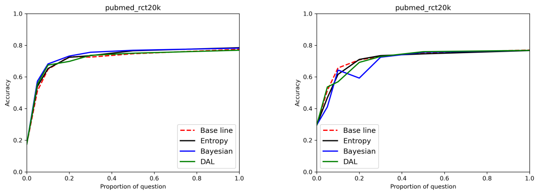
FIGURE IV.2 – L’abscisse représente la proportion des questions posées à l’oracle au regard du nombre de questions possibles et l’ordonnée, l’exactitude du classifieur. Le graphique de la première colonne correspond à l’architecture BERT tandis que la deuxième colonne correspond à l’architecture XLNet (jeu de données PubMed RCT).
