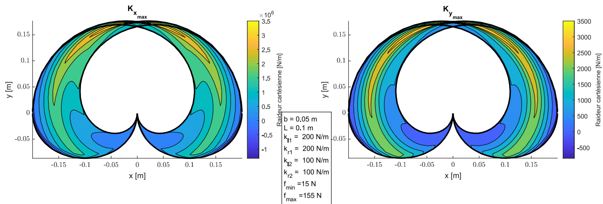
FIGURE 4.23 – Espace de travail accessible et raideur cartésienne maximale pour la stratégie strut-routed.
