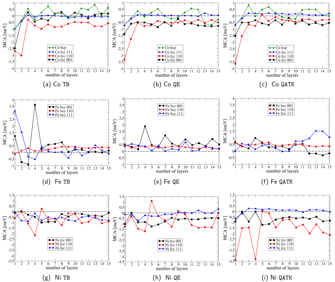
Figure 2.3 – MCA = E_{\parallel} - E_{\perp} en fonction de l'épaisseur de la couche mince. A chaque abscisse est associée la sommation des MCA de chaque site pour un système de N couches. Les différents éléments, cobalt, fer et nickel, sont représentés sur la première, deuxième et troisième ligne, respectivement. Les méthodes utilisées, TB, QE et QATK, sont représentées sur la première, deuxième et troisième colonne, respectivement.
