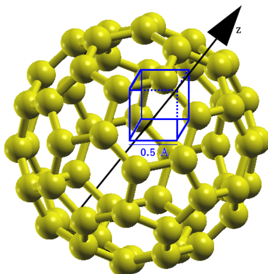
Figure 4.15 – Exemple d'une boîte fictive de vide dans laquelle nous calculons les densités d'état électronique déposée sur un fullerène en liaison hexagonale.
