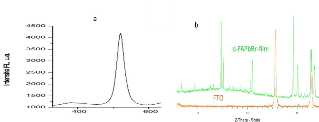
Figure 3. 13 : (a) Spectre de photoluminescence (PL) d'un film du d-FAPbBr ;(b) diffractogramme expérimental d'un film de d-FAPbBr( \lambda_{ex}=320nm ).
