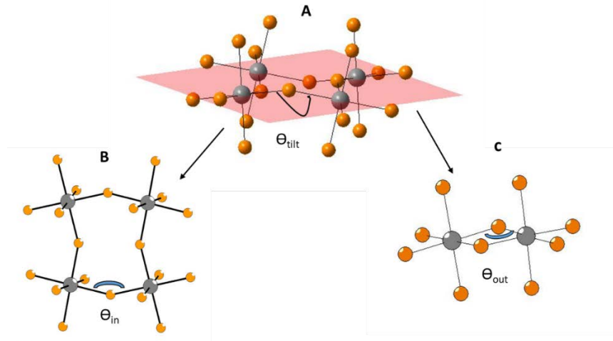
Figure 1. 25 : A) Schéma montrant \Theta_{\text{tilt}} (angle Br-Pb-Br) dans une couche pérovskite, et sa projection dans le plan défini par les atomes de plomb ( \Theta_{\text{in}} , B) et dans un plan perpendiculaire ( \Theta_{\text{out}} , C). 80
