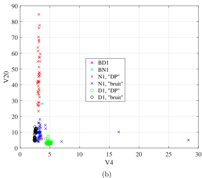
FIGURE 5.32 – Représentation des exemples dans l'espace des deux variables n^o4 ( V4 ) et n^o20 ( V20 ) dans les environnements d'apprentissage D1 et de test D2 (a) et N1 (b).
