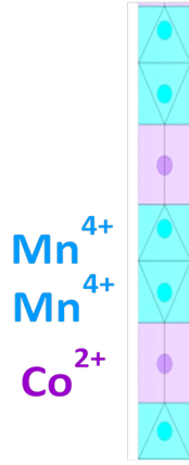
FIGURE 7.1 – Structure des chaînes du composé Sr_2Ca_2CoMn_2O_9 . Les prismes trigonaux en violet sont remplis par Co^{2+} et les octaèdres en cyan sont occupés par Mn^{4+} . Les chaînes sont le long de l'axe c .
