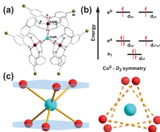
FIGURE A.3 – (a) représente la structure moléculaire du complexe [\text{HNEt}_3][\text{Co}(\text{II})\text{Co}(\text{III})_3\text{L}_6] . (b) montre la configuration électronique simplifiée d^7 pour l'ion \text{Co}(\text{II}) avec symétrie D_3 . (c) montre l'environnement de coordination de l'ion central \text{Co}(\text{II}) (coordination six). Figure extraite de [51].
