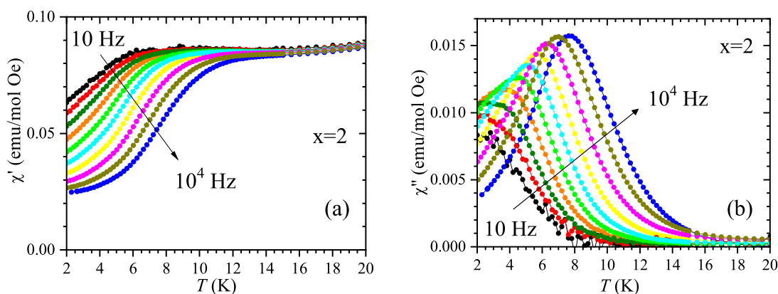
FIGURE 2.14 – Évolution de \chi'_{ac} (a) et \chi''_{ac} (b) de la susceptibilité magnétique alternative en fonction de la température et pour différentes fréquences du composé x=2 . Ces fréquences sont : 10, 21, 46, 100, 464, 1000, 2154, 4641 et 10000 Hz.
