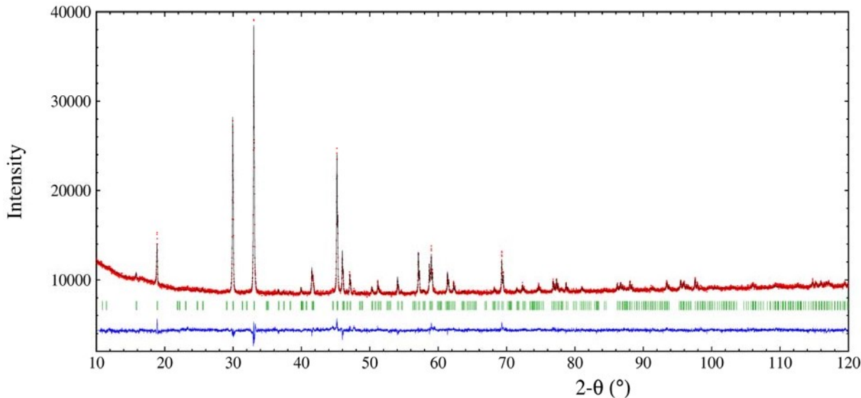
FIGURE 2.6 – Diagramme de diffraction des rayons X sur poudre et à température ambiante du composé \text{Sr}_2\text{Ca}_2\text{CoMn}_2\text{O}_9 ( x=2 ). Les diagrammes en noir et rouge correspondent respectivement au diagramme mesuré et affiné par la méthode de Rietveld. La différence entre ces deux derniers est en bleu. Les traits verts verticaux marquent les pics de Bragg.
