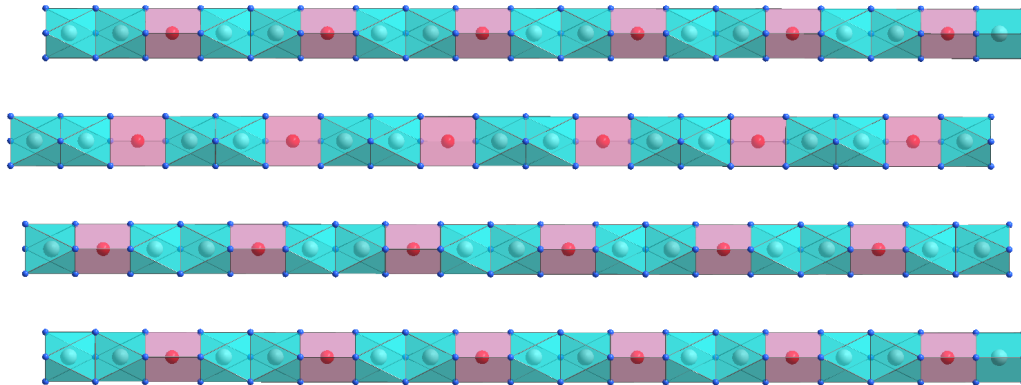
FIGURE 6.9 – Structure des chaînes commensurables du composé x=0 . Les prismes trigonaux, occupés par les ions Co^{2+} , sont en rose et les octaèdres, occupés par les ions Mn^{4+} , sont en cyan. Les atomes d’oxygène sont en bleu.
