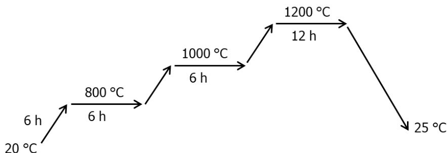
FIGURE 6.7 – Schéma du cycle thermique employé pour la synthèse de la céramique x=0 en tube scellé.
