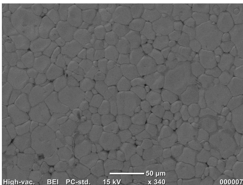
Figure V-3 : Microstructure en surface du BCTZ de référence calciné à 1200 °C pendant 2 heures et fritté à 1350 °C durant 3 heures observée par MEB.
