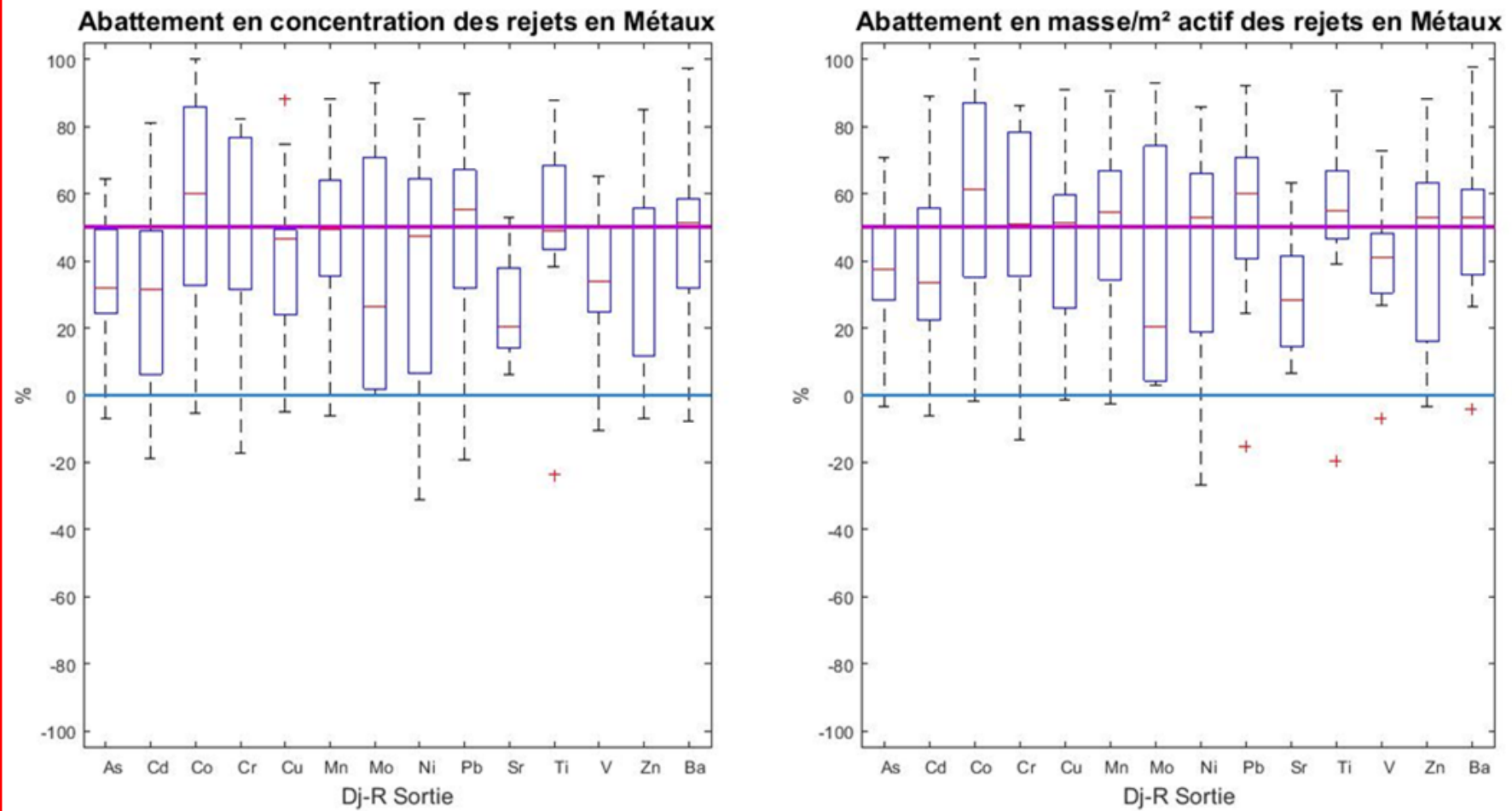
Figure 3.43 : Abatement en concentration (gauche) et masse (droite) de polluants pour les métaux du bassin de retenue de Django-Reinhardt
