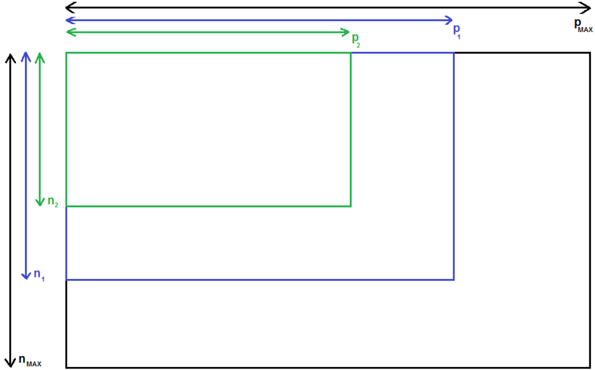
FIGURE 4.1 – Découpage de la matrice de données de l'ensemble d'apprentissage. Les matrices de génotypes incluent (n_{max}, n_1, n_2) = (10000, 5000, 1000) individus. Pour les génotypes simulés (p_{max}, p_1, p_2) = (5 \times 10^5, 10^5, 10^4) et pour les génotypes de UK-Biobank (p_{max}, p_1, p_2) = (417106, 10^5, 10^4)
