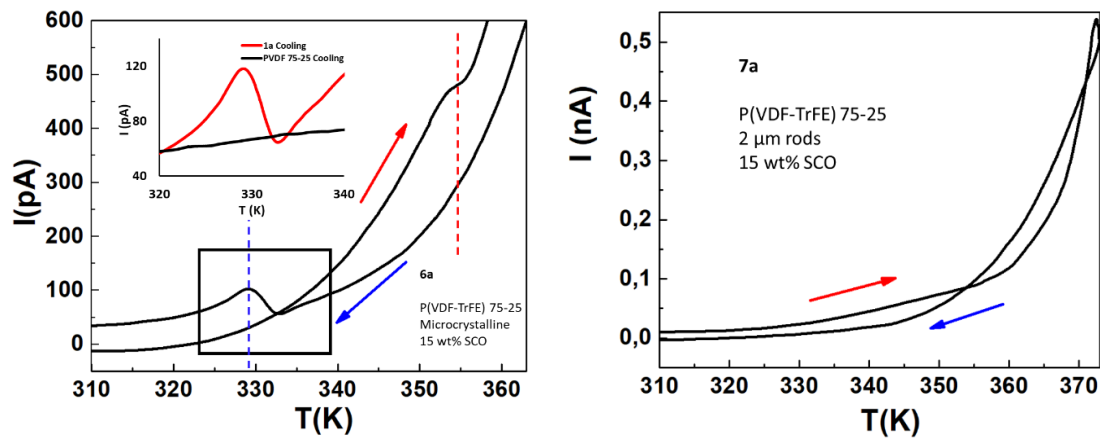
Fig 9) Cycle de décharge pyroélectrique pour les échantillons polarisés 6a et 7a . Les flèches indiquent le chauffage et le refroidissement. Les lignes en pointillés indiquent les pics de décharge liés à la TS pour le refroidissement (à gauche) et le chauffage (à droite). L'encadré montre une comparaison entre l'échantillon 6a et le PVDF-TrFE 75-25 pur (courant corrigé par la proportion de polymère).
