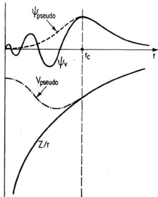
Figure 31: Représentation schématique du comportement de la fonction d'onde et du potentiel en considérant tous les électrons (trait plein) ou en utilisant un pseudopotential (pointillés). Extrait de Payne (1992).
