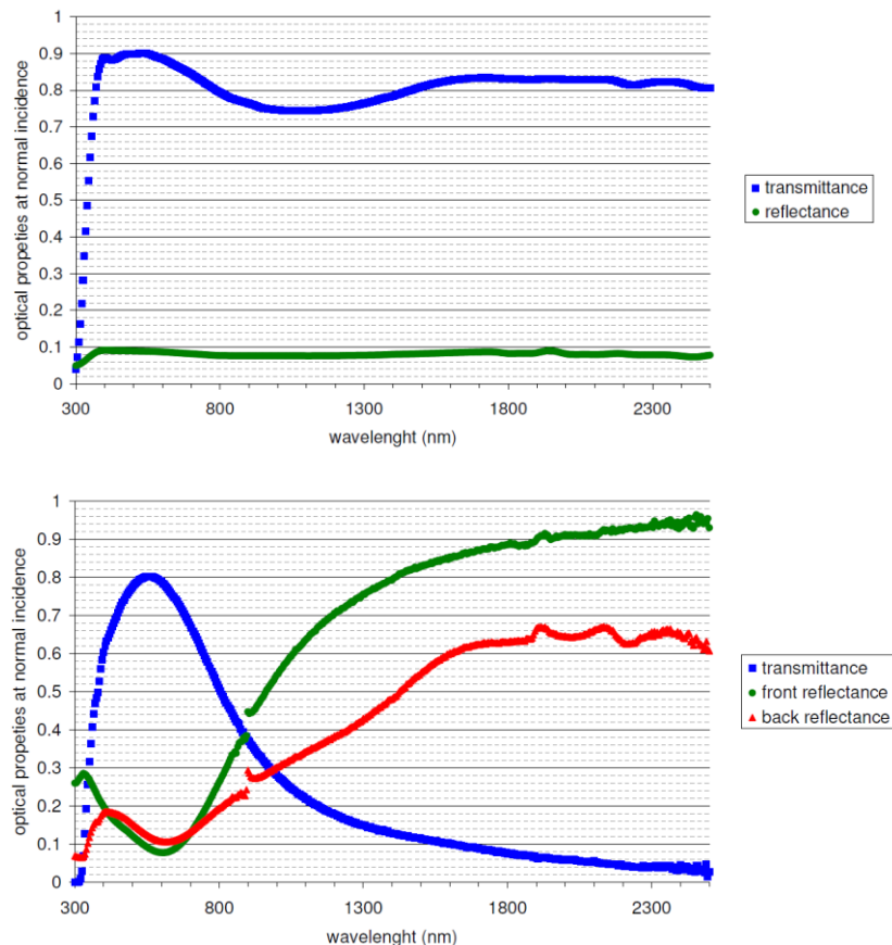
Figure 1.12 : Transmittances et réflectances à l'angle d'incidence normal ( 0^\circ ) en fonction des longueurs d'onde pour un vitrage sans traitement de 4mm (haut) et pour le même vitrage avec un traitement argent supplémentaire (bas) [Dama 2004].
