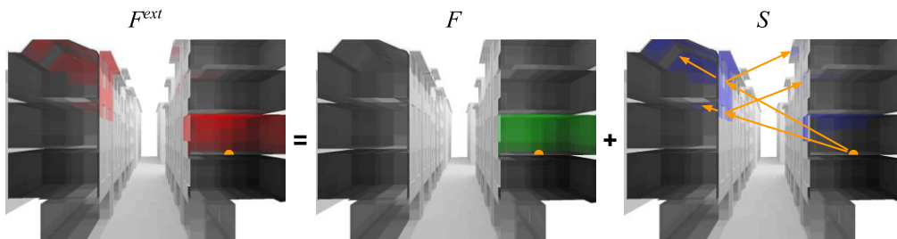
Figure 2.25 : Coupe transversale des bâtiments d'une rue de Bayonne. Le carreau marqué en jaune voit, directement ou indirectement, l'ensemble des carreaux rouges. Les carreaux vus directement (verts) et après réflexions spéculaires et transmissions directes (bleus) sont séparés dans les deux images de droite.
