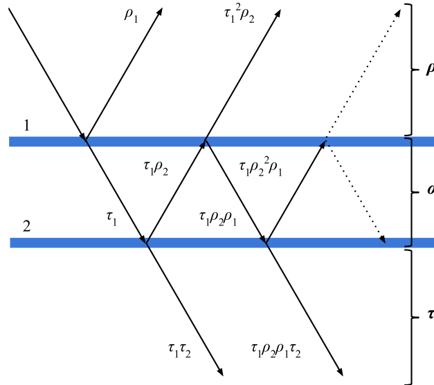
Figure 1.10 : Représentation géométrique des inter-réflexions produites à l'intérieur d'un double vitrage.
