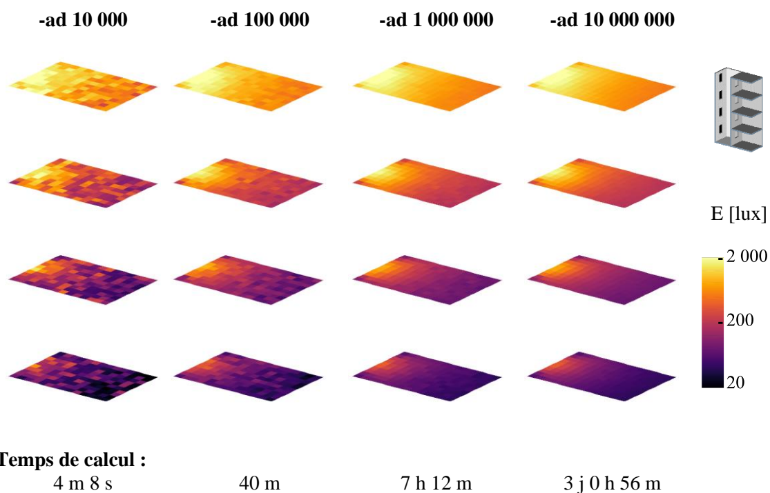
Figure 3.17 : Résultats et temps de calcul de simulations RADIANCE des éclairagements instantanés sur les quatre plans de travail avec différentes quantités de rayons émis par capteur (paramètre -ad). (30 réflexions sont prises en compte)
