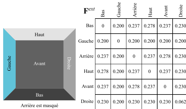
Figure 2.28 : Matrice des facteurs de vue étendus dans un cube. Toutes les surfaces sont diffuses sauf le carreau Gauche en bleu qui est un miroir.
