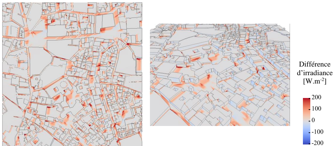
Figure 4.13 : Différences d'irradiance entre la rue normale spéculaire et normale diffuse (variante spéculaire – variante diffuse).
