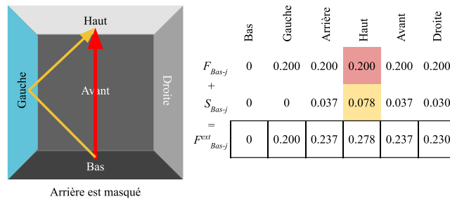
Figure 2.27 : Facteurs de vue ( F ), partie supplémentaire des facteurs de vue étendus ( S ), et facteur de vue étendu ( F^{ext} ) du carreau Bas . Le carreau bleu Gauche est un miroir.
