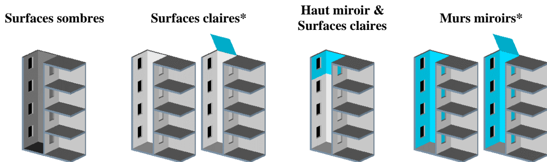
Figure 3.3 : Les 4 variantes étudiées et les 2 supplémentaires avec le dispositif de redirection. Les miroirs sont en bleu ciel.
