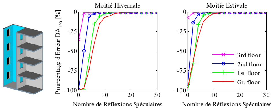
Figure 3.20 : Convergence des résultats de DA_{100} dans les 4 étages d'un puits de jour avec murs miroirs durant la moitié estivale et hivernale en fonction du nombre de réflexions spéculaires.
