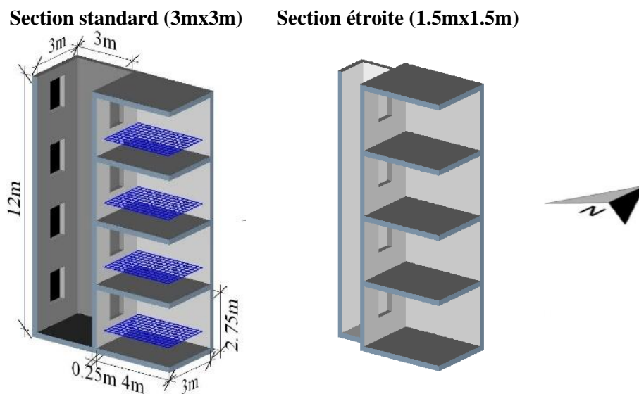
Figure 3.2 : A gauche : la géométrie du puits de jour de section 3mx3m (WI = 4) et les 4 pièces adjacentes avec leur grille de capteurs ; à droite : le puits de jour avec une section étroite de 1.5mx1.5m (WI = 8).
