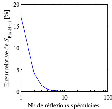
Figure 2.30 : Convergence de l'erreur relative du calcul de S_{Bas-Haut} en fonction du nombre de réflexions spéculaires prises en compte dans le cas du cube avec les deux carreaux miroirs parallèles.
