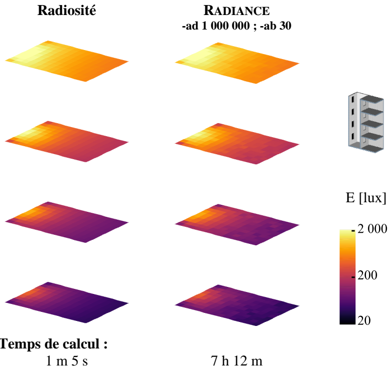
Figure 3.24 : Comparaison des temps de calcul à précision équivalente entre la méthode de radiosité développée et RADIANCE.
