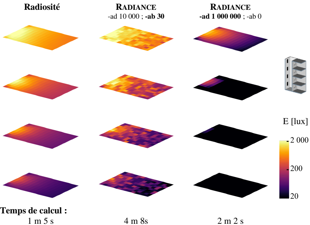
Figure 3.25 : Comparaison des résultats de la méthode de radiosité développée et de RADIANCE à temps de calcul équivalents. Deux simulations RADIANCE sont présentées : la première avec un nombre de rayons diminué, la seconde avec un nombre de réflexion diminué.
