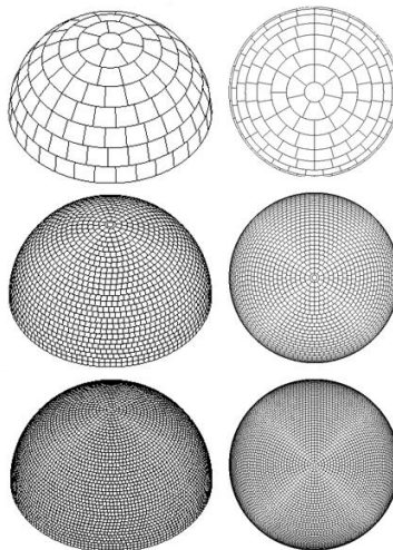
Figure 2.11 : Vues 3D et projections orthographiques de 3 partitions de l'hémisphère en 145, 2 000 et 5 000 carreaux selon [Beckers 2012].
