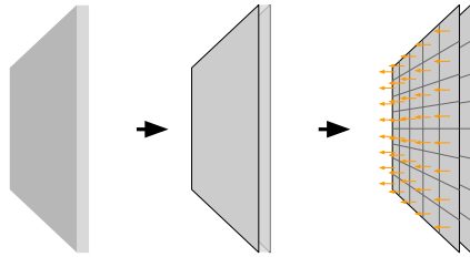
Figure 2.5 : Maillage des deux surfaces d'un même élément fin non-opaque.
