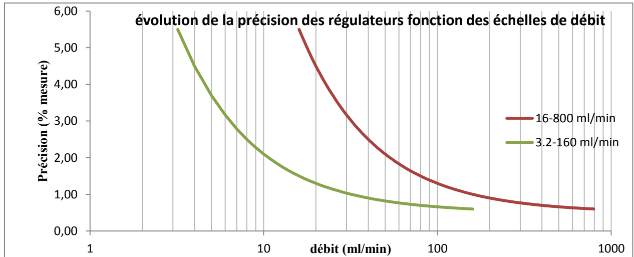
Figure III-4 : Evolution de la précision des régulateurs
