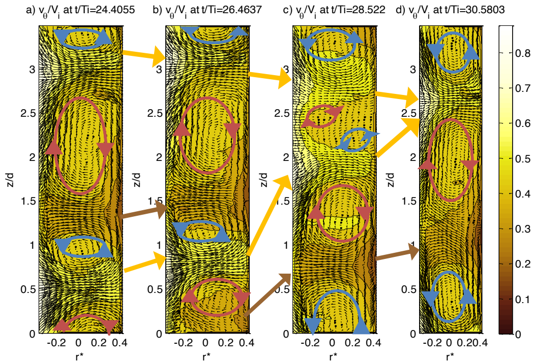
Figure VI-44 : Cartographie instantanée de la vitesse azimuthale et superposition au champ de vecteur instantané dans le plan vertical (pour les instants correspondants aux points a-b-c-d de la Figure VI-43 a) t/T_i=24,40 b) t/T_i=26,46 c) t/T_i=28,52 d) t/T_i=30,58 ( Re = 1731, Q_g = 80 \text{ ml/min} )
