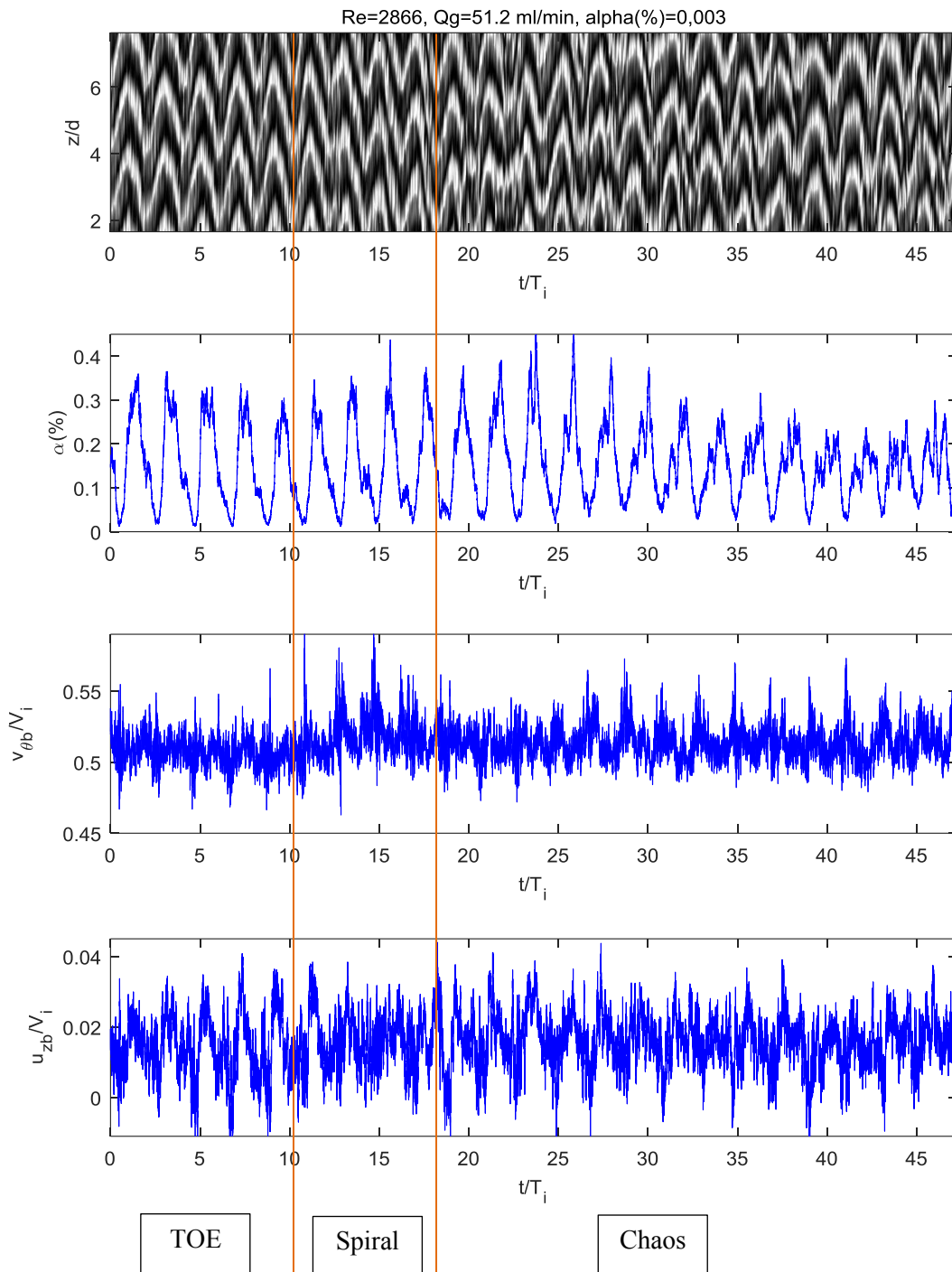
Figure VII-7 : Evolution temporelle du taux de vide instantané global et évolution temporelle des vitesses axiale et azimuthale instantanées globales en régime de coexistence structurée, pour différents motifs. Superposition avec le diagramme spatio-temporel qui permet d'identifier les motifs.
