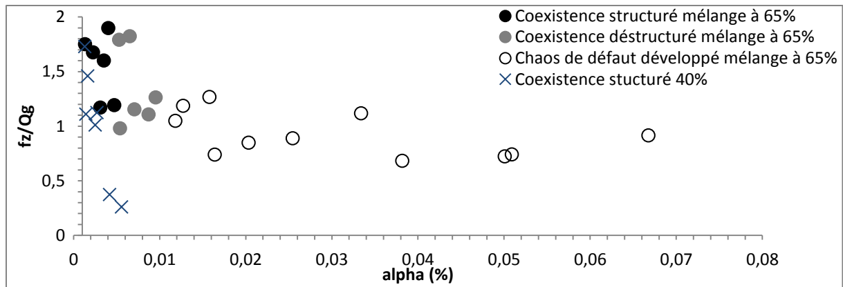
Figure VII-6 : Ratio entre le flux axial et le débit d'air imposé en fonction du paramètre alpha. Distinction des régimes.
