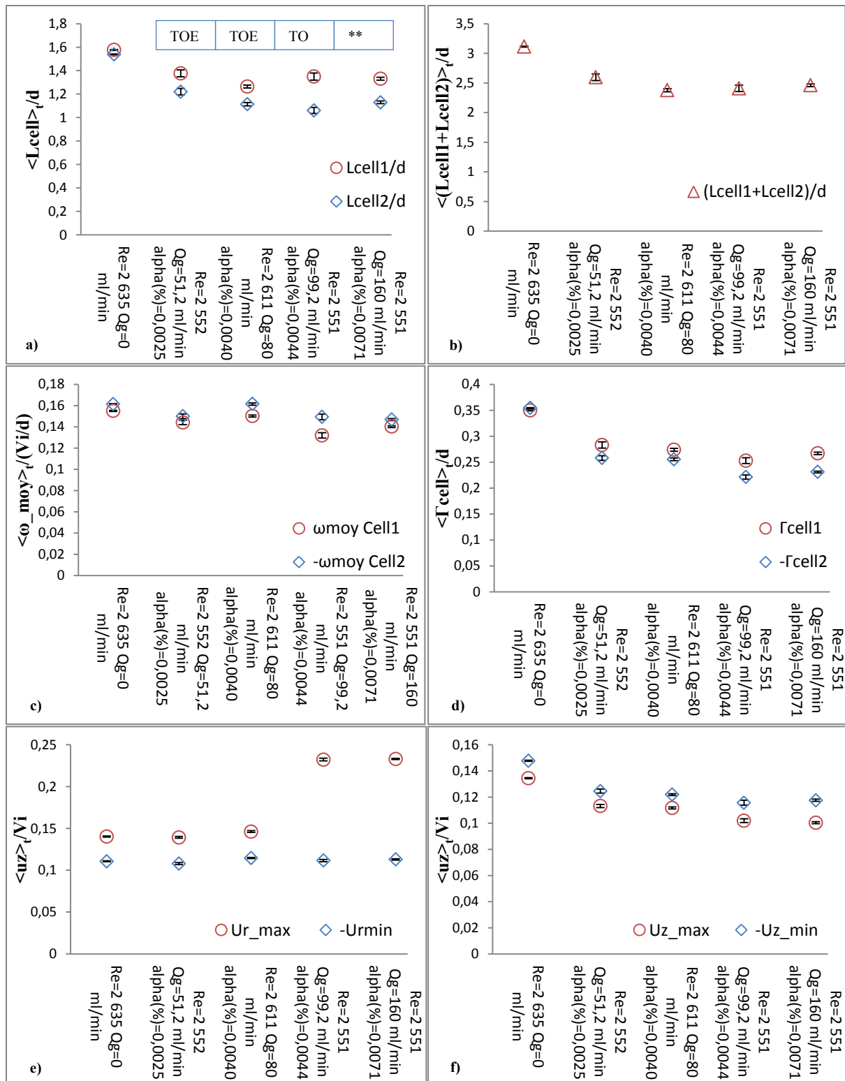
Figure Annexe H.6 : Influence du alpha sur la séquence de chaos de défauts a) taille des cellules, b) longueur d'onde axiale, c) vorticit , d) circulation, e) extrema de vitesse radiale, f) extrema de vitesse axiale adimensionnelle et moyenn  en temps
