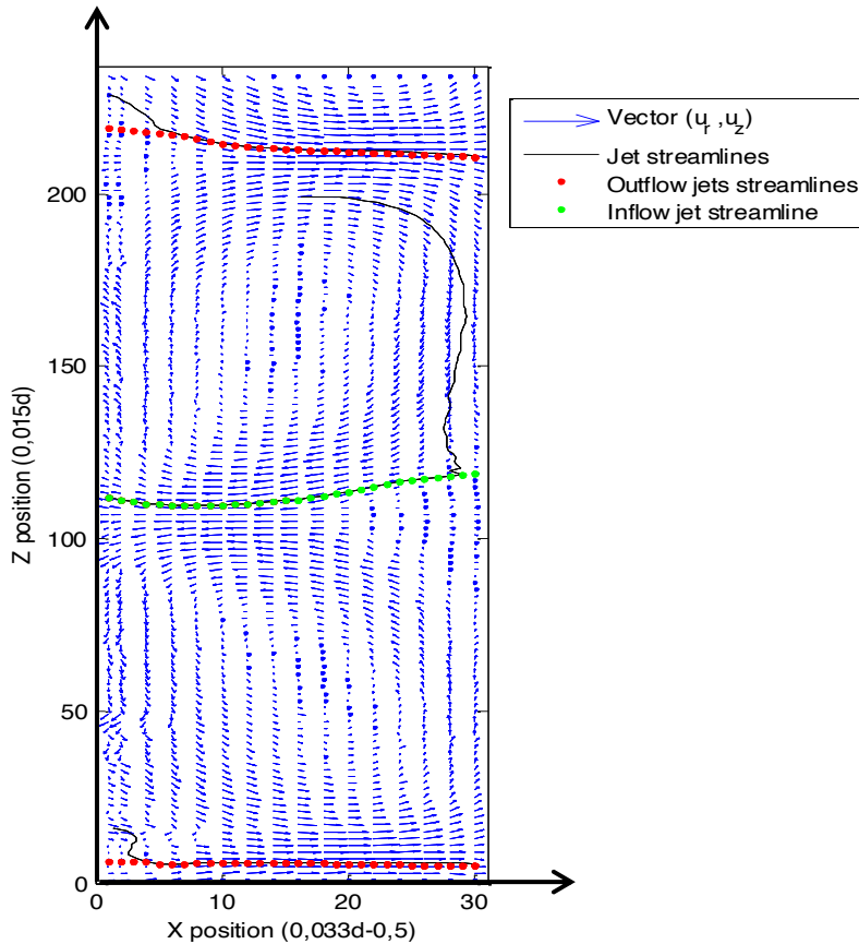
Figure IV-7 : Exemple de ligne de courants obtenus par calcul dans les zones de jets et leur extrapolation (rouge : outflow, vert : inflow). Superposition au champ de vecteur instantané (u_r, u_z) (calcul en monophasique pour Re = 2760 )
