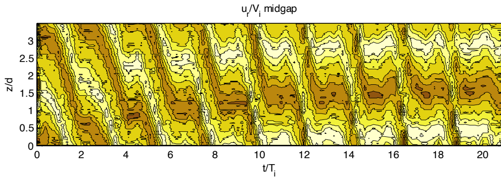
Figure VI-5 : Diagramme spatio-temporel de la vitesse radiale en milieu d'entrefer. Sélection de la séquence de motif spiral ( Re = 2551, Q_g = 51,2 \text{ ml/min}, \alpha(\%) = 0,0024 )
