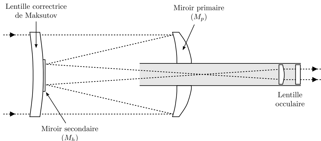
Figure 2.10: Télescope catadioptrique de type Maksutov-Cassegrain.
