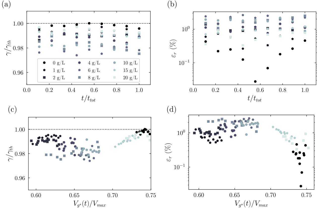
Figure 2.18: Mesure dynamique de la tension de surface \gamma et écarts relatifs \varepsilon_r , pour différentes concentrations d'éosine Y, en fonction du temps t/t_{tot} [(a) et (b)] et du volume adimensionné V_{g^*}(t)/V_{max} [(b) et (d)]. La légende en (a) est valable pour les courbes (b), (c) et (d). La ligne discontinue (.....) matérialise la tension de surface théorique de l'eau à 25°C.
