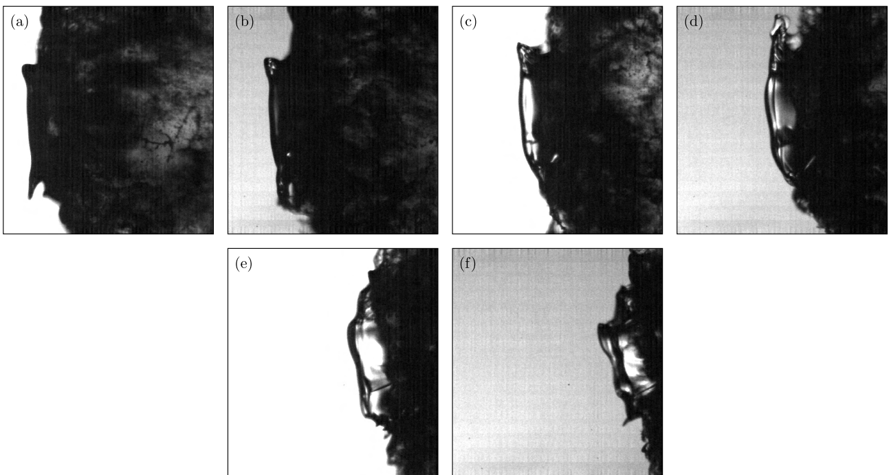
Figure 2.15: Développement d'une lèvre sur le front avant de la goutte à We=1350 . Les temps adimensionnés \tilde{t} sont (a) 1.78, (b) 1.84, (c) 1.90, (d) 1.96, (e) 2.14, (f) 2.2
