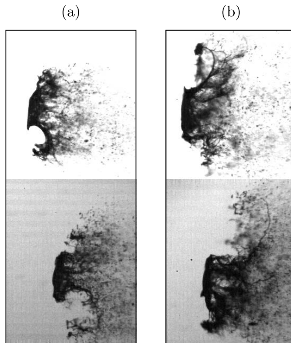
Figure 4.5: Fragmentation des ligaments. Les images du haut montrent des ligaments encore intègres et accrochés au corps de la goutte tandis que les images du bas, 25 \mu s après, montrent les ligaments fragmentés. (a) We=332 ( \tilde{t} \approx 1.4 - 1.7 ), (b) We=350 ( \tilde{t} \approx 1.4 - 1.7 ).
