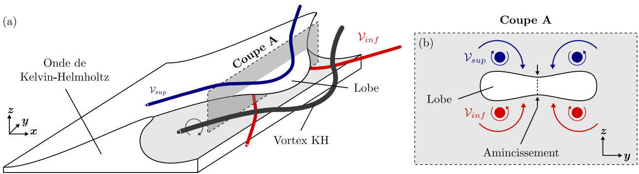
Figure 4.26: (a) Sch ma 3-D de la superposition de deux vortex en  pingle contra-rotatifs, l’un au-dessus du lobe (bleu) et l’autre en-dessous (rouge). (b) Coupe z - y (plan A) du lobe de l’onde Kelvin-Helmholtz illustrant l’action combin e des deux vortex   l’origine de l’amincissement du lobe. Les vortex sont p riodiques suivant les directions x et y . Ce sch ma s’inspire de la figure 16 de la r f rence [152].
