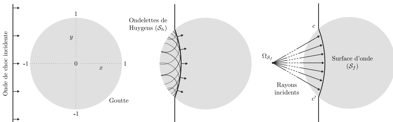
Figure 3.5: Formation d'une surface d'onde suivant le principe de Huygens.
