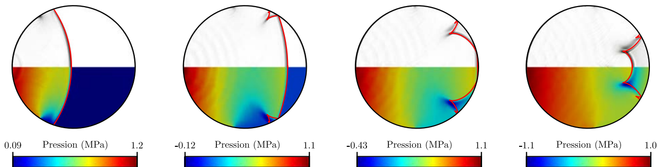
Figure 3.13: Superposition des fronts d’ondes déterminés par la théorie des rayons (rouge) et le schlieren numérique (niveaux de gris) de la simulation 2D (demi-espace supérieur de la goutte). Superposition des fronts d’onde déterminés par la théorie des rayons (rouge) et champs de pression numérique de la simulation 2D (demi-espace inférieur de la goutte). Ces résultats correspondent à l’interaction d’une onde de choc à Ms = 2 avec une goutte d’eau ( R_0 = 1 mm). Les temps \tilde{t} , de gauche à droite, sont respectivement 0.52, 0.89, 1.04 et 1.18.
