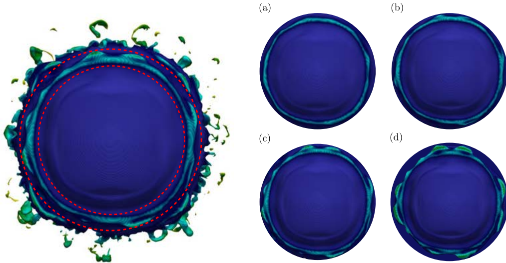
Figure 4.25: Développement de perturbations azimutale transverse pour We = 470 (vue de face). Les temps caractéristiques \hat{t} sont (a) 0.79, (b) 0.82, (c) 0.84 et (d) 0.86. Les images (a)-(d) sont des coupes.
