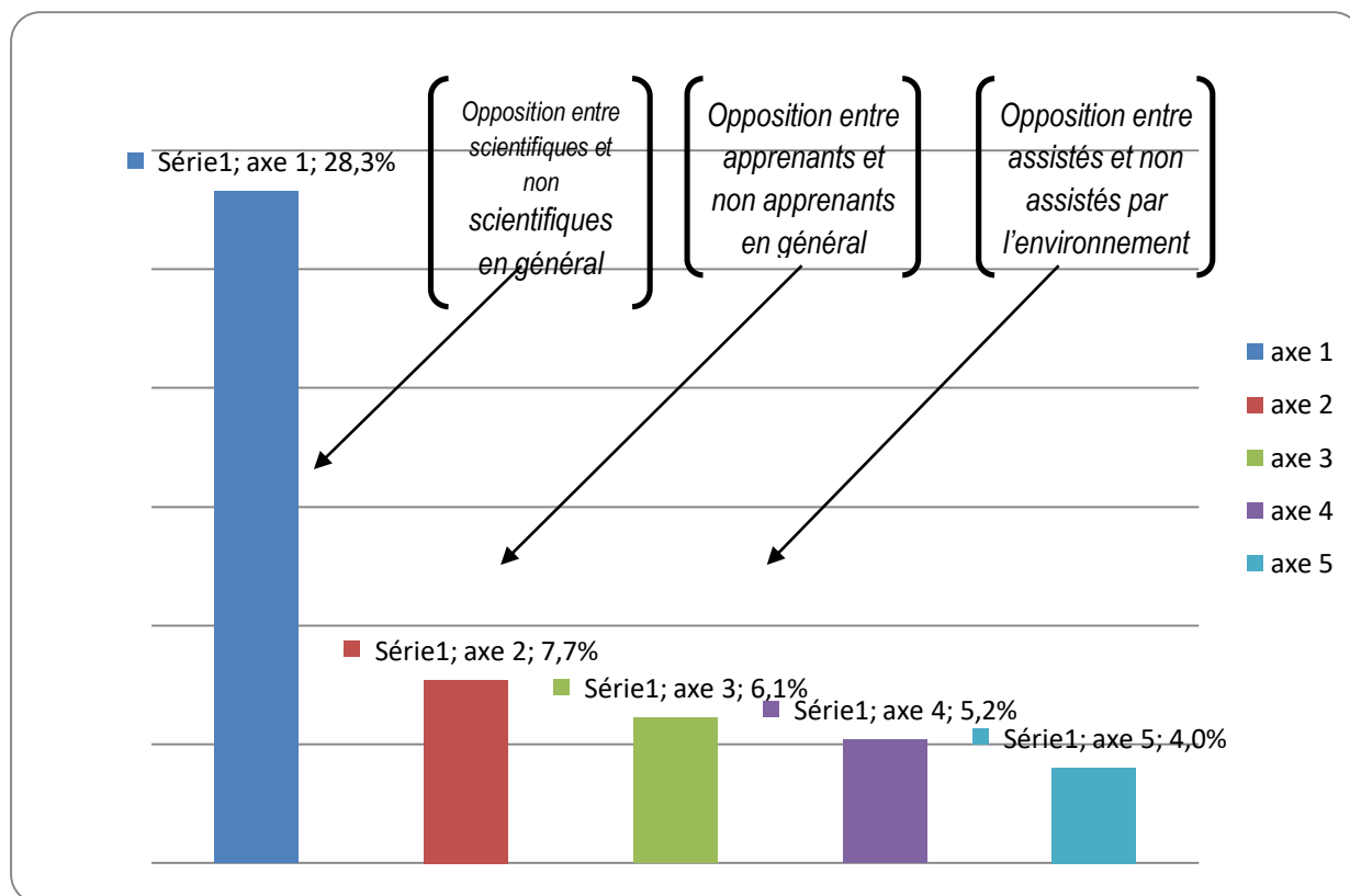
Figure 35: Histogramme des premières valeurs propres, donnant le pourcentage d'informations expliquées par axe.
