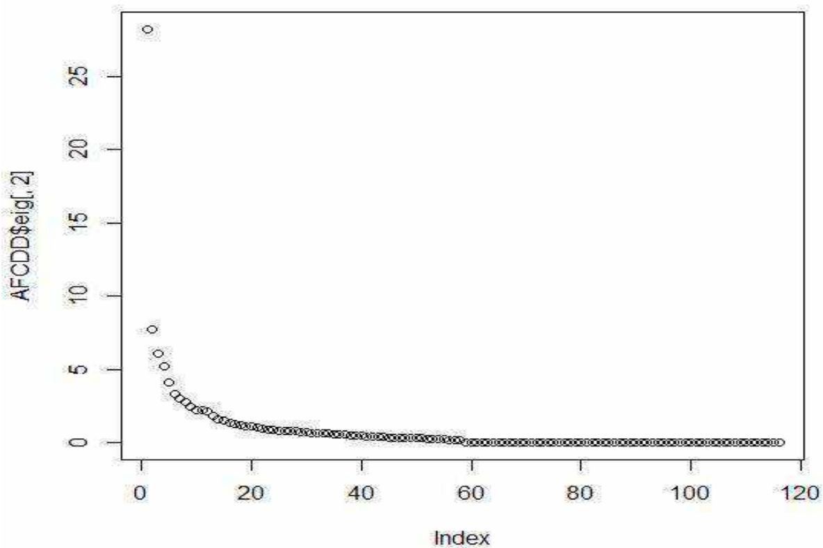
Figure 18 : Graphique de l'histogramme des valeurs propres et l'importance des plans factoriels
