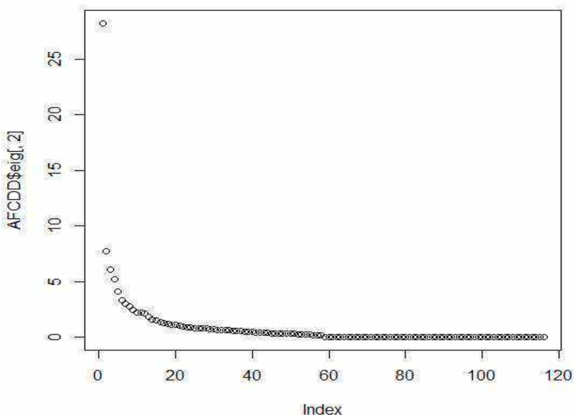
Graphe 6: l'histogramme des valeurs propres
