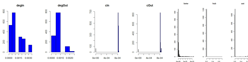
FIGURE 6.7 – Distributions des 7 centralités sur le réseau AAD_APA_ARE.
