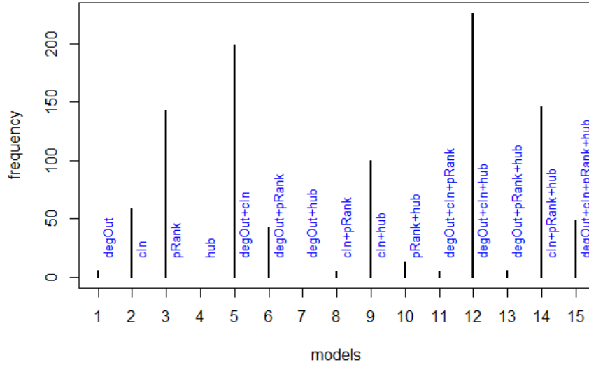
FIGURE 5.5 – Choix du meilleur modèle logistique par 1000 itérations de Bootstrap
