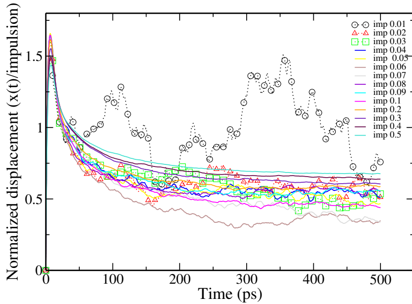
FIGURE A.6 – Déplacements moyens normalisés \langle x_u \rangle(t) / V_0 pour un ensemble de vitesses croissantes allant de 0,01 à 0,09 nm.ps -1 et de 0,10.5 nm.ps -1 .
