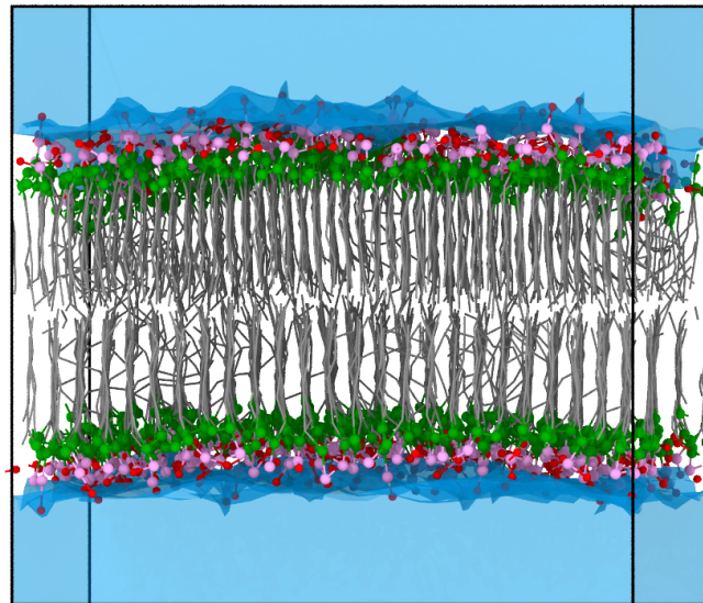
FIGURE A.8 – Snapshot d'une configuration à basse température (280 K).
