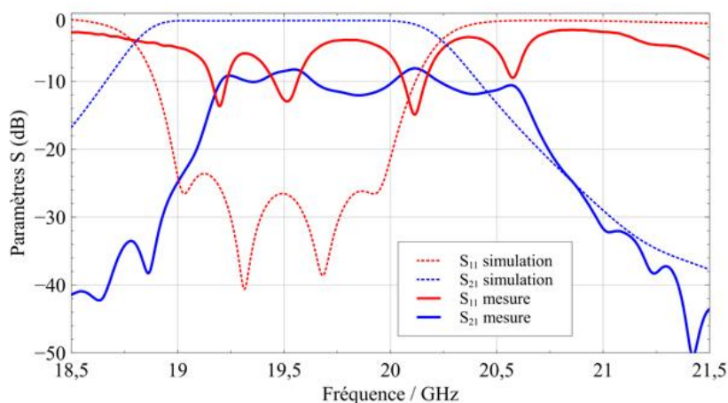
Figure 105 : à droite, visualisation du filtre en cordiérite avant métallisation, puis vue du prototype complet, à gauche comparaison de la mesure avec la simulation
