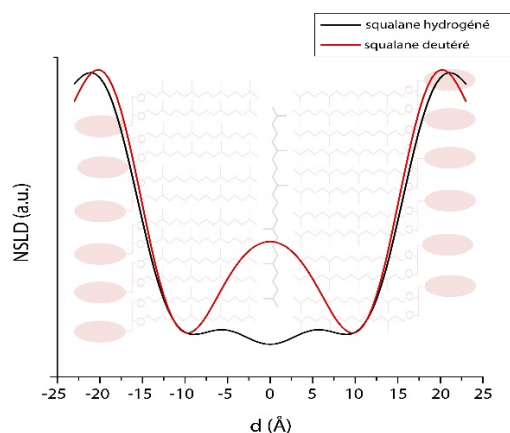
Figure 3. Profile de densité neutronique de DoPhPC: DoPhPE (9:1) en présence de squalane hydrogéné (noir) et deutéré (rouge). d représente l'épaisseur de la bicouche lipidique, étant d = 0 Å son centre.
