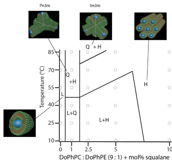
Figure 4. Diagramme de phases de DoPhPC : DoPhPE (9 : 1) avec différents pourcentages de squalane. Les phases représentées sont L : lamellaire, Q : cubique et H : hexagonale. Les cercles gris représentent les conditions mesurées. Les têtes polaires sont représentées en vert et les chaînes hydrophobes en marron, l'eau est représentée par les sphères bleues.
