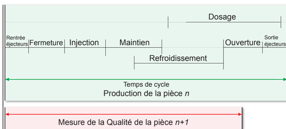
Figure 1.10 – Intégration de la mesure dans le cycle d’injection-moulage.
