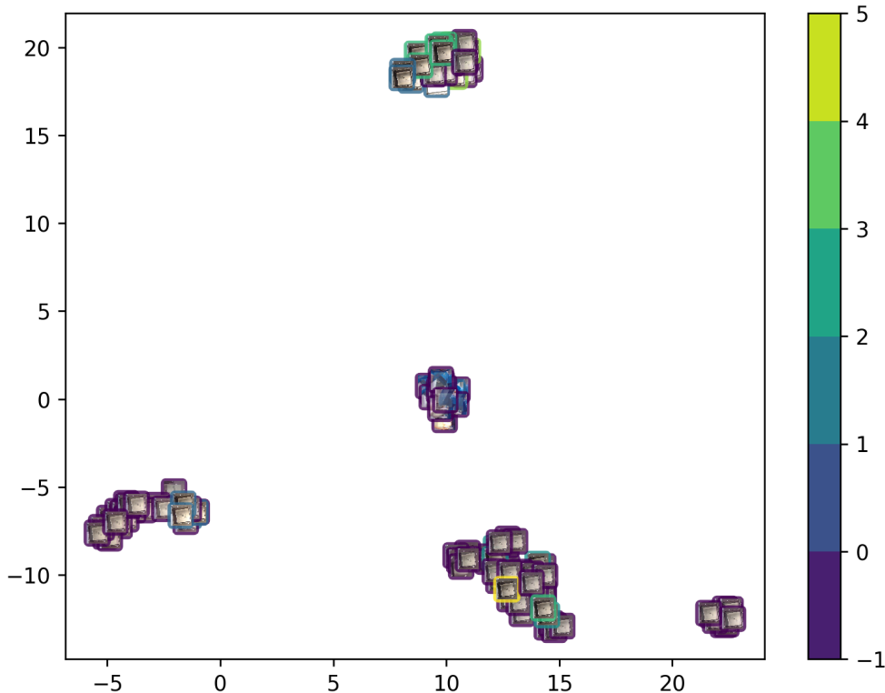
Figure 3.6 – Projection par t-SNE à partir des valeurs de la dernière couche d'un réseau de triplets. L'échelle 1-5 correspond aux niveaux de qualité évalués par les experts humains; -1 correspond aux pièces non annotées.
