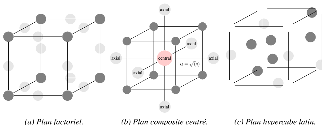
Figure D.1 – Essais prévus pour des plans d'expériences à trois niveaux pour trois variables.
