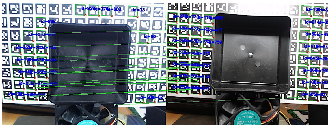
Figure 2.11 – Détection et association de marqueurs ChAruco entre deux caméras.
