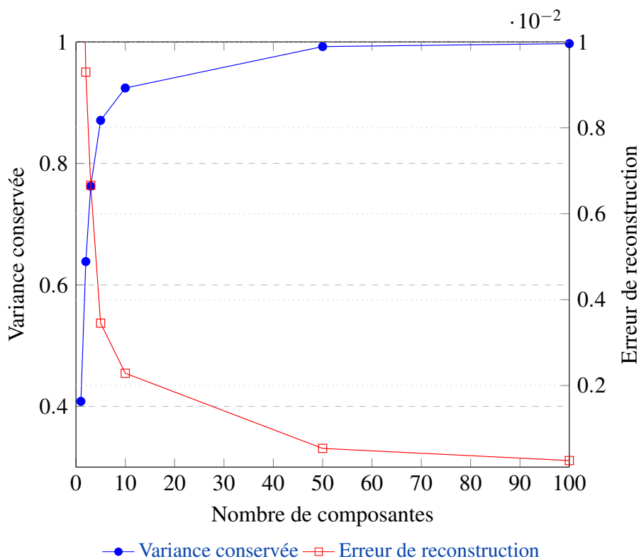
Figure 3.9 – Qualité de la compression par ACP en fonction du nombre de composantes.
