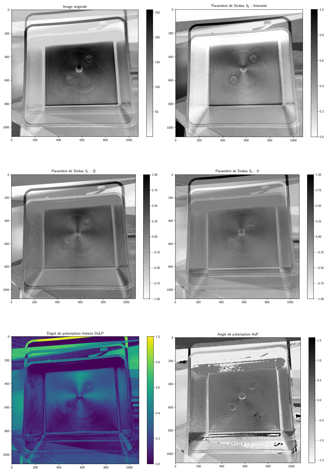
Figure 2.13 – Reconstruction des paramètres de Stokes partiels, du Degré et de l'Angle de Polarisation, à partir des images de 3 caméras.
