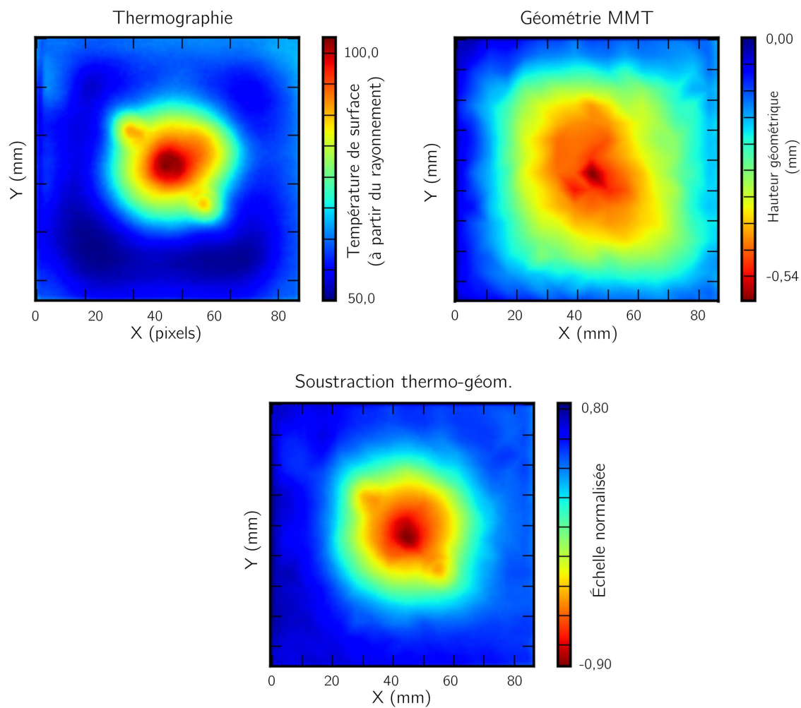
Figure 2.4 – Mesure thermique et mesure géométrique d'une pièce thermo-moulée.
