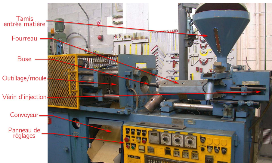
Figure 1.1 – Une presse à injecter. Photographie originale de Glenn McKechnie © by SA 2.5, Wikimedia Commons .
