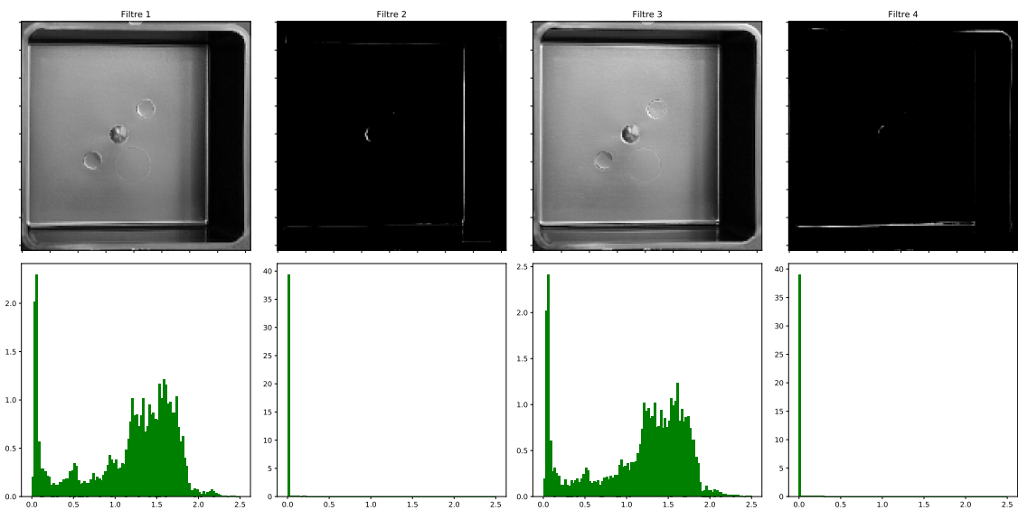
(c) Sorties avec max pooling.
