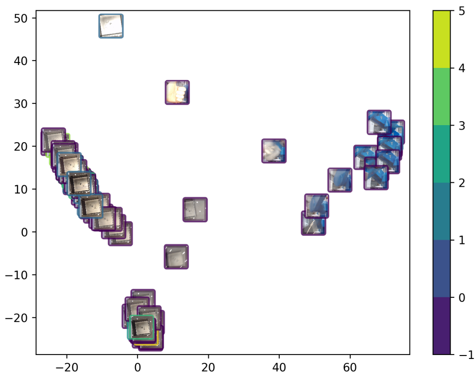
Figure 3.10 – Projection par ACP à partir de la valeur des pixels des images. L'échelle 1-5 correspond aux niveaux de qualité évalués par les experts humains; -1 correspond aux pièces non annotées.
