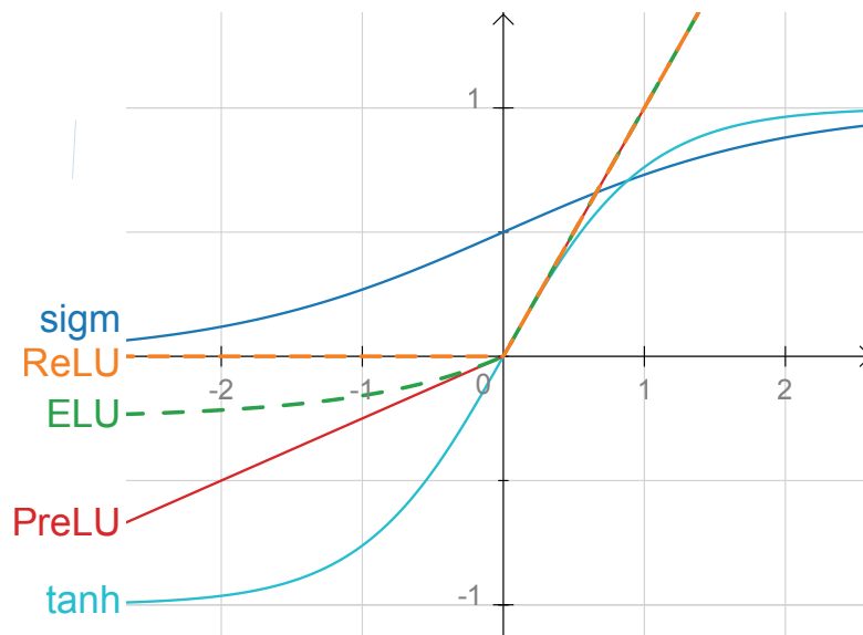
Figure F.2 – Fonctions d’activation.
