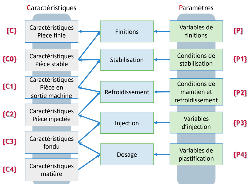
Figure 1.7 – Représentation Zig Zag du procédé d'injection-moulage des thermoplastiques.
