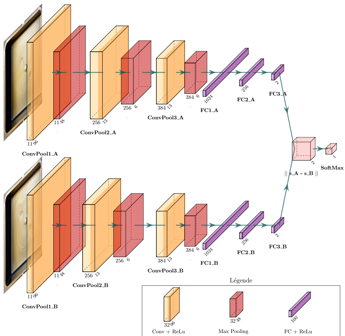
Figure 3.3 – Architecture d'un réseau siamois.
