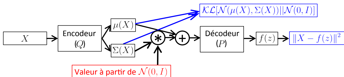
Figure 3.19 – Graphe d'un auto-encodeur variationnel, inspiré de [Doe16].
