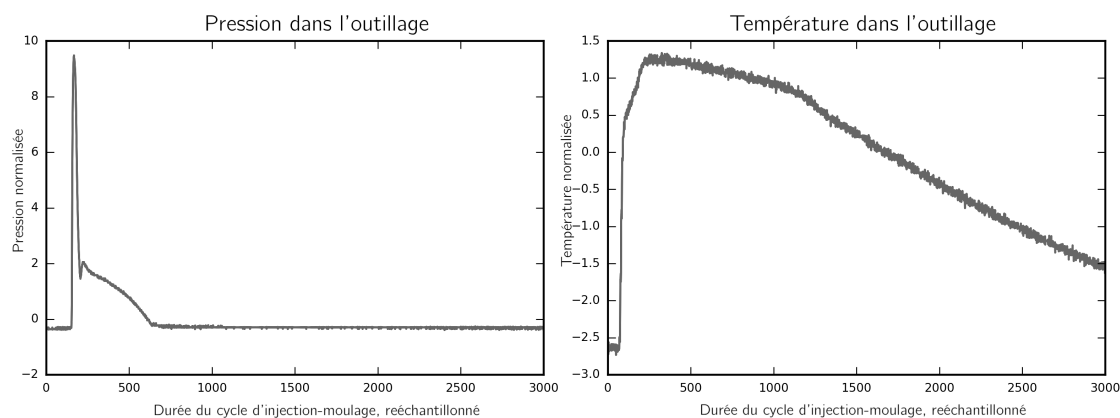
Figure 1.8 – Résultats de mesure de la pression et la température dans l'outillage pendant tout le cycle.
