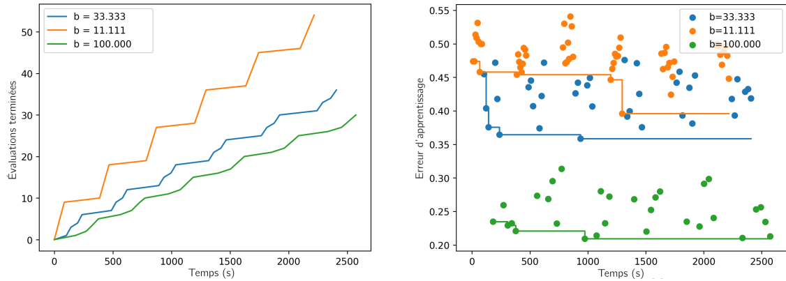
(a) Nombre d'évaluations de f réalisées en fonction de la limite de temps b .
