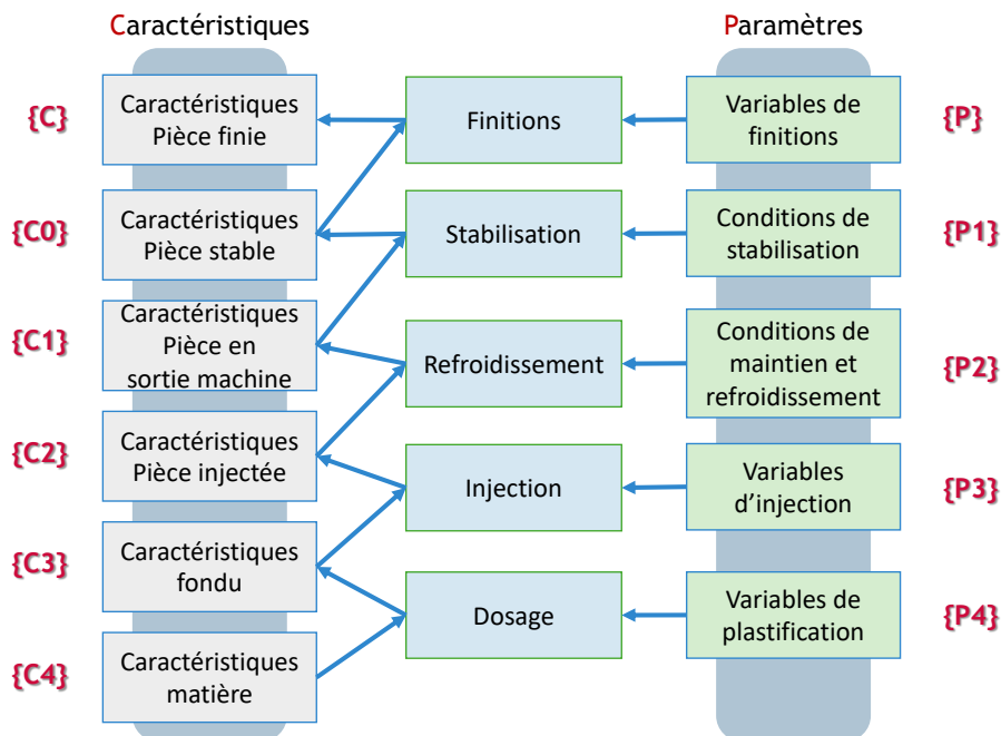
Figure A.1 – Représentation Zig Zag du procédé d'injection-moulage des thermoplastiques.
