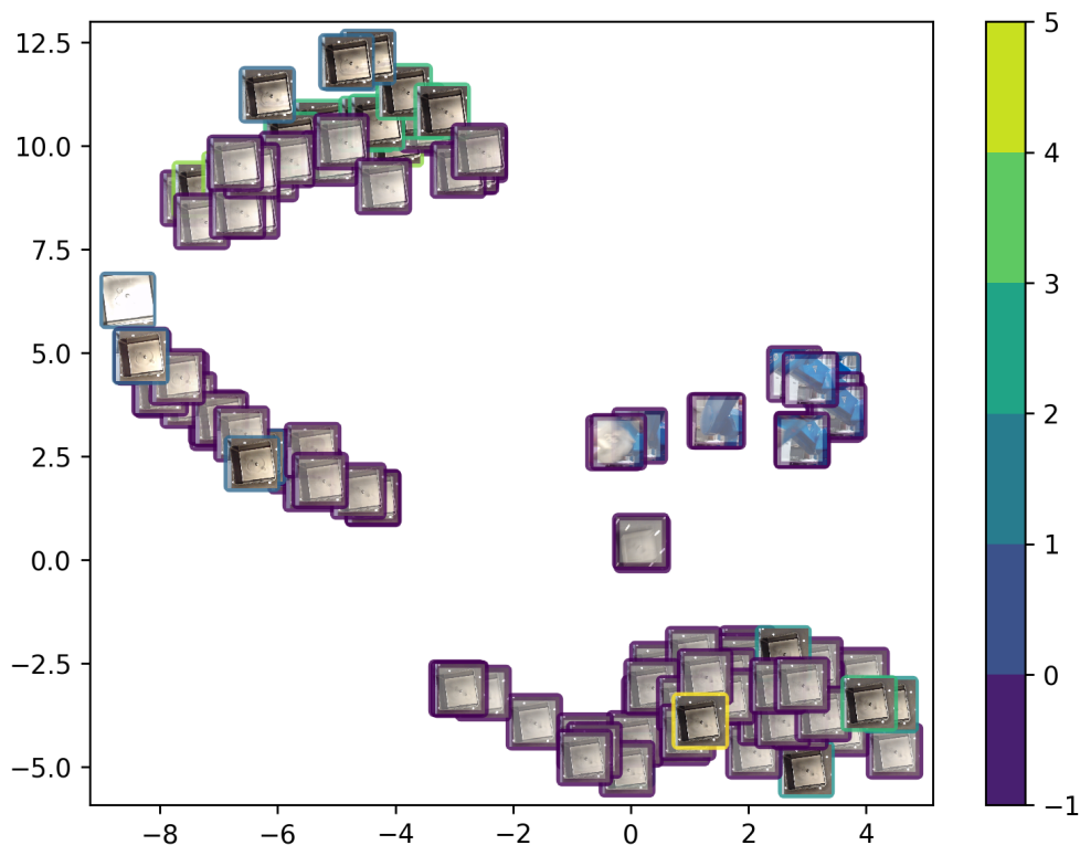
Figure 3.18 – Projection par t -SNE à partir des valeurs de l'espace latent z d'un VAE. L'échelle 1-5 correspond aux niveaux de qualité évalués par les experts humains; -1 correspond aux pièces non annotées.
