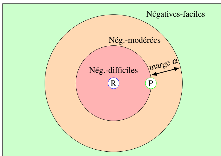
Figure 3.4 – Trois différents types d’images Négatives possibles pour un couple d’images (Référence, Positive)
