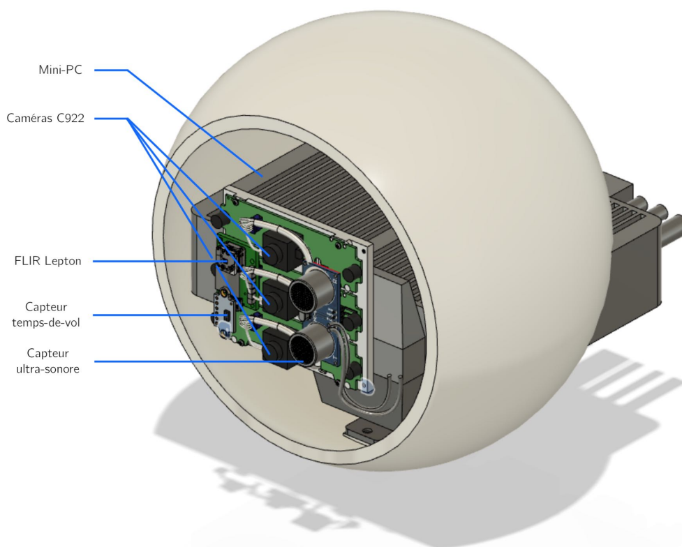
Figure 4.2 – Intégration des capteurs.
