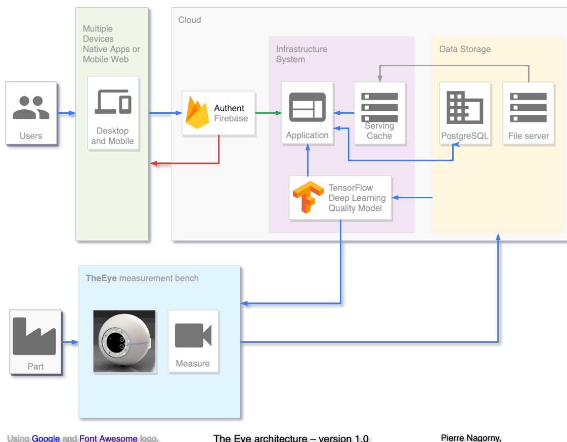
Figure 4.4 – Architecture logicielle du système proposé.
