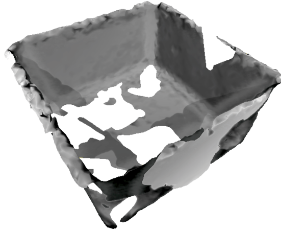
Figure 1.13 – Nuage de points de la pièce obtenue en cycle industriel avec le HandyScan.
