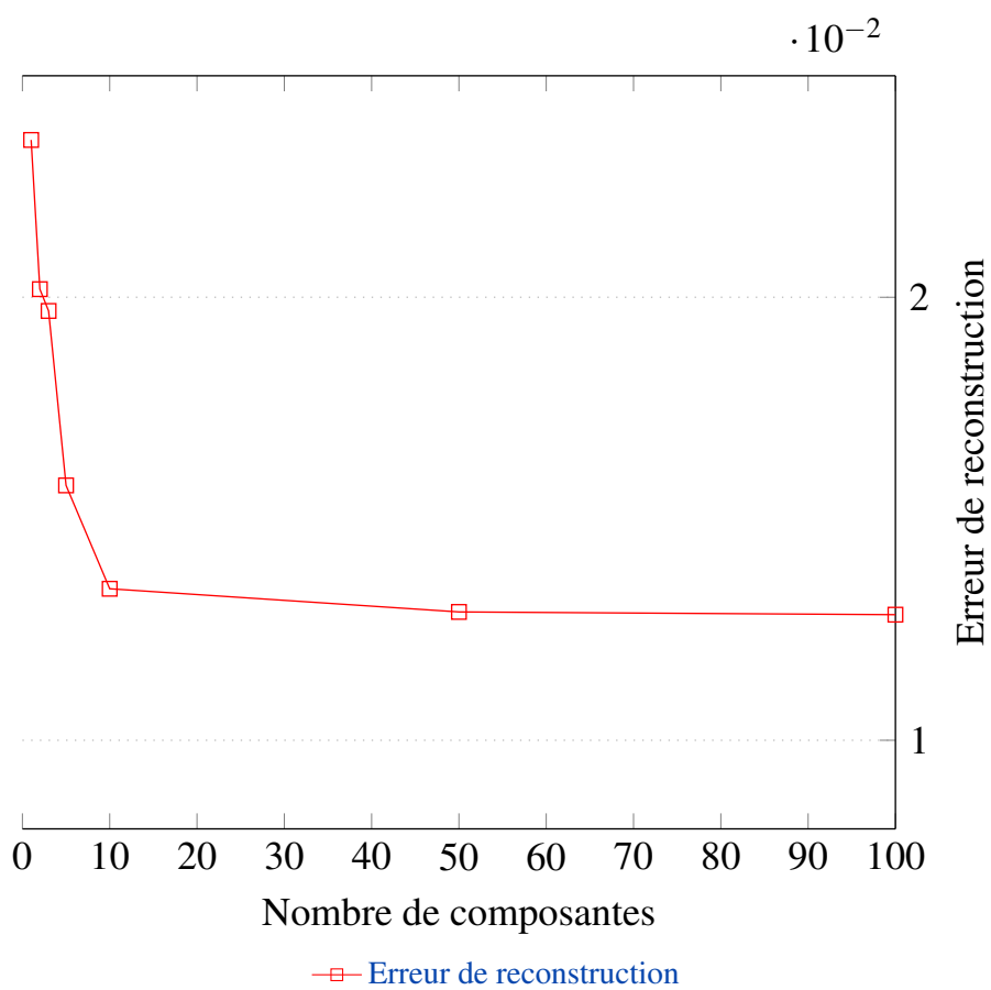
Figure 3.13 – Qualité de la compression par ACP à noyau en fonction du nombre de composantes.
