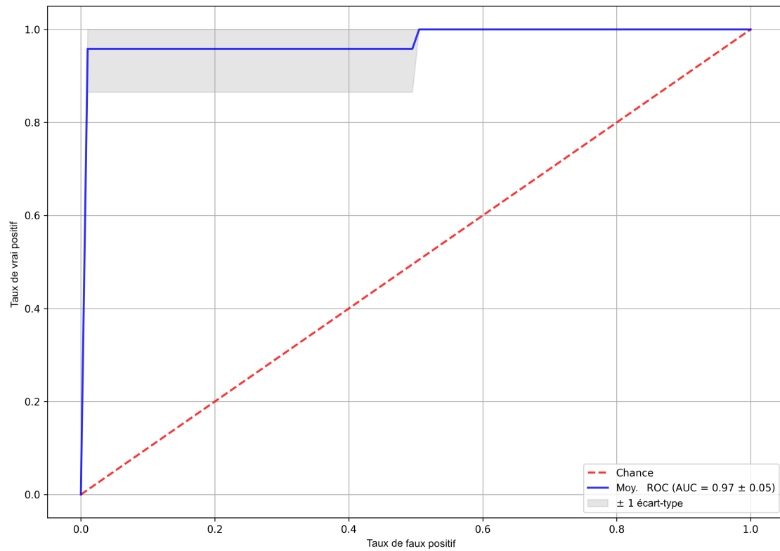
Figure 4.9 – Courbe ROC du meilleur classifieur de la qualité des pièces pour l'essai "boîtes noires".
