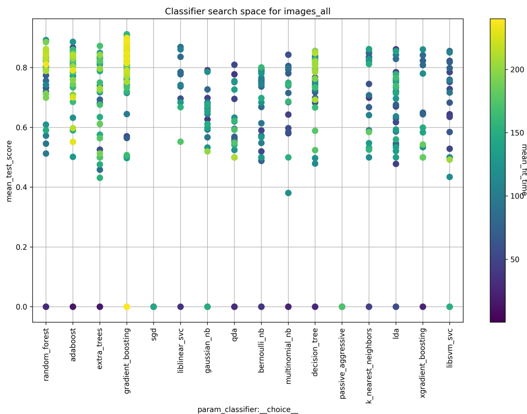
Figure 3.23 – Optimisation d’un modèle appris de manière supervisée, à l’aide de la librairie auto-sklearn [Feu+15].
