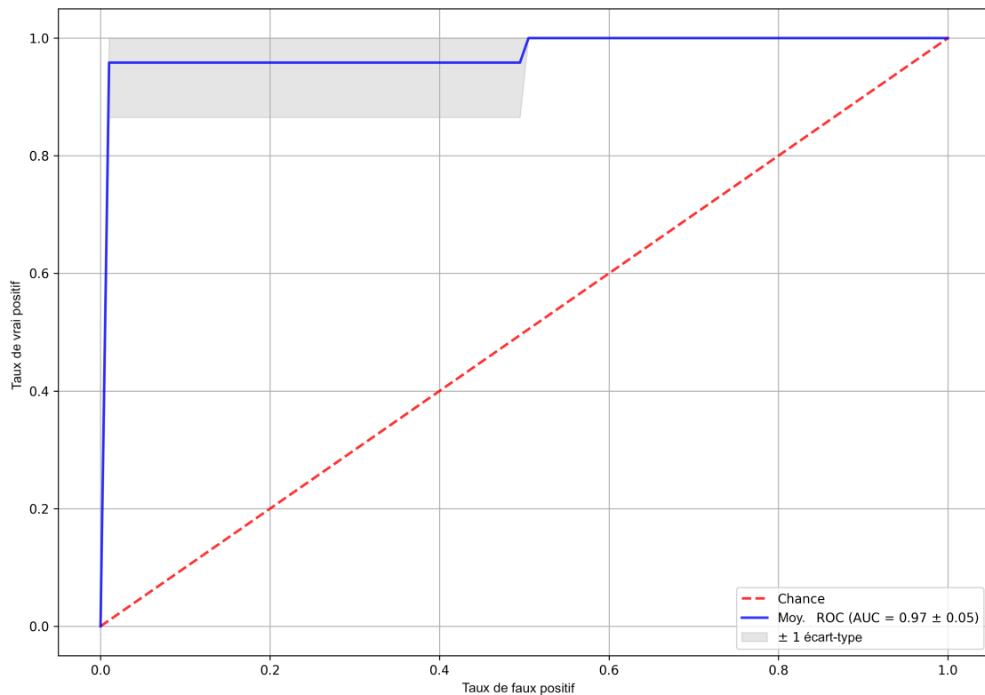
Figure E.1 – Courbe ROC du meilleur classifieur de la qualité des pièces.
