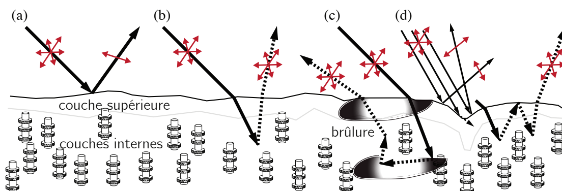
Figure 2.8 – Différentes composantes de réflexion d'un polymère semi-cristallin. (a) réflexion spéculaire, (b) réflexion diffuse, (c) réflexion diffuse sur un défaut structurel du matériau, (d) réflexion spéculaire sur un défaut de forme géométrique. Figure inspirée de [Deb+00]. .
