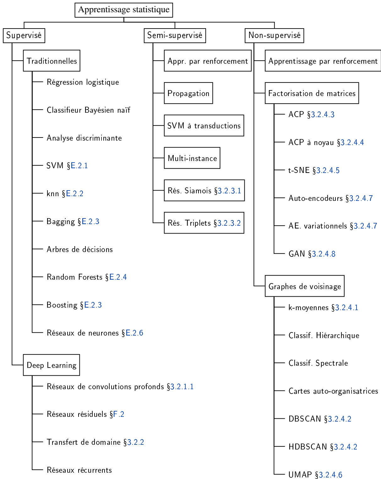
Figure 3.26 – Taxonomie de l'apprentissage statistique.
