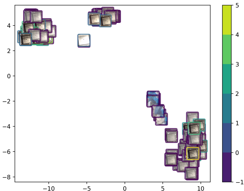
Figure 3.14 – Projection par t -SNE à partir de la valeur des pixels des images. L'échelle 1-5 correspond aux niveaux de qualité évalués par les experts humains ; -1 correspond aux pièces non annotées.
