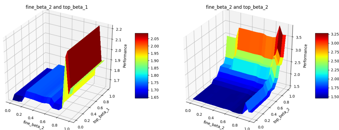
Figure 3.25 – f ANOVA des hyper-paramètres suite à l'optimisation avec BOHB.
