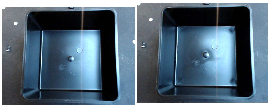
(b) Image d'une pièce non-conforme à cause d'une retassure.
