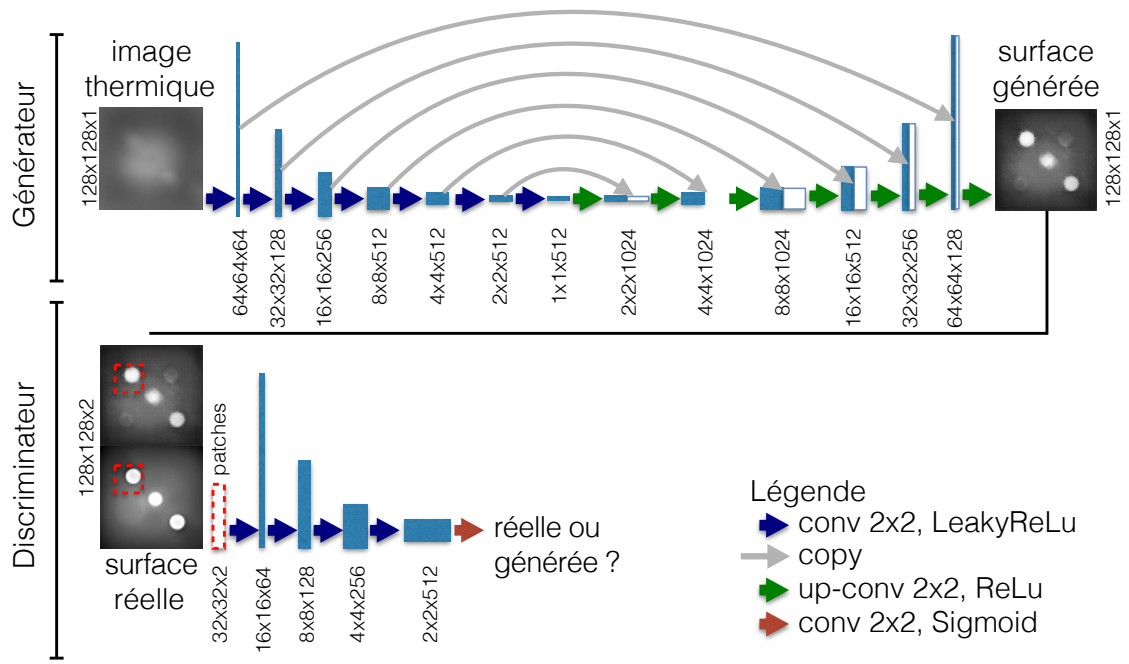
Figure 2.5 – Architecture du réseau antagoniste génératif U-Net, utilisée par le modèle pix2pix.
