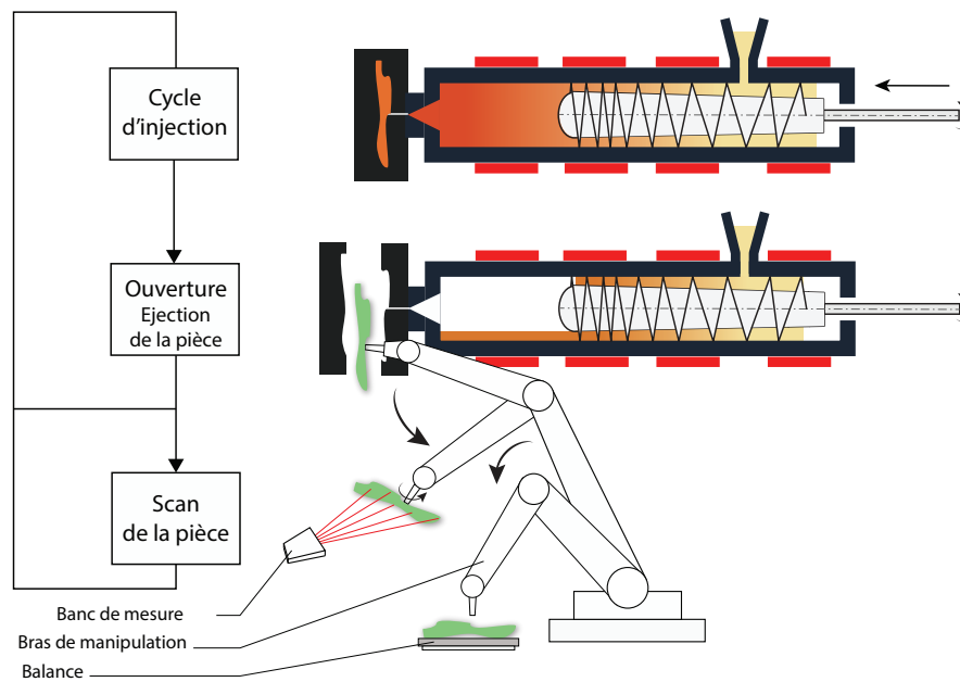
Figure 1.12 – Mesure de la géométrie d'un objet par triangulation laser en cycle industriel.
