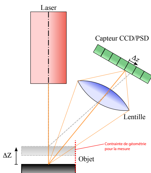
Figure 1.11 – Mesure de la géométrie d'un objet par triangulation laser. Figure dérivée du travail original de Georg Wiora (Dr. Schorsch), CC BY-SA 3.0, via Wikimedia Commons.
