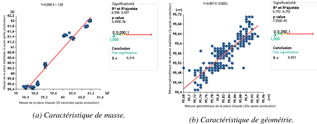
Figure 2.2 – Modèle linéaire entre les caractéristiques des pièces chaudes (30 secondes après production) et des pièces stabilisées (3 jours après production), Logiciel Ellistat 1 .
