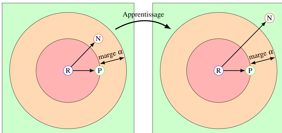
Figure 3.5 – Principe de l’apprentissage d’un réseau de triplets.
