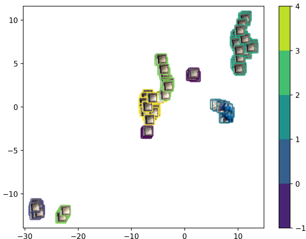
Figure 3.7 – Projection par UMAP à partir de la valeur des pixels des images. L'échelle -1 à 4 correspond aux clusters obtenus par HDBSCAN.
