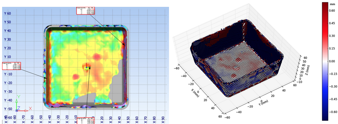
(a) Interpolation du nuage de points à l’aide du logiciel PowerInspect2017 de Autodesk. (b) Interprétation de l’écart des points de mesures à l’aide de la librairie Python Matplotlib [Hun07; Cas+19].
