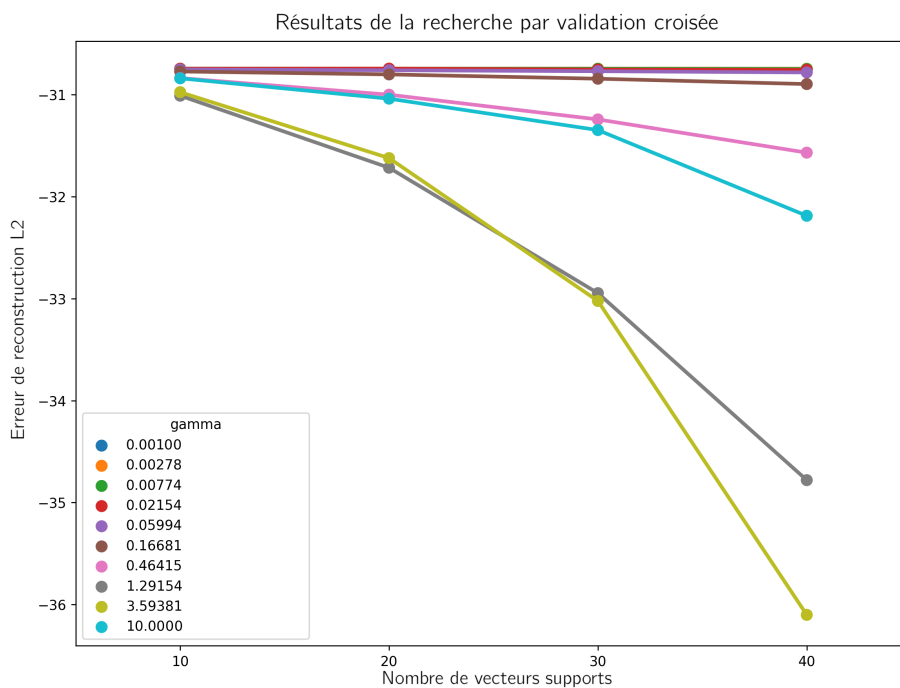
Figure 3.11 – Optimisation des paramètres d’une ACP à noyaux. Métrique : Norme \ell_2 .
