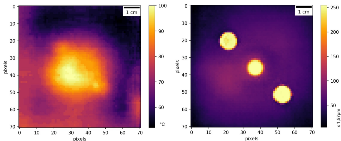
(a) Image thermique de la pièce 10s après prod. (b) Image de l'altitude de la surface de la pièce.
