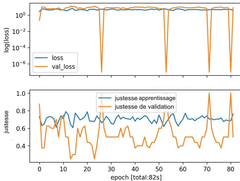
(b) Apprentissage de spécialisation de l'ensemble des poids du réseau.
