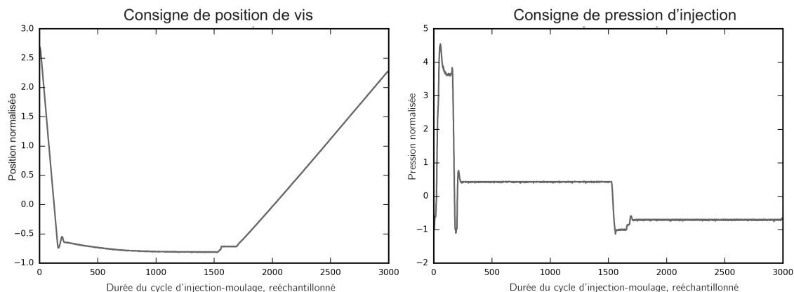
Figure 1.3 – Profil de position de la vis et de pression d'injection pendant un cycle d'injection-moulage.
