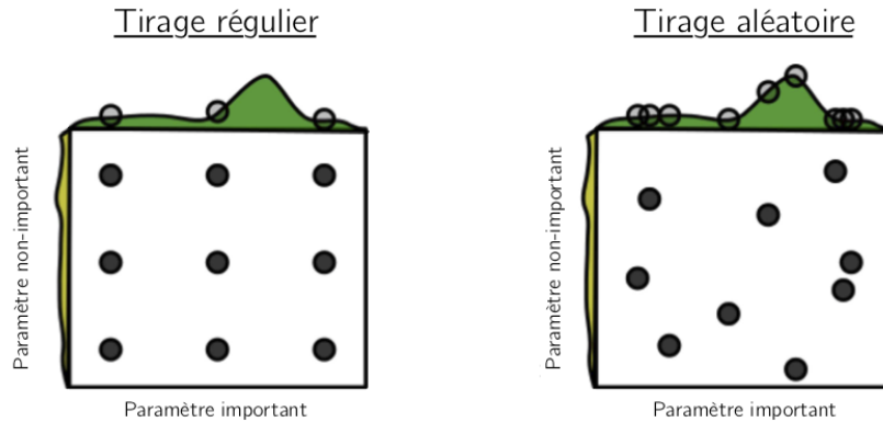
Figure 3.22 – Optimisation d'une fonction à deux variables avec neuf essais. Figure reproduite de [BB12].
