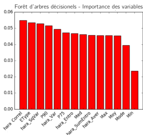
Figure 2.18 – Importance des descripteurs par Forêt d'arbres décisionnels.
