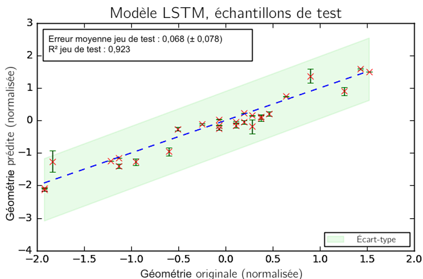
Figure 1.9 – Résultats du modèle LSTM sur le jeu de données de test.
