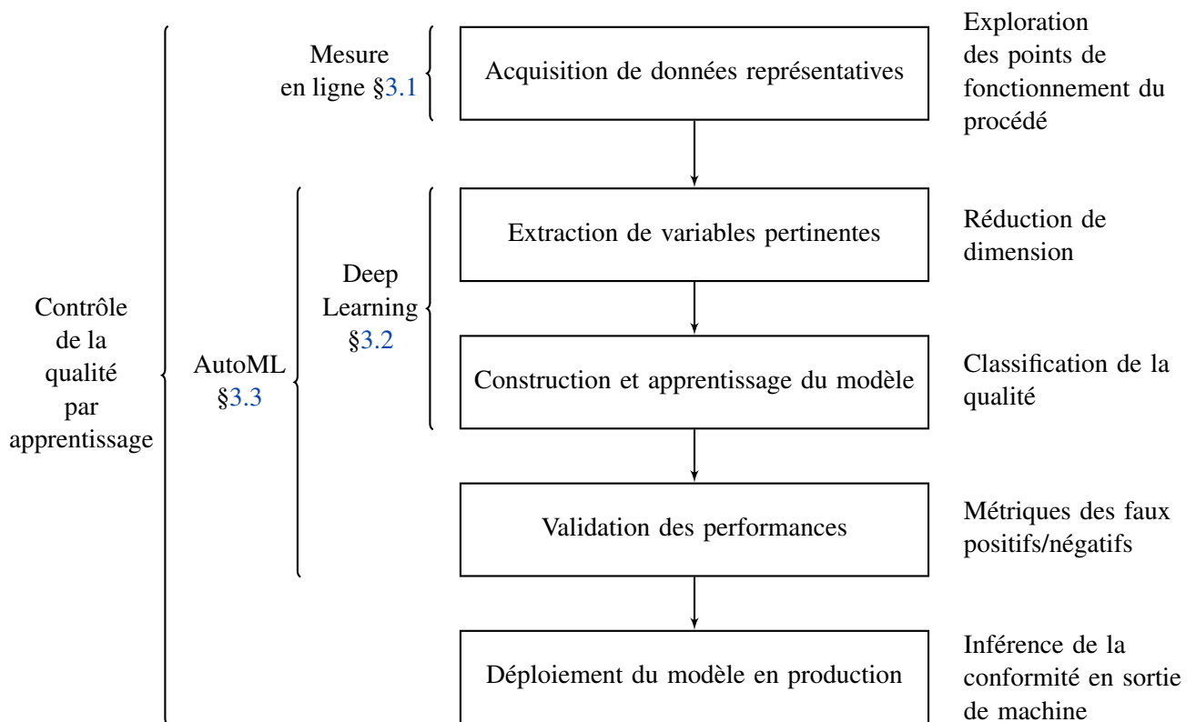
Figure 3.1 – Diagramme du processus de construction d'un algorithme de contrôle de la qualité par apprentissage.
