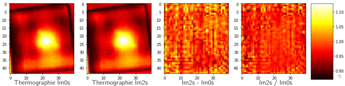
Figure 2.19 – Mesure par caméra thermique de l'évolution sur 2 secondes de la température d'une pièce.
