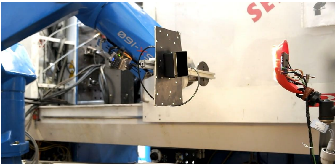
Figure 4.3 – Photographie de la présentation, par le bras robot, d'une pièce devant le prototype du dispositif de mesure, lors de l'essai §4.2.1.
