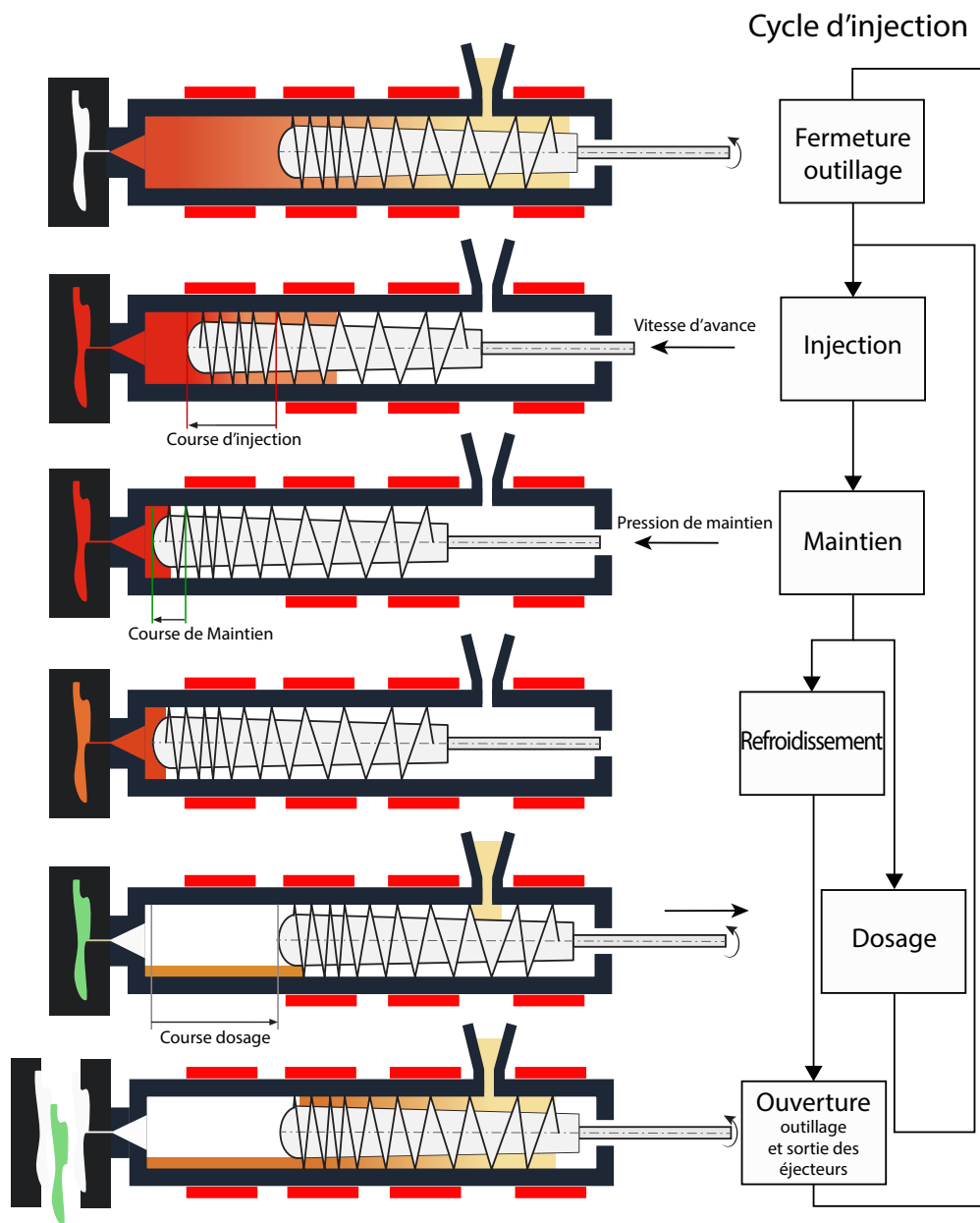
Figure 1.2 – Schéma-bloc du procédé d'injection-moulage.
