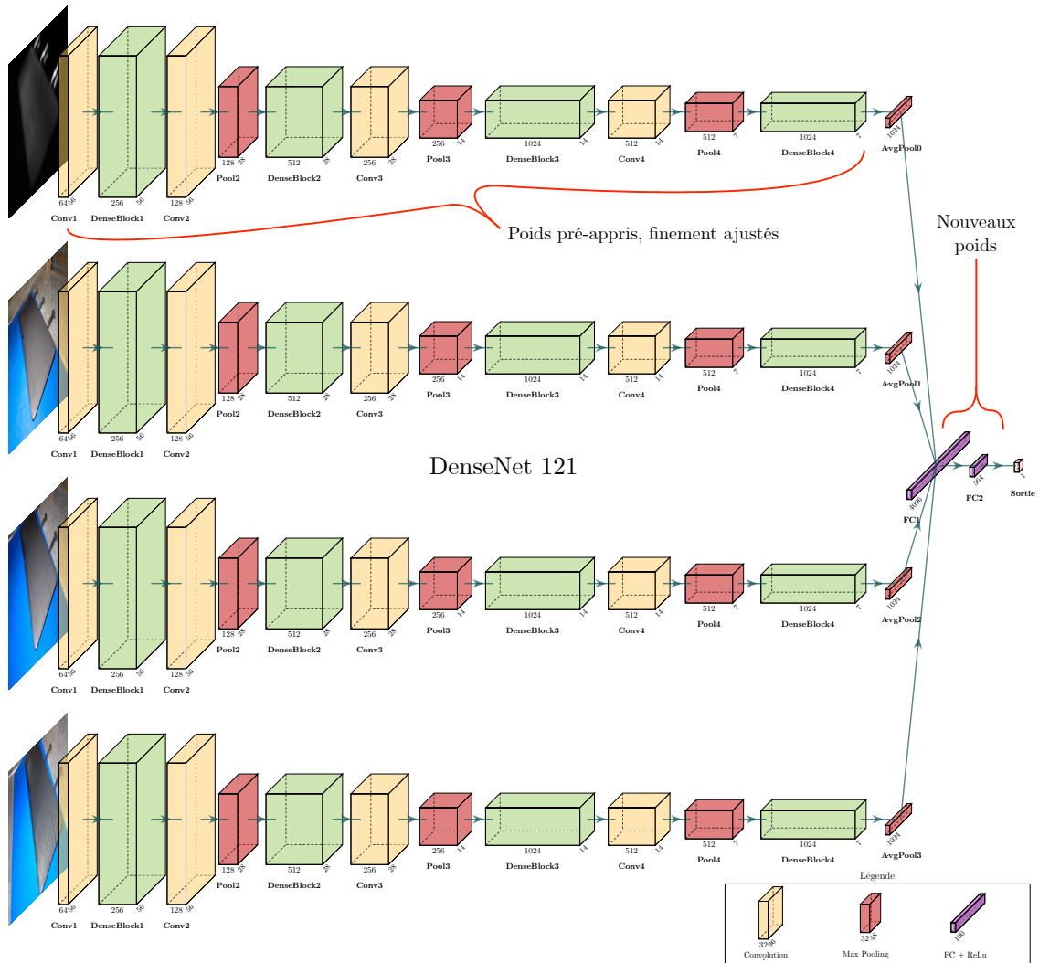
Figure 4.5 – Apprentissage par transfert de domaine à partir du réseau DenseNet121 pré-entraîné sur ImageNet.
