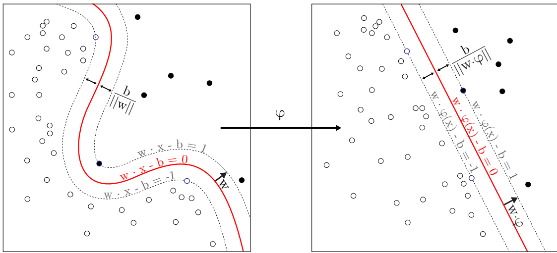
Figure E.3 – SVM avec kernel trick \varphi .
