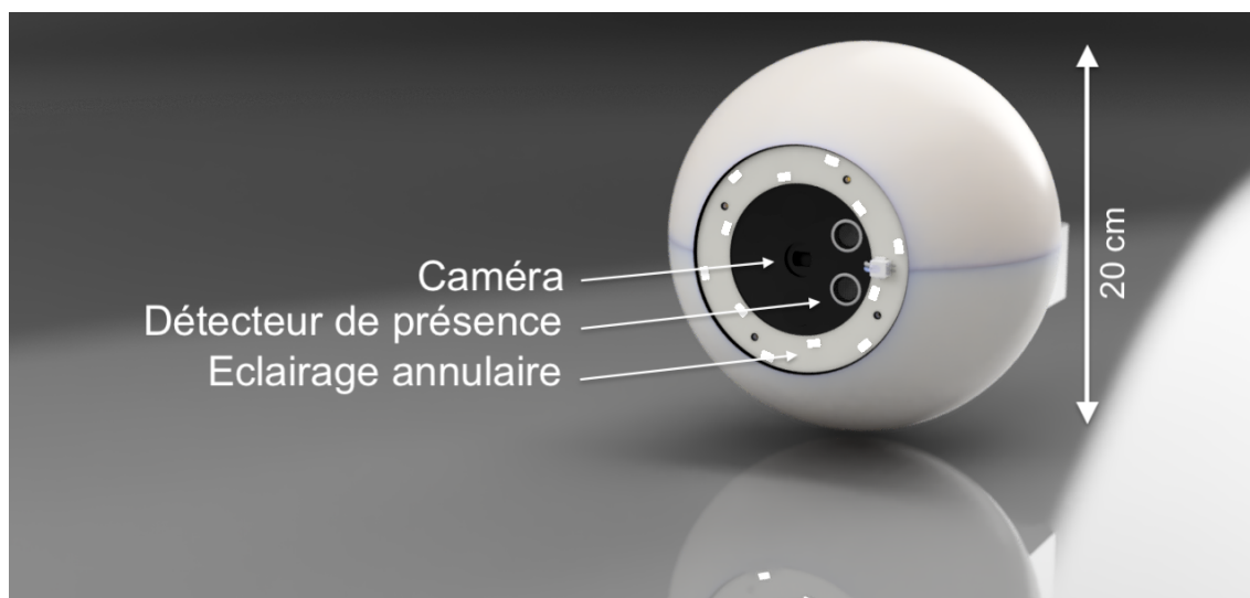
Figure 4.1 – Rendu réaliste du dispositif de mesure proposé.
