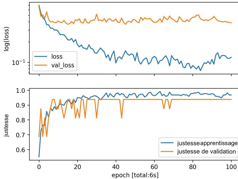
(a) Apprentissage initial des dernières couches du réseau.
