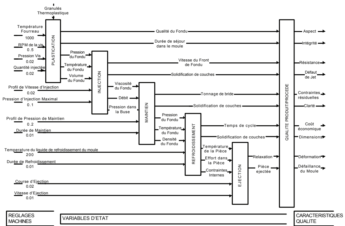
Figure 1.6 – Vue systémique du procédé d'injection-moulage, traduite de KAZMER et HATCH [KH99].
