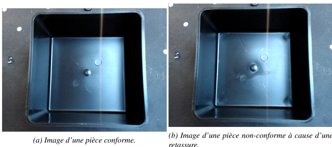
Figure 4.8 – Images originales pour la caméra linéairement polarisée selon un angle de 0^\circ .
