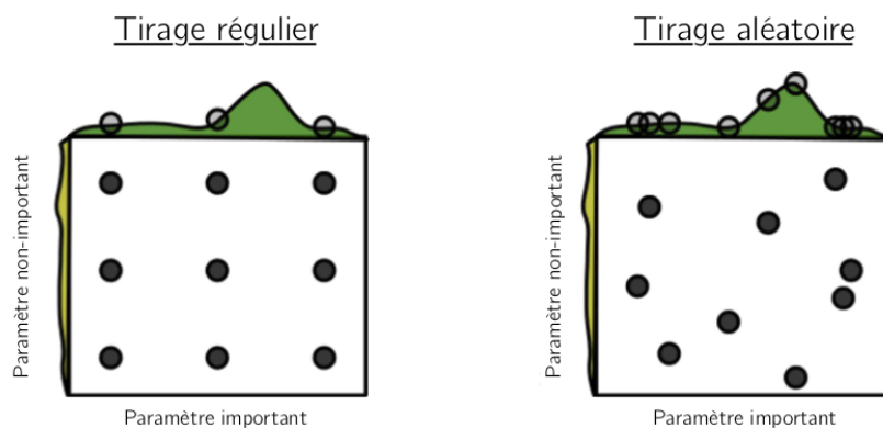
Figure 3.22 – Optimisation d'une fonction à deux variables avec neuf essais. Figure reproduite de [BB12].
