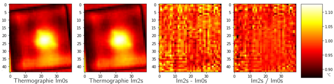
Figure 2.19 – Mesure par caméra thermique de l'évolution sur 2 secondes de la température d'une pièce.
