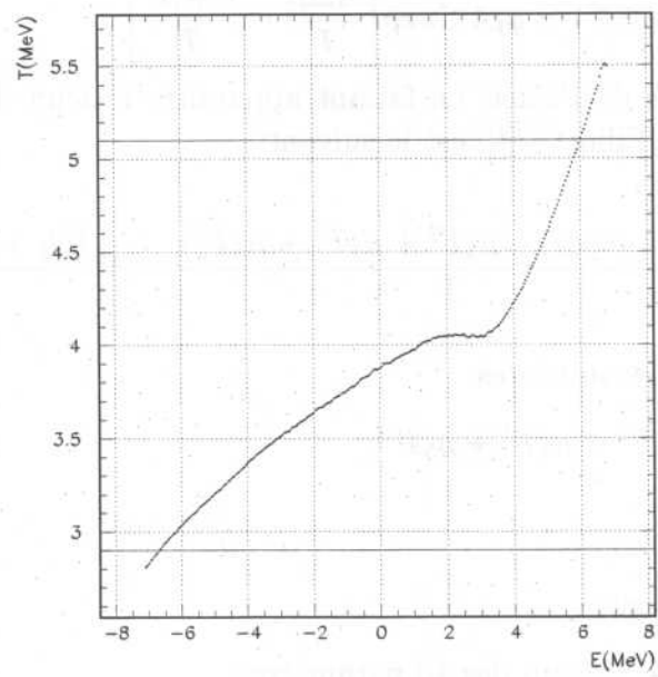
FIG. 22 - Courbe calorique à \lambda = \lambda_c constant
