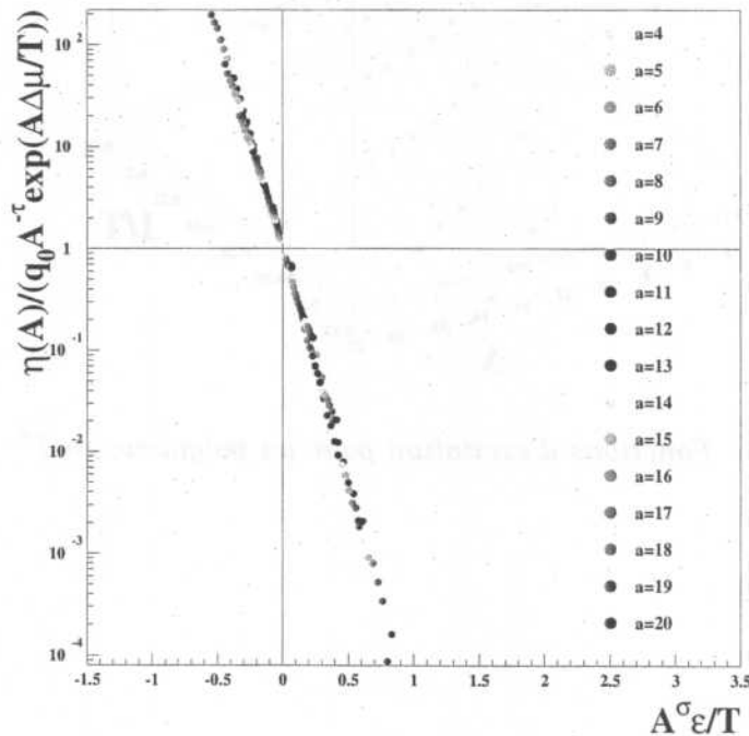
FIG. 34 – Fonction d'échelle pour un polynôme en T^6
