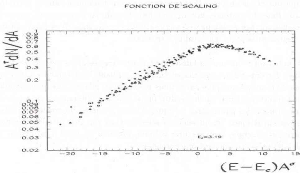
FIG. 20 – Fonction d'échelle, ensemble microcanonique à \langle V \rangle constant, masses 4 à 11
