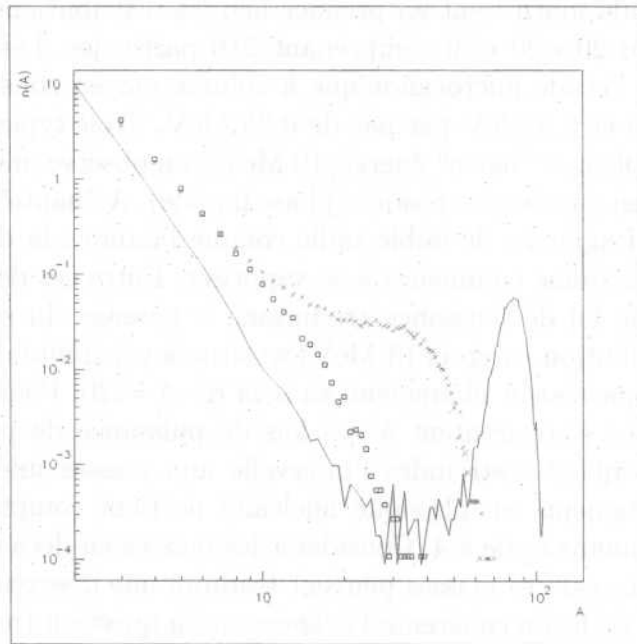
FIG. 7 – Distribution en masse des fragments
