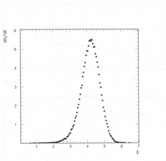
FIG. 5 - Distribution d'énergie pour T = 4.1 \text{ MeV} , pour les masses A = 1 .
