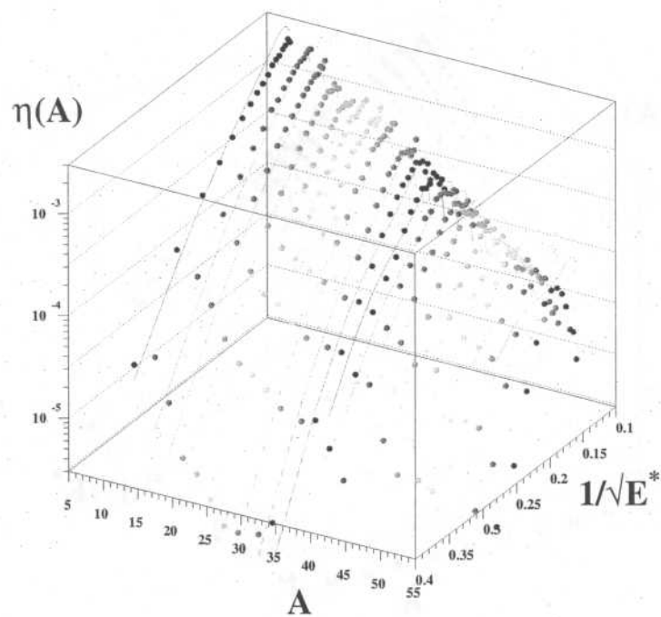
FIG. 49 – Fonctions d'excitation théoriques (lignes) et expérimentales (points) pour le système Au + Au à 60A.MeV
