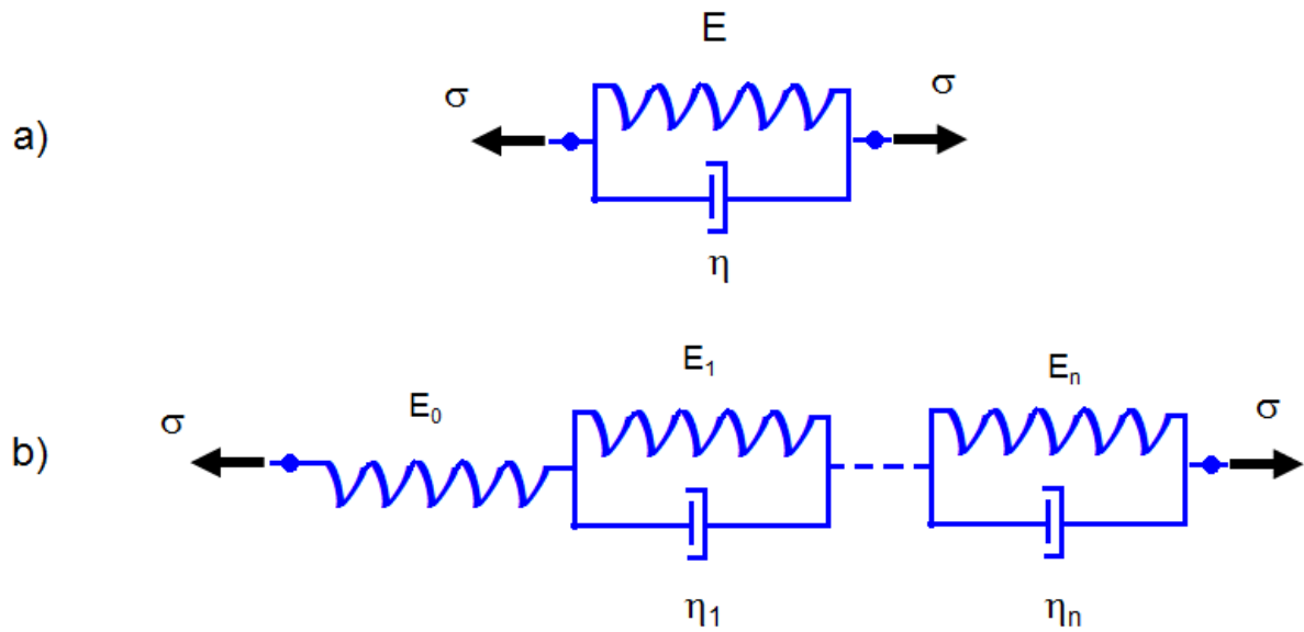
Figure III. 4 : a) Modèle de Kelvin-Voigt, b) Modèle de Kelvin-Voigt généralisé.
