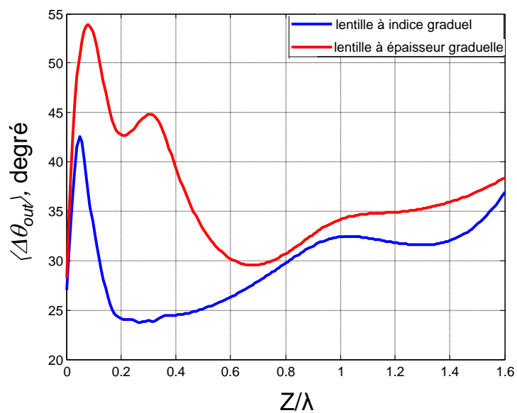
Fig. 3.14. Erreurs de compression \langle \Delta\theta_{out} \rangle des lentilles à indice graduel et à épaisseur graduelle sous éclairage positif \theta_{in} = 60^\circ en fonction de la distance normale normalisée.
