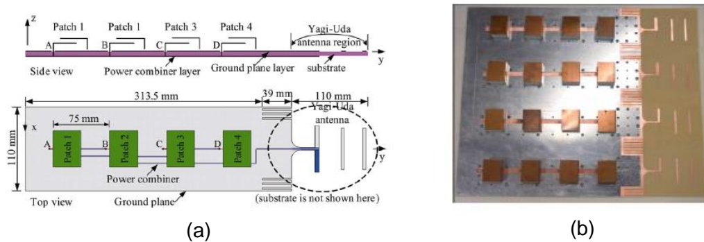
Fig. 4.8. Répéteur passif (a) configuration d'une unité, (b) photo du prototype fabriqué [IV.9].
