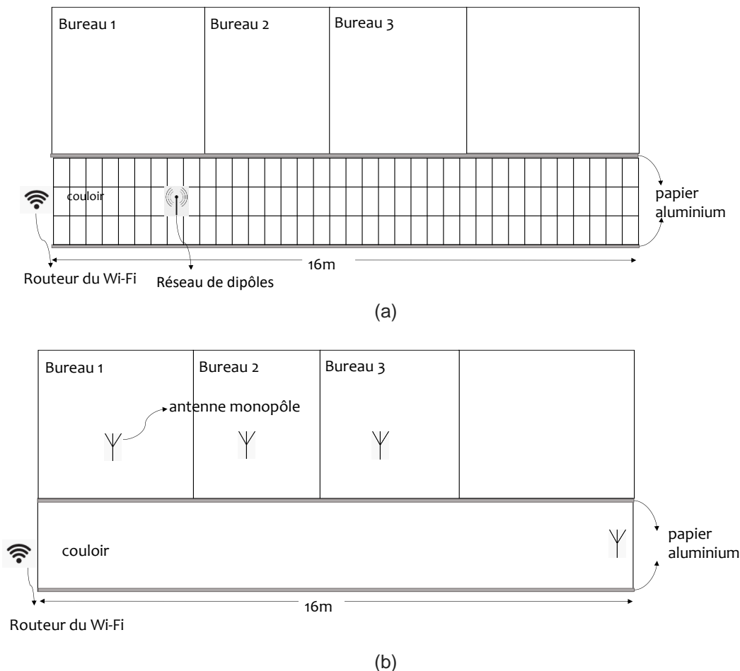
Fig. 4.22. Plan de mesure (a) maillage du couloir, (b) positionnement des points de mesure.
