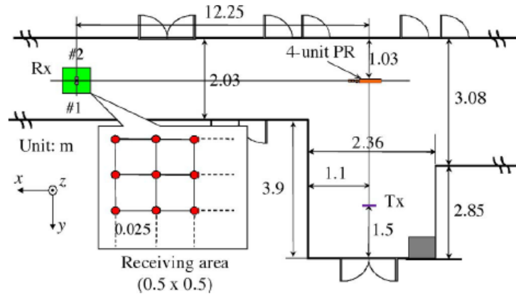
Fig. 4.9. Environnement de mesure [IV.9].
