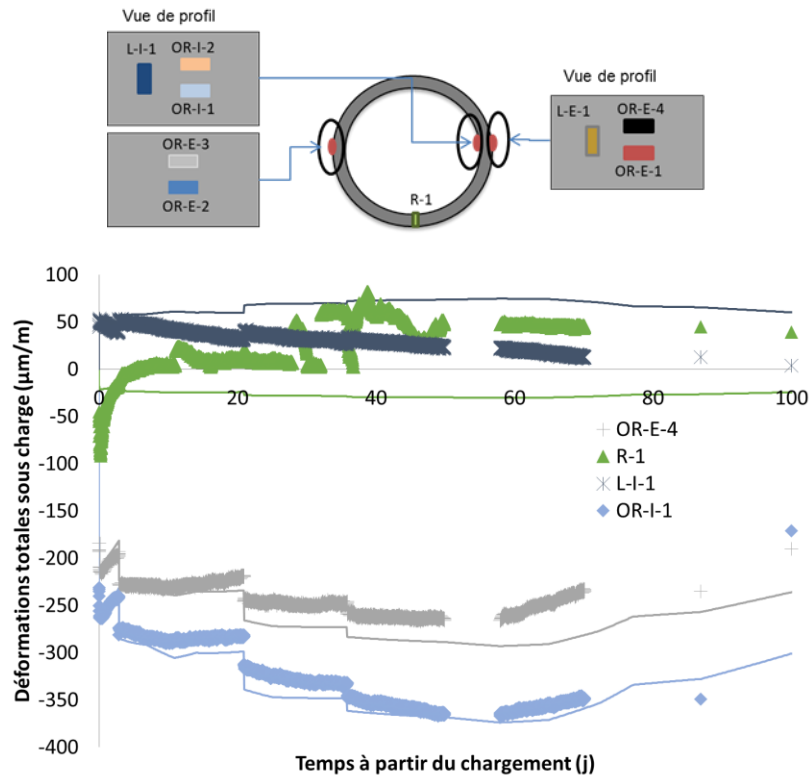
Figure IV-9 : résultats expérimentaux sous charge de l'anneau 2 dans la direction radiale (R-1), orthoradiales intrados (OR-I-1 et OR-E-1) et suivant la hauteur en intrados (L-I-1), avec modélisation à partir de la date de chargement et rappel du positionnement des jauges
