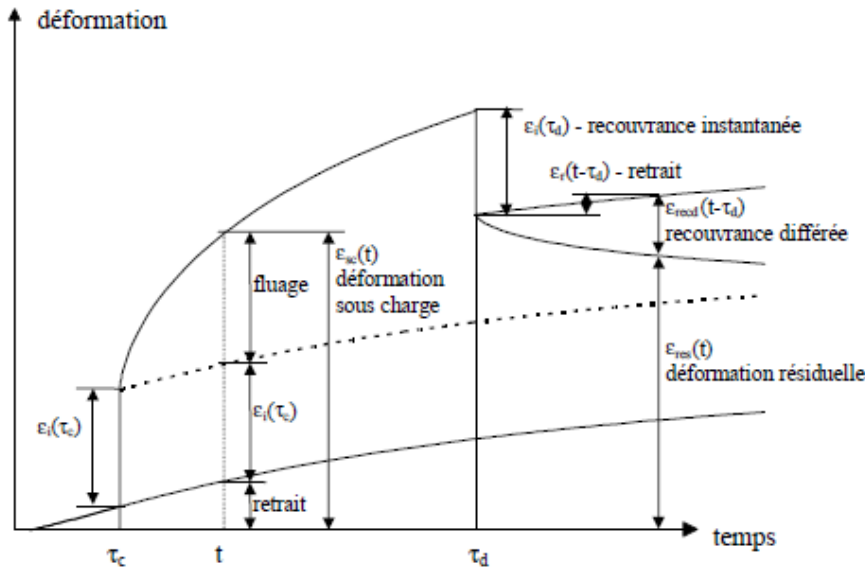
Figure I-18 : décomposition conventionnelle des déformations différées avec \epsilon_i la déformation instantanée au temps de chargement \tau_c , \tau_d la date de décharge, \epsilon_{sc} la déformation sous charge, \epsilon_r la déformation de retrait, \epsilon_{recd} la déformation de recouvrance et \epsilon_{res} la déformation résiduelle
