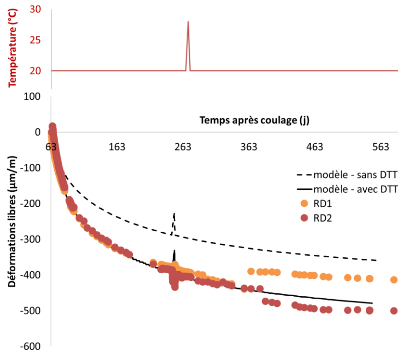
Figure IV-11 : évolutions expérimentales du retrait en dessiccation de deux éprouvettes cylindriques 11 x 22 cm 3 (RD1 et RD2) à 20 °C et 50% HR, et modélisations avec ou sans prise en compte des paramètres de DTT à partir de la date de séchage
