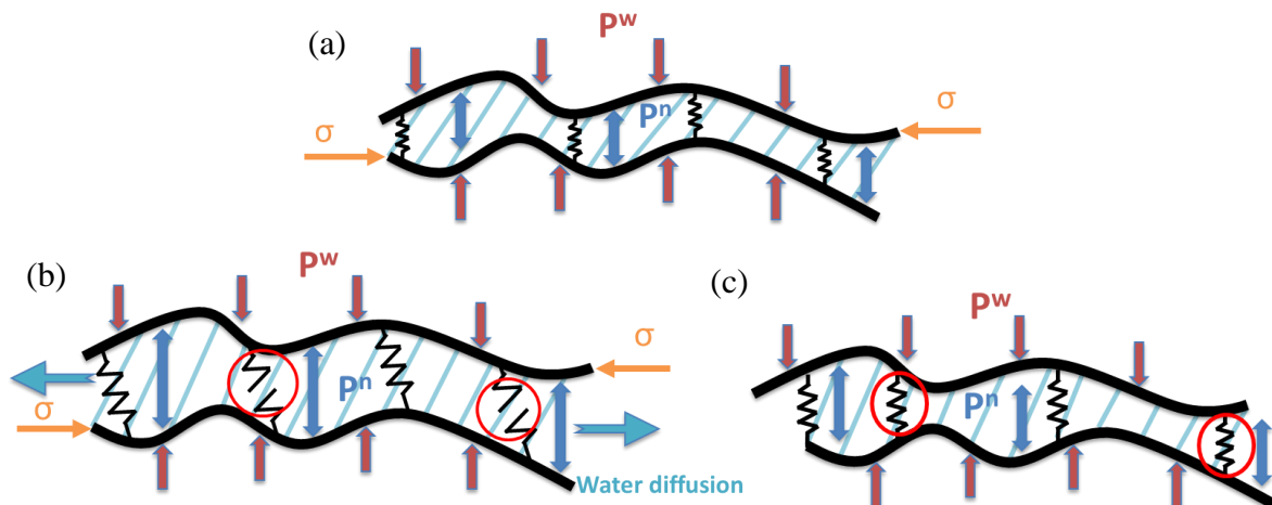
Figure II-1 : schéma de configuration des C-S-H sous charge ; (a) état stable de référence avant chauffage, (b) état lors d'une élévation thermique rapide, les feuillet s'éloignent, ce qui facilite le cisaillement, (c) retour à un état stable après évacuation d'une quantité d'eau de l'inter-feuillet nécessaire pour rééquilibrer les pressions
