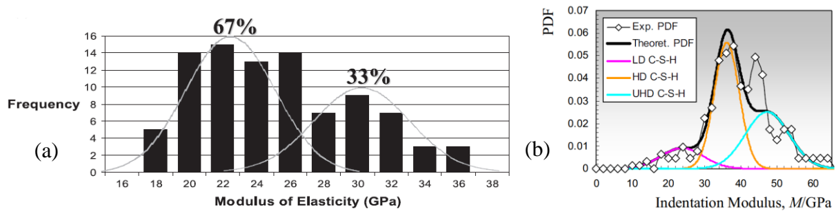
Figure I-2 : fréquence du module d'élasticité des C-S-H issus de la nanoindentation [Constantinides et Ulm, 2004] (a) et probabilité de densité du module d'indentation (Probability density plots = PDF) [Vandamme et Ulm, 2009] (b)
