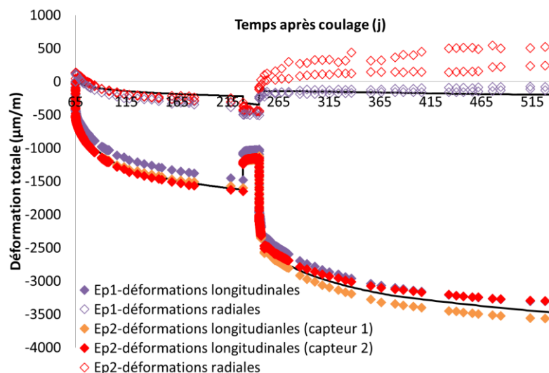
Figure IV-14 : déformations longitudinales et radiales (2 jauges par éprouvettes) totales en dessiccation de deux éprouvettes cylindrique 11 \times 22 \text{ cm}^3 (Ep1 avec 1 capteur interne et Ep2 avec 2 capteurs externes) sous charge variable de 30%-60% f_{cm} à 20 °C et 50% HR, et modélisation finale à partir de la date de chargement
