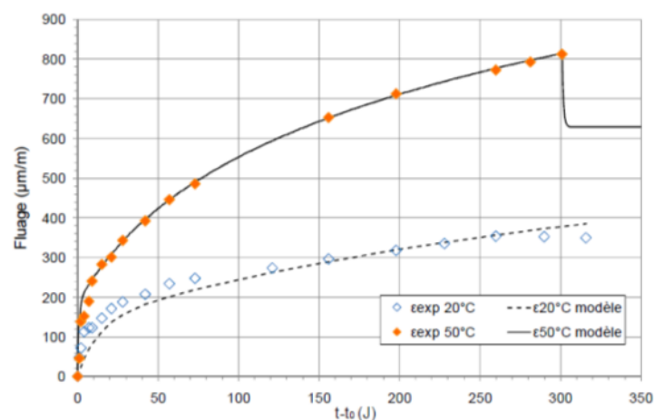
Figure I-26 : évolution du fluage propre d'un CEM I chargé à 30% f_{cm} à deux températures 20 °C et 50 °C [Ladaoui, 2010]
