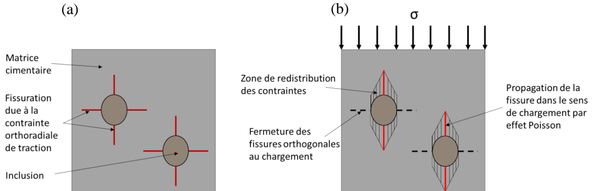
Figure IV-2 : schéma de fissuration autour des inclusions causée par le retrait de dessiccation due à la traction orthoradiale (a), schéma de concentration des contraintes sous charge extérieure due à la fissuration du matériau, avec les fissures dans la direction chargée (en rouge) qui s'ouvrent, tandis que celles perpendiculaires (en pointillé) ne peuvent pas se créer ou se refermer (b)
