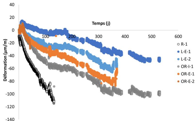
Figure III-20 : déformations totales des essais sur anneaux en endogène à 20°C depuis leur démoulage
