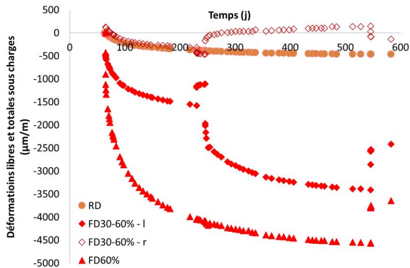
Figure III-17 : déformations libres et totales sous charge des essais en dessiccation sur éprouvette cylindrique 11 x 22 \text{cm}^3
