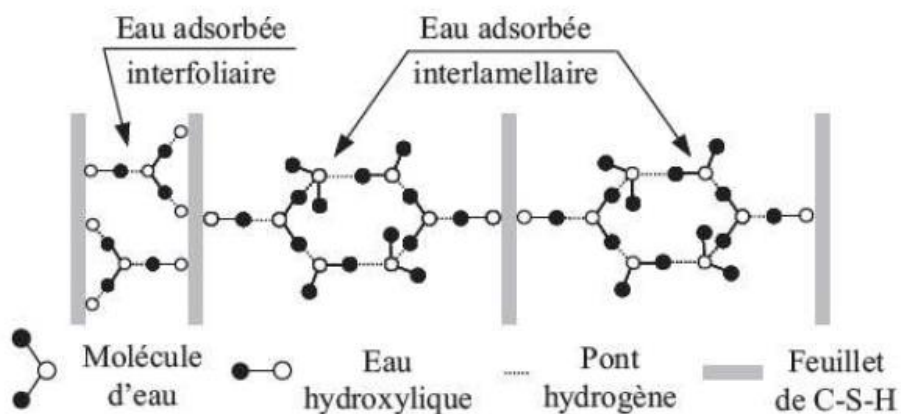
Figure I-7 : état de l'eau dans le gel de C-S-H [Sierra, 1974]
