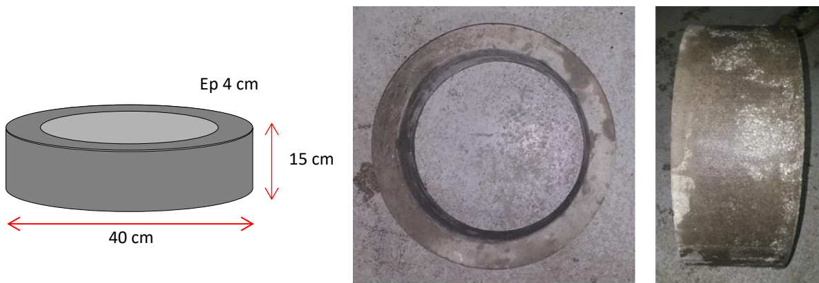
Figure III-4 : géométries et photos des anneaux de béton au démoulage
