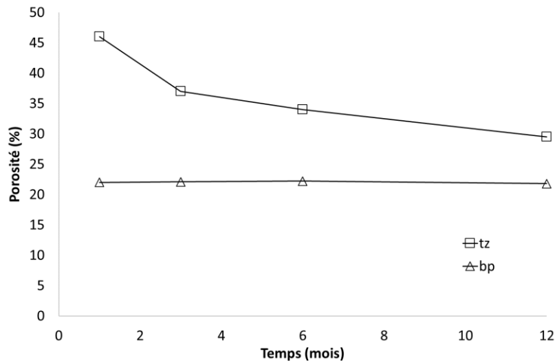
Figure I-16 : évolution de la porosité de l'ITZ (courbe tz) et de la pâte de ciment (courbe bp) d'un mortier au cours du temps [Bourdette et al., 1995]
