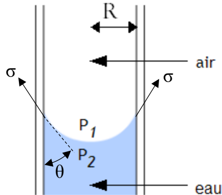
Figure I-5 : représentation schématique de la tension capillaire dans un tube
