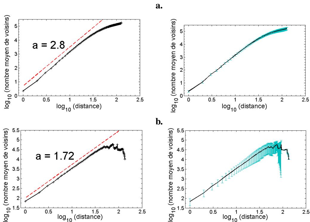
FIGURE 5.17 – La méthode statistique basée sur l’intégrale de corrélation pour les images des quarante-cinq scènes forestières de notre ensemble. a. Les attributs statistiques correspondant aux images couleur. b. Les attributs statistiques correspondant aux images de profondeur. Dans les deux cas, le tracé de gauche retranscrit l’évolution de l’intégrale de corrélation C(r) ainsi que l’exposant de la loi de puissance suivie. Le tracé de droite correspond à la même évolution associée aux barres d’erreur à plus ou moins l’écart-type obtenu sur les quarante-cinq scènes naturelles.
