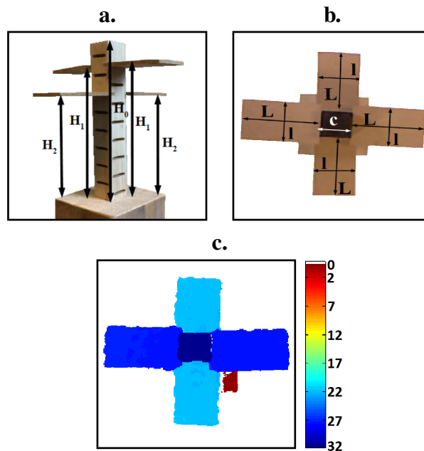
FIGURE 4.3 – Un objet de calibration de Volume Efficace connu. a. Une image couleur latérale ( H_0 = 31 \text{ cm} , H_1 = 27 \text{ cm} et H_2 = 21.5 \text{ cm} ). b. Une image couleur de dessus ( L = 10 \text{ cm} , l = 6 \text{ cm} et c = 4 \text{ cm} ). c. Une image de profondeur de dessus. La colorbar donne la différence entre la valeur de profondeur maximum et la profondeur locale Z_i (les valeurs sont données en cm). Valeur théorique : H_0 \times c \times c + 2 \times L \times l \times (H_1 + H_2) - 4 \times H_2 \times 1 \times 1 = 6230 \text{ cm}^3 .
