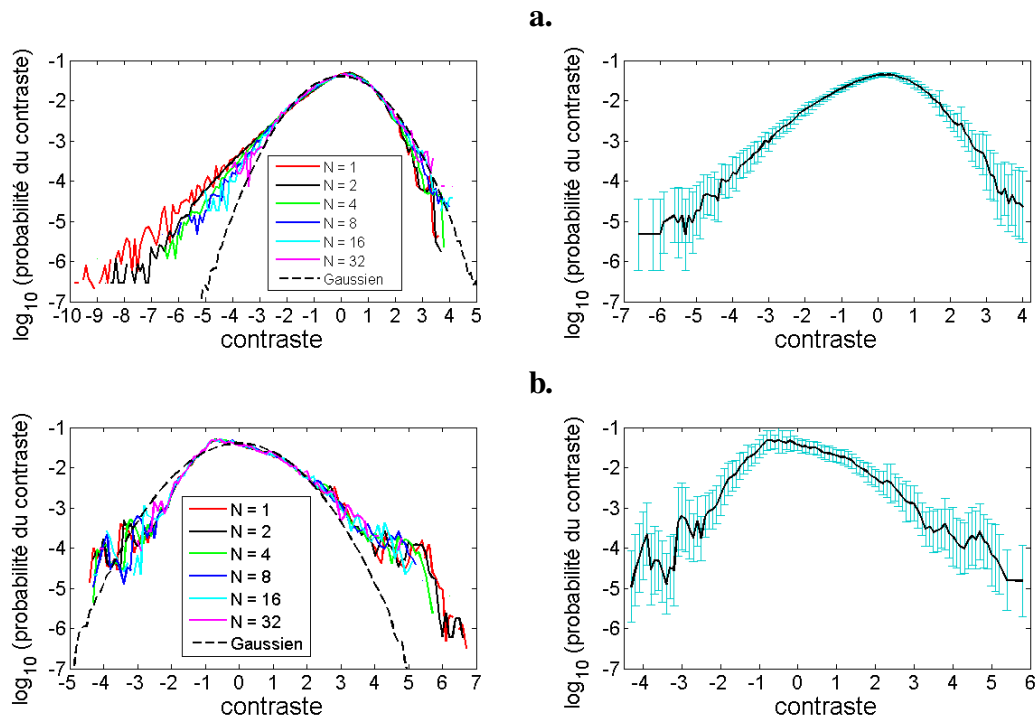
FIGURE 5.12 – La méthode statistique basée sur la distribution du contraste pour les images des quarante-cinq scènes forestières de notre ensemble. a. Les attributs statistiques correspondant aux images d’intensité. b. Les attributs statistiques correspondant aux images de profondeur. Dans les deux cas, le tracé de gauche retranscrit l’évolution de la distribution du contraste P_N(I_N(x, y)) pour chaque échelle N simulée. Le tracé de droite correspond à la distribution du contraste P_8(I_8(x, y)) associée aux barres d’erreur à plus ou moins l’écart-type obtenu sur les quarante-cinq scènes.
