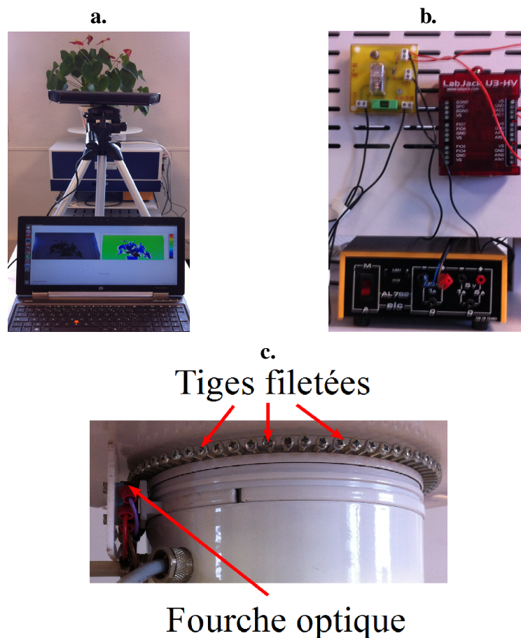
FIGURE 4.10 – L'imageur de profondeur motorisé. a. Une vue globale. b. Son système LabJack pour déclencher la rotation. c. Sa fourche optique et ses tiges filetées pour arrêter la rotation.
