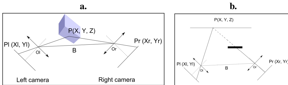
FIGURE 2.3 – Les méthodes de stéréo-vision. a. Un schéma de principe de la méthode de stéréo-vision à deux systèmes de vision. b. Illustration de la présence d'occlusions.
