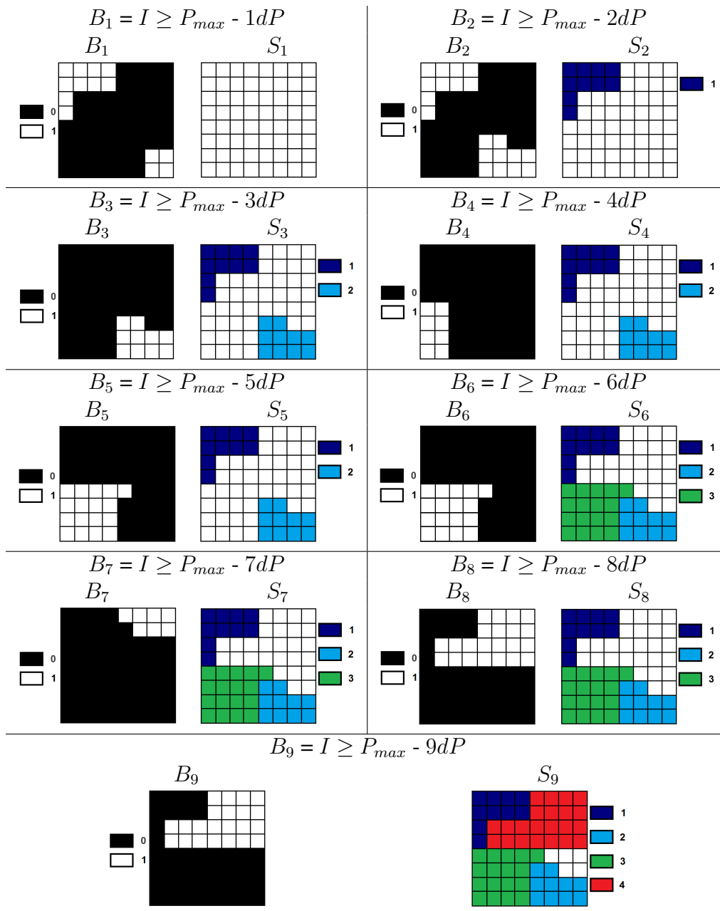
FIGURE 3.4 – Le déroulement de notre méthode de segmentation lorsqu'elle est appliquée à l'image I de la Fig. 3.2. Dans chaque case du tableau, l'image B_s correspond à l'image binaire analysée à l'étape s et S_s à l'image segmentée correspondante.
