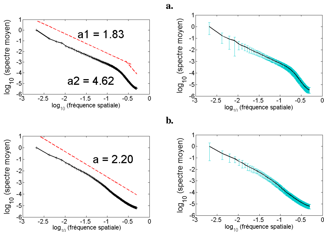
FIGURE 5.14 – La méthode statistique basée sur le spectre de puissance moyen pour les images des quarante-cinq scènes forestières de notre ensemble. a. Les attributs statistiques correspondant aux images d'intensité. b. Les attributs statistiques correspondant aux images de profondeur. Dans les deux cas, le tracé de gauche retranscrit l'évolution du spectre de puissance moyen \overline{P}(\rho) ainsi que les différentes lois de puissance suivies. Le tracé de droite correspond à la même évolution associée aux barres d'erreur à plus ou moins l'écart-type obtenu sur les quarante-cinq scènes.
