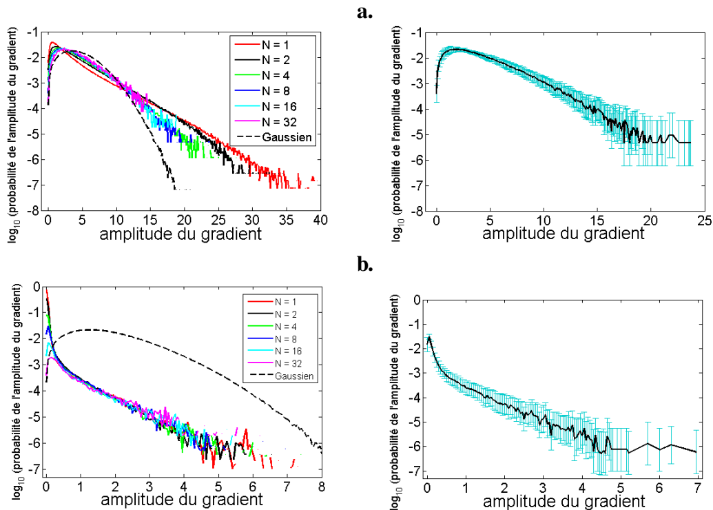
FIGURE 5.13 – La méthode statistique basée sur la distribution du gradient pour les images des quarante-cinq scènes forestières de notre ensemble. a. Les attributs statistiques correspondant aux images d'intensité. b. Les attributs statistiques correspondant aux images de profondeur. Dans les deux cas, le tracé de gauche retranscrit l'évolution de la distribution du gradient P_N(|\nabla I_N(x, y)|) pour chaque échelle N simulée. Le tracé de droite correspond à la distribution du gradient P_8(|\nabla I_8(x, y)|) associée aux barres d'erreur à plus ou moins l'écart-type obtenu sur les quarante-cinq scènes.
