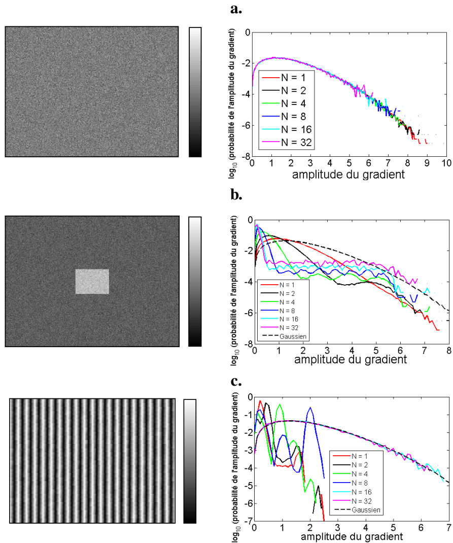
FIGURE 5.4 – Trois images synthétiques de référence et leurs histogrammes P_N(|\nabla I_N(x, y)|) de la distribution du gradient. Les trois images sont identiques à celles de la Fig. 5.3.
