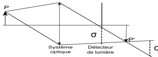
FIGURE 2.4 – La focalisation à travers un système de vision composé d'une optique et d'un détecteur de lumière. Le point P' n'est pas focalisé.
