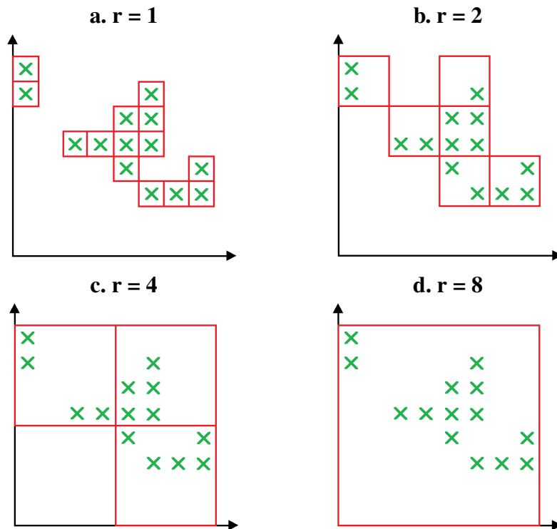
FIGURE 5.6 – Le recouvrement d'un nuage de points bidimensionnel de 14 points par N(r) carrés de côté r . a. Pour r = 1 , Il faut 14 carrés pour entièrement recouvrir le nuage de points. b. Pour r = 2 , Il en faut 6. c. Pour r = 4 , Il en faut 3. d. Pour r = 8 , Il en faut 1.
